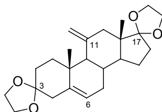
11-Méthylidène-3,3,17,17-(éthylènedioxy)androst-5-ène
