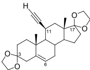
11 \beta -(S)-Éthynyl-3,3,17,17-(éthylènedioxy)-androst-5-ène
