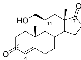
11β-(S)-Hydroxyméthylandroster-5-èn-3,17-dione
