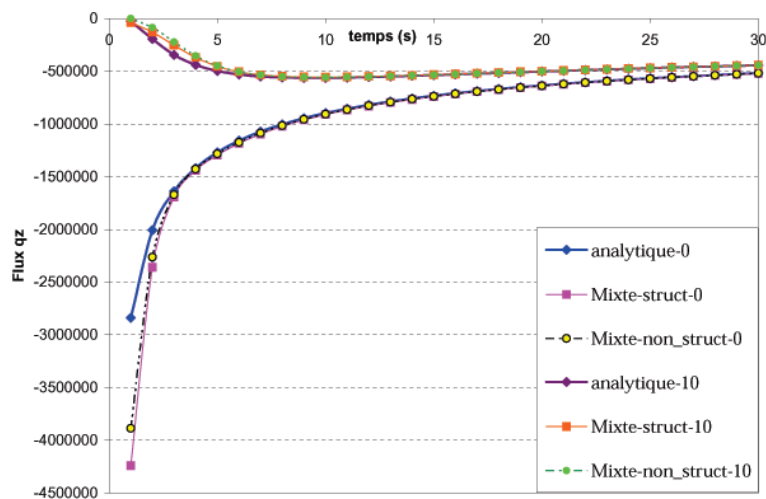
FIG. 3.20 – Influence du mode de triangulation sur l'évolution du flux q_z avec h = 2,5mm .
