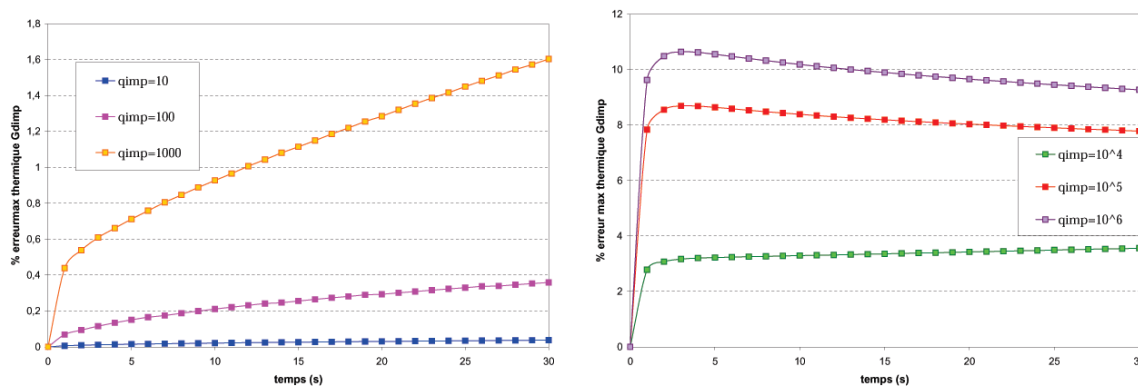
FIG. 2.54 – Influence de la valeur de \Phi_{imp} sur la solution numérique Gdimp : évolution de la température pour un noeud placé directement sur la face imposée ( z = 0\text{mm} ) avec h = 2\text{mm} .
