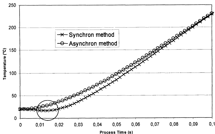
FIG. 1.7 – Comparaison entre la thermique synchrone et asynchrone [D'Alvise 2002].
