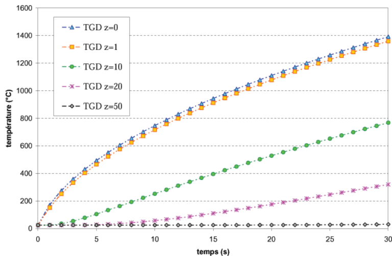
FIG. 2.25 – Evolution de la thermique TGD pour les 5 traceurs avec h = 2,3\text{ mm} et dt = 1\text{ s} .
