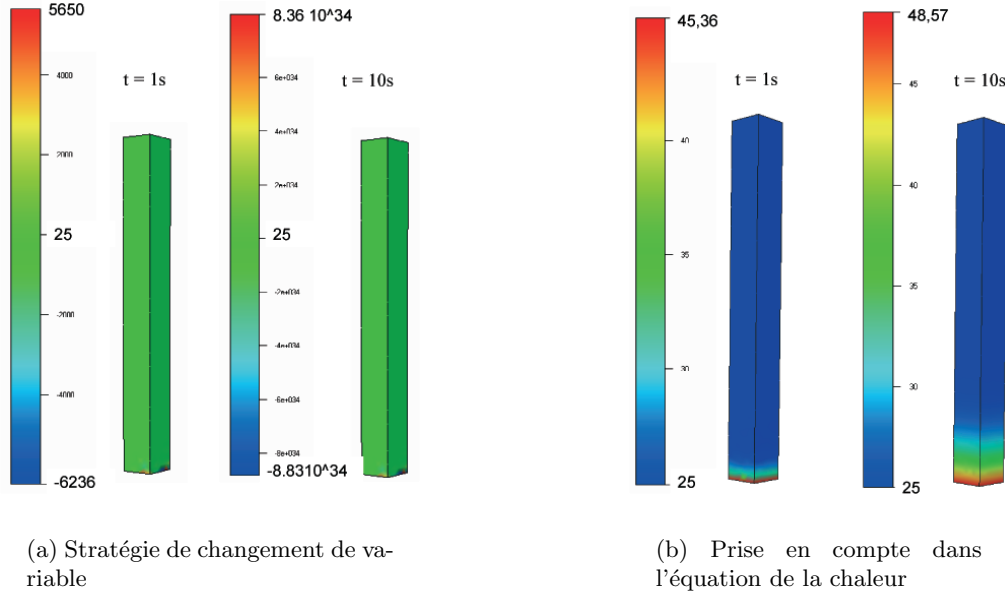
FIG. 3.4 – Test de conduction imposée : T_0 = 25^\circ\text{C} , T_{out} = 50^\circ\text{C} et h_{cd} = 20\,000\text{ W/m}^\circ\text{K} .
