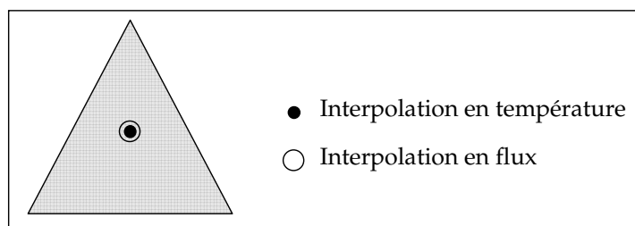
FIG. 2.1 – Configuration 2D de l'élément fini mixte P_0/P_0 en température/flux.
