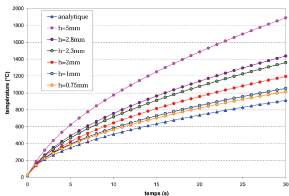
(a) évolution thermique du second traceur situé à 1 mm du bord
