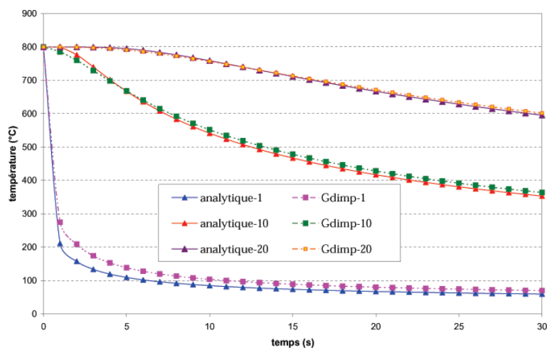
FIG. 2.43 – Evolution de la température des 3 traceurs : comparaison entre la solution analytique et la version Gdimp de Forge3 ® : h = 2,8\text{ mm} et dt = 1\text{ s} .
