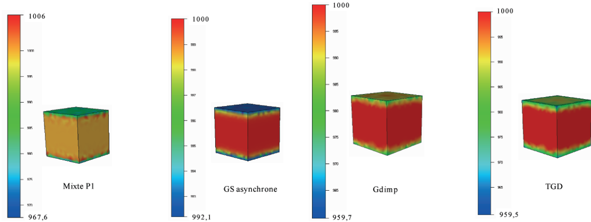
FIG. 4.10 – Isovaleurs de la température avec les quatre modèles de résolution thermique à l'instant dt = 0,01s et h = 1mm .
