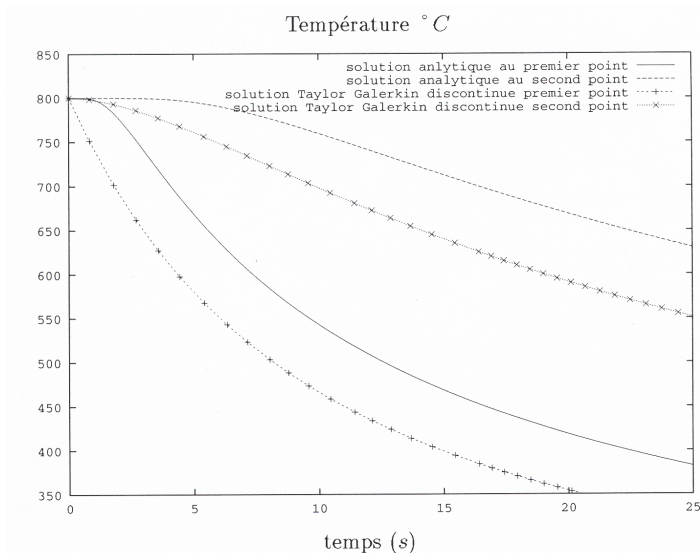
FIG. 2.8 – Absorption du choc thermique avec la version TGD "TTT" de [Aliaga 2000].
