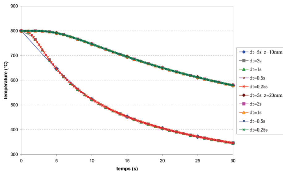
FIG. 2.17 – Evolution thermique en fonction du pas de temps dt à maillage fixé ( h = 2\text{mm} ).
