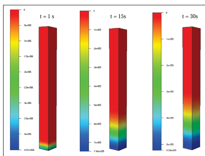
FIG. 3.15 – Isovaleurs de la composante suivant z du flux de chaleur lors de la résolution Mixte continue: mise en évidence du phénomène de diffusion thermique.
