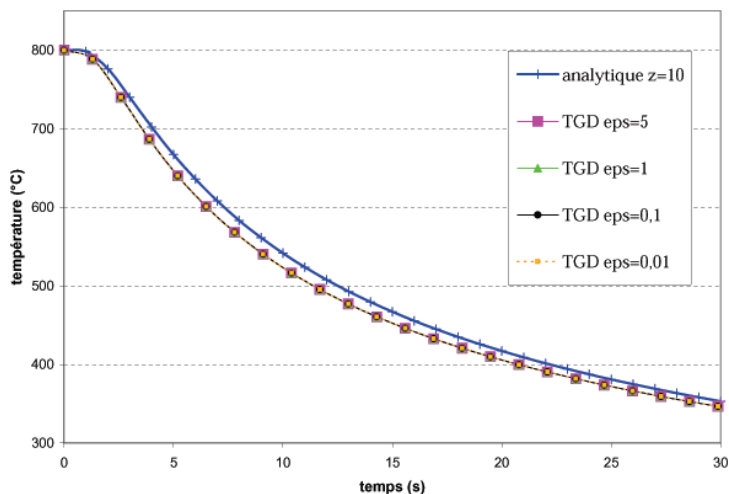
FIG. 2.20 – Sensibilité du schéma TGD en fonction de l'erreur \varepsilon : évolution de la température pour z = 10\text{mm} et h = 2\text{mm} .
