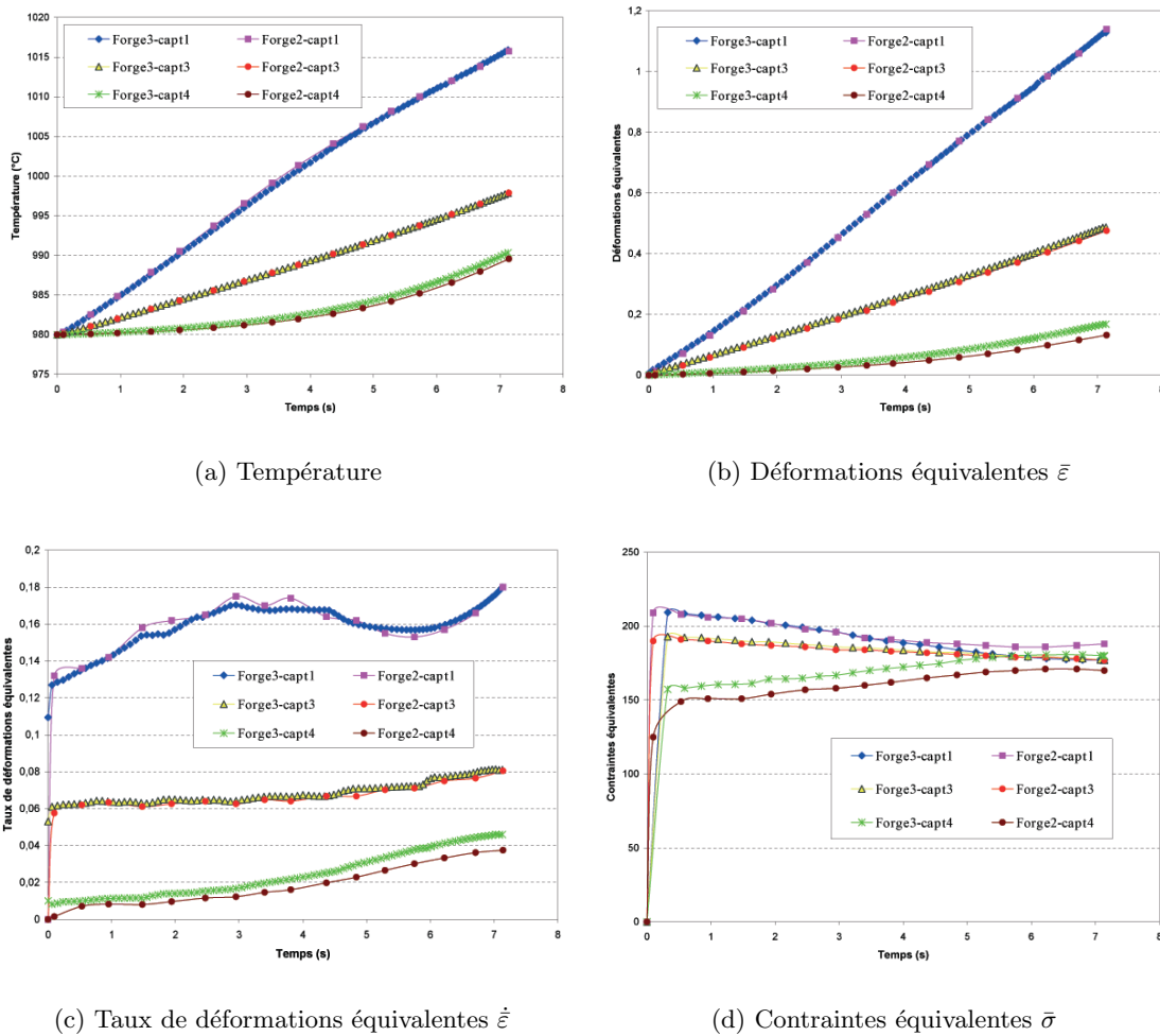
FIG. 4.18 – Cas anisotherme: résultats Cemef pour la résolution thermomécanique de Forge2 ® et de Forge3 ® .
