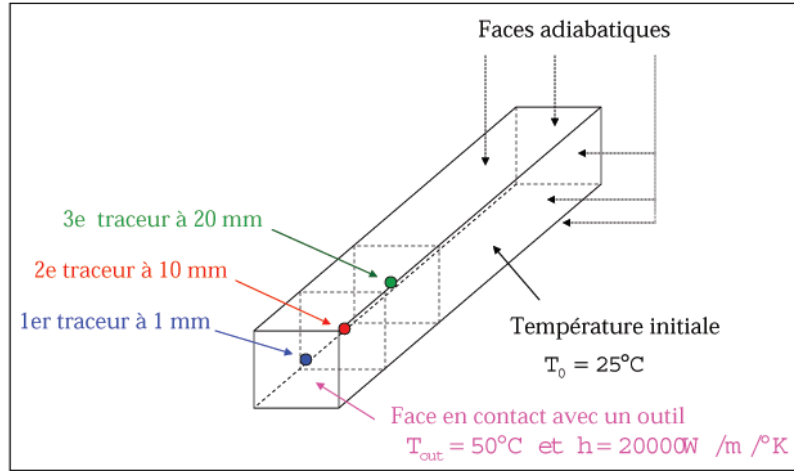
FIG. 3.42 – Barre d'acier à 25^\circ\text{C} maintenue à \Phi_{cond} sur l'une de ces faces.
