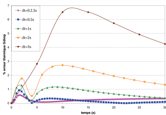
(d) Evolution de l'erreur thermique z = 10mm
