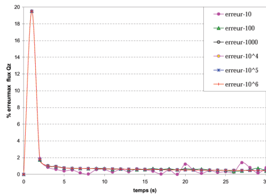
(c) Erreur q_z
