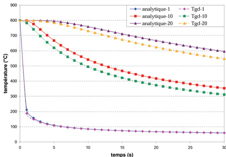
FIG. 2.11 – Evolution de la température TGD avec un maillage grossier h = 5\text{mm} .
