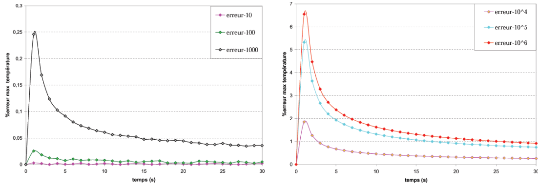
(a) Erreur thermique
