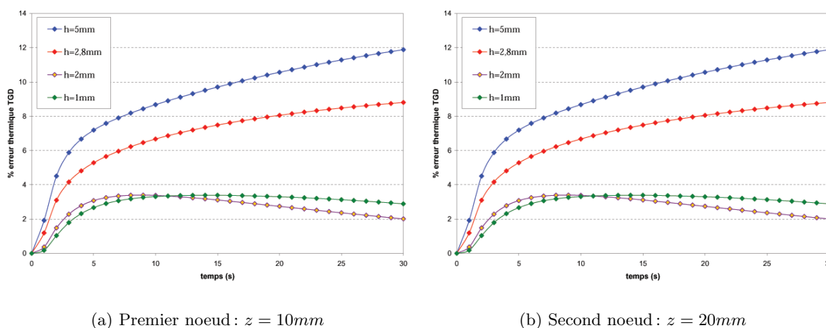
FIG. 2.16 – Etude de l'erreur de la solution numérique TGD en fonction du maillage.
