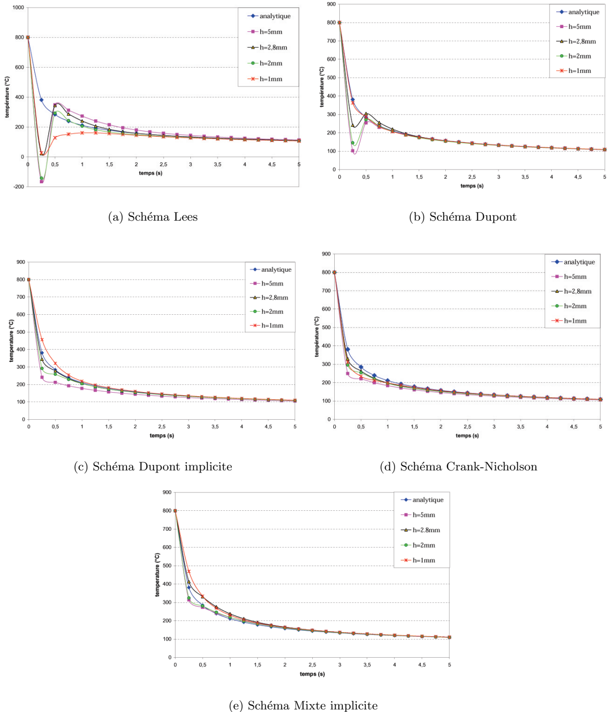
FIG. 3.8 – Evolution de la température pour les 5 schémas d'intégration en fonction du maillage avec un capteur en peau à z = 1\text{mm} .
