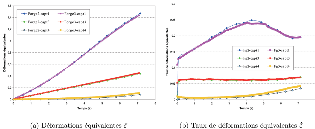
FIG. 4.16 – Résultats Cemel pour la résolution mécanique de Forge 2 ® et de Forge 3 ® .
