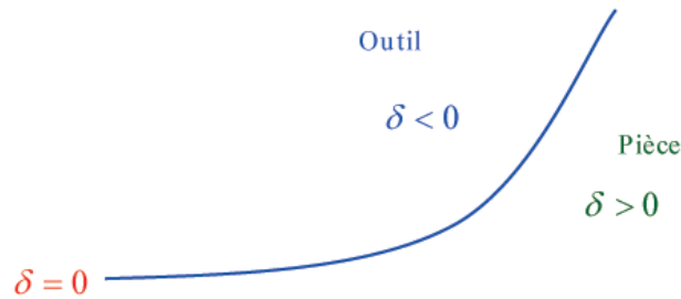
FIG. 4.3 – Distance de pénétration.
