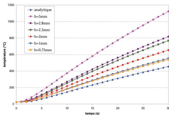
(b) évolution thermique du troisième traceur situé à 10 mm du bord
