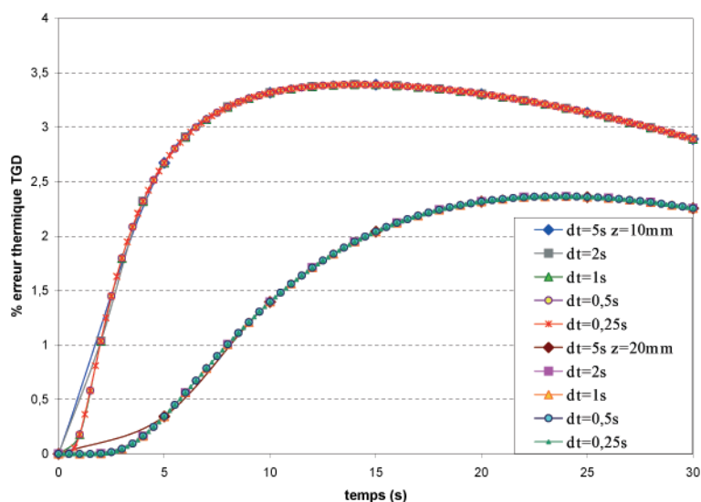
FIG. 2.18 – Evolution de l'erreur TGD des deux traceurs en fonction de dt avec h = 2\text{mm} .
