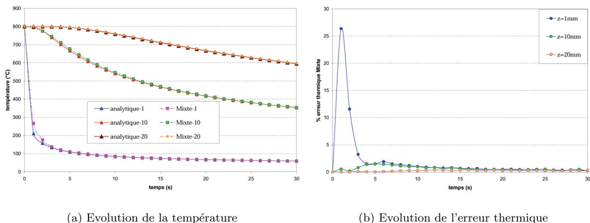
FIG. 3.16 – Comparaison entre la formulation Mixte continue et la solution analytique.
