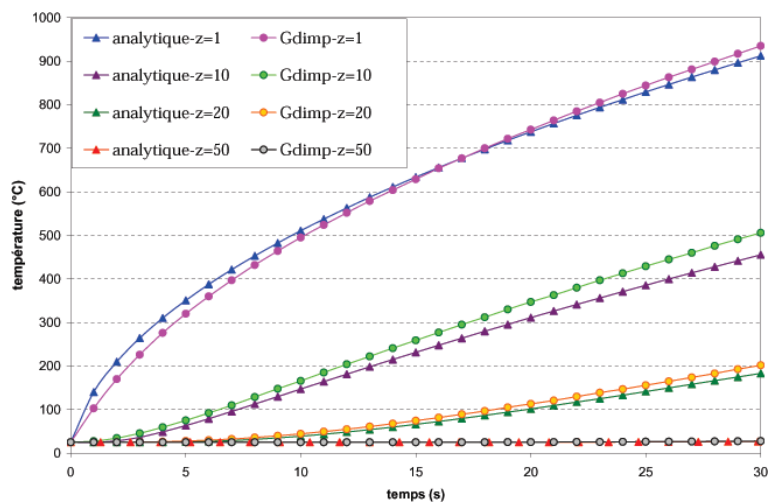
FIG. 2.51 – Evolution de la température des 2 traceurs : comparaison entre la solution analytique et la version Gdimp de Forge3 ® .
