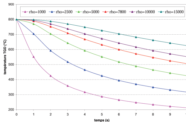
(d) courbes TGD : influence de la densité \rho
