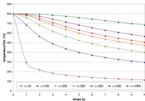
(f) courbes TGD : influence de la capacité c
