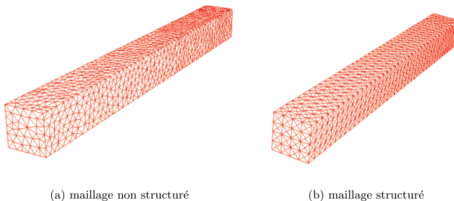
FIG. 2.12 – Taille de maille h = 2,5\text{mm} .
