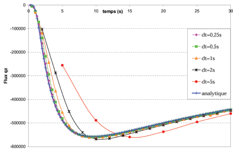
FIG. 3.27 – Influence du pas de temps dt sur l'évolution du flux q_z avec z = 10mm .
