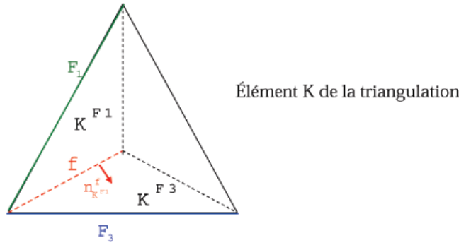
FIG. 2.39 – Calcul du saut à l'interface de deux sous-éléments K^{F1} et K^{F3} .
