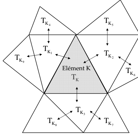
FIG. 2.3 – Schéma P_0/P_0 : contribution de 2 couches d’éléments au voisinage de l’élément K .
