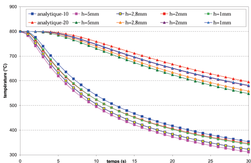
FIG. 2.15 – Evolution thermique TGD des deux traceurs en fonction du raffinement du maillage à pas de temps fixé ( dt = 1 \text{ s} ).
