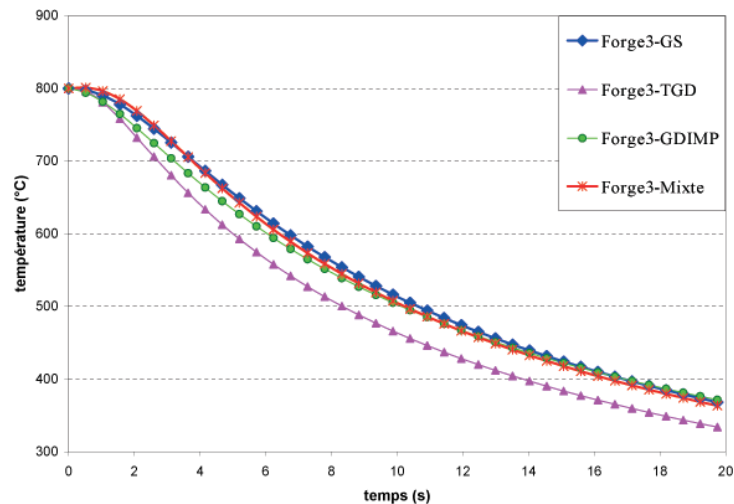
FIG. 3.54 – Comparaison des divers modèles numériques sur le test de refroidissement.
