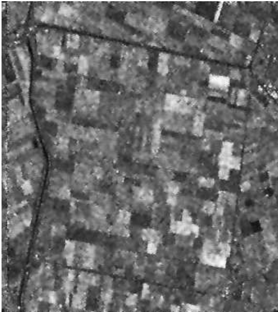
Fig. 2.13 – Résultat de la restauration par le filtrage de Lee de l'image radar présenté en figure 2.10.
