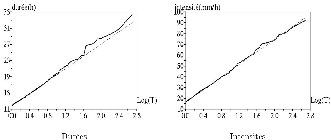
FIG. 8.8 – Distribution des durées et intensités des événements pluvieux générés à l'aide du modèle stochastique de pluie (trait continu), et comparaison avec la distribution exponentielle ( \text{Gradex } 3.3 \ln(10) = 7.6 heures pour les durées et \text{Gradex } 12.5 \log(10) = 28.8 \text{ mm/h} pour les intensités moyennes). Deux événements pluvieux sont séparés par 24 heures de temps sec.
