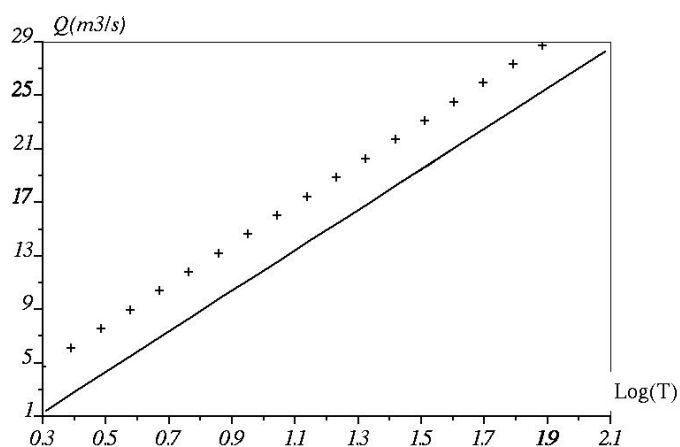
FIG. 7.5 – Distributions théoriques des débits de pointes de crues d'un bassin fictif de 100 \text{ km}^2 d'après le modèle d'Hebson & Wood : a) F(Q_{max}) = 1 - \exp(-\beta Q_{max}/KA_r) distribution des intensités moyennes de pluie efficace (croix), b) distribution issue du modèle d'Hebson & Wood (trait continu).
