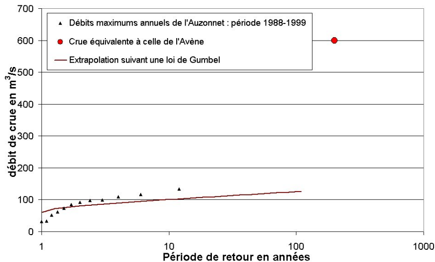
FIG. 1.1 – Distribution statistique des débits de pointes de crues d'un bassin versant de 50 km^2 situé dans le Gard (Auzonnet), ajustement d'une distribution de Gumbel, et débit de la crue de 1997 de l'Avène (bassin versant voisin).
