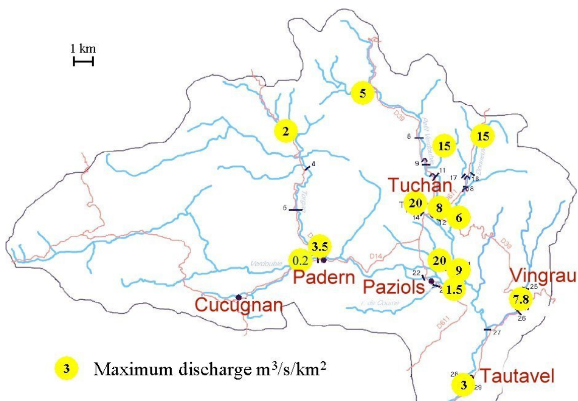
FIG. 4.17 – Répartition des débits de pointe de crue estimés dans le bassin versant du Verdoble
