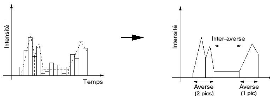
FIG. 8.2 – Représentation schématique d'un hyétogramme dans le modèle stochastique de pluie
