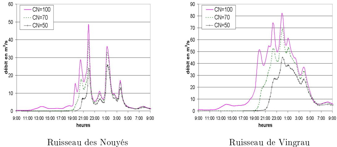
FIG. 4.20 – Résultats de simulations hydrologiques de la crue du Verdouble des 12 et 13/11/99.
