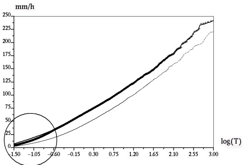
FIG. 8.16 – Distribution des intensités de pluies efficaces ( S = 10 mm) : a) intensités de pluies brutes en 5 minutes (trait continu), b) modèle SCS standard (pointillés), c) modèle SCS modifié (croix).
