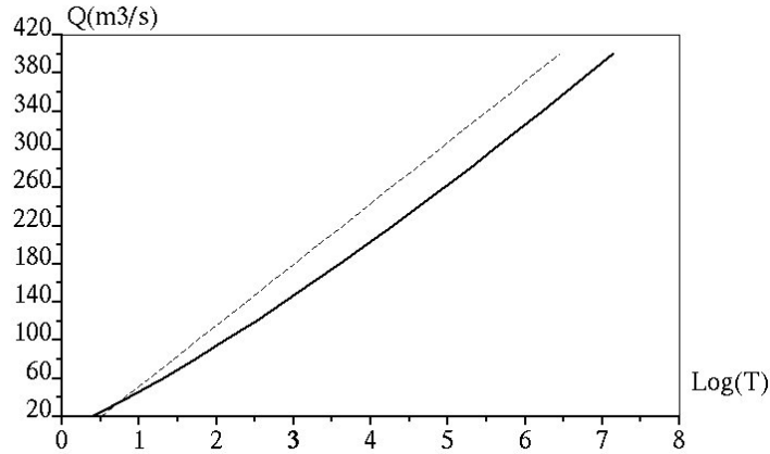
FIG. 7.8 – Distributions théoriques des débits de pointes de crues d'un bassin fictif de 100 km^2 d'après des données proposées dans la publication de Diaz-Granados et al. : a) Approximation de Diaz-Granados avec 1/\beta = 0.1 cm/h , 1/\lambda = 30 h et K = 0.044 cm/h , b) F(Q_{max}) = 1 - \exp(-\beta[(Q_{max}/A) + K]) (trait pointillé)
