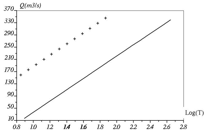
FIG. 7.7 – Distributions théoriques des débits de pointes d'un bassin fictif de 1000 km^2 d'après le modèle d'Hebson & Wood : a) F(Q_{max}) = 1 - \exp(-\beta Q_{max}/K A_r) (croix), b) distribution issue du modèle d'Hebson & Wood (trait continu).
