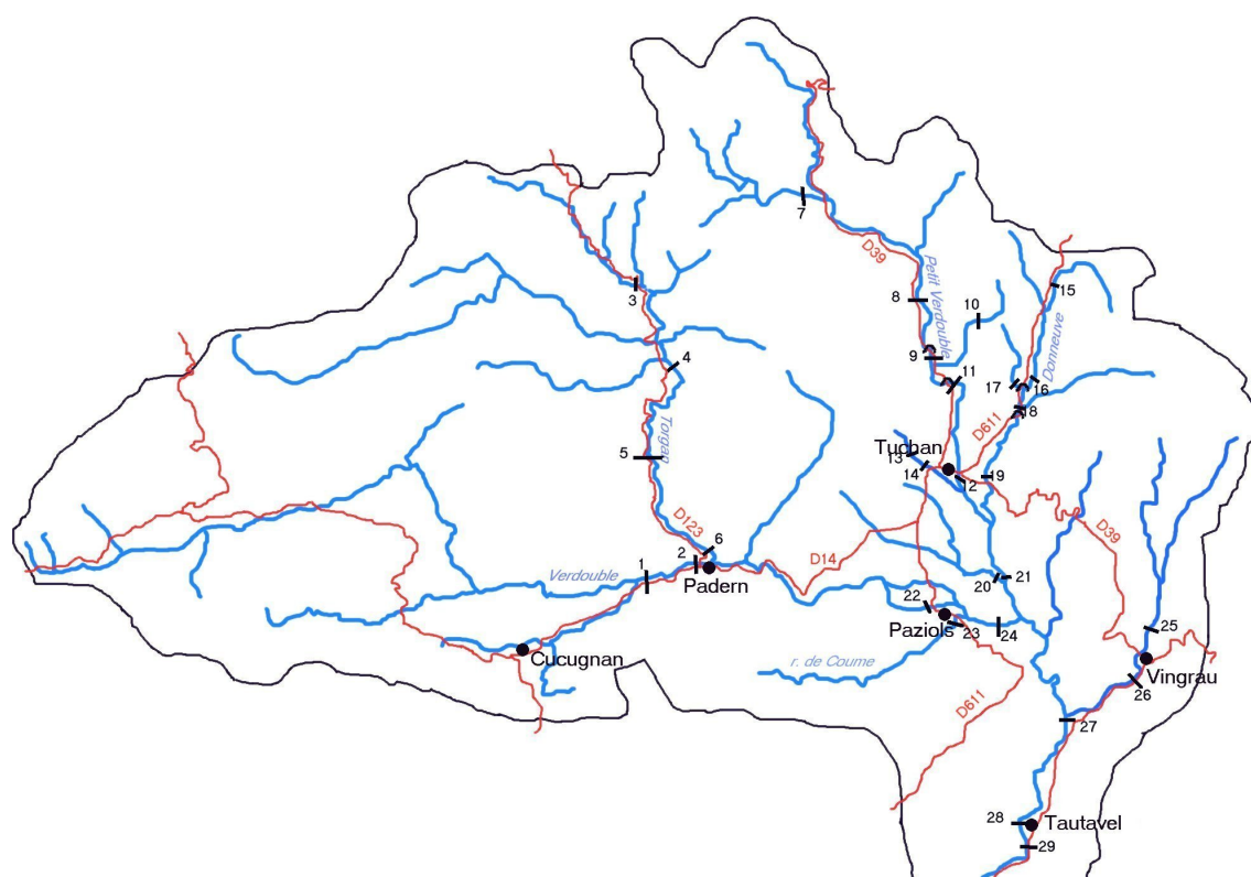
FIG. 4.14 – Le bassin versant du Verdoble, localisation des sections où ont été estimés des débits de pointe de crue
