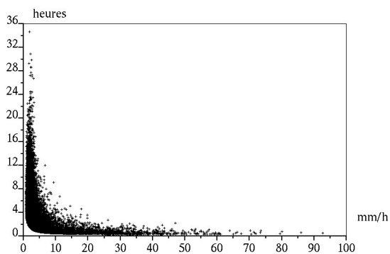
FIG. 8.9 – Dépendance entre les durées et intensités moyennes des événements pluvieux générés par le modèle stochastique de pluie.
