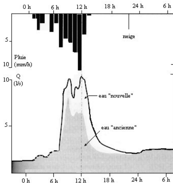
FIG. 2.1 – Décomposition isotopique de l'hydrogramme de la crue du 26 octobre 1981 d'un sous bassin de la Solenzara en Corse : 29 hectares, coefficient d'écoulement de 1.5% (Loye-Pilot & Jusserand, 1990)
