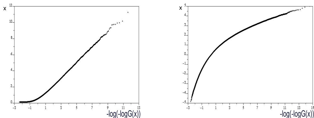
Loi exponentielle de moyenne 1
