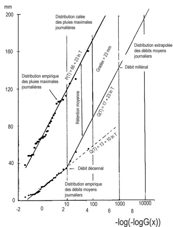
FIG. 6.7 – Exemple d'extrapolation d'une distribution empirique par la méthode du Gradex : cas des débits moyens maximums de la Loire en 24 heures exprimés en millimètres à la station de Brives Charensac, 35 années d'observations (Duband, 2000)
