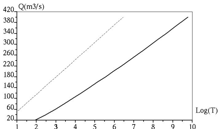
FIG. 7.9 – Distributions théoriques des débits de pointes de crues d'un bassin fictif de 100 \text{ km}^2 : a) Approximation de Diaz-Granados avec \beta = 1/0.1 \text{ h/cm} , \lambda = 1/3 \text{ h}^{-1} et K = 0.044 \text{ cm/h} , b) F(Q_{max}) = 1 - \exp(-\beta[(Q_{max}/A) + K]) (trait pointillé)
