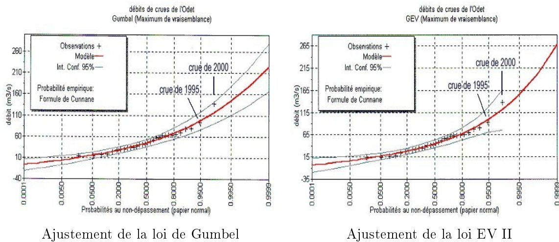
FIG. 6.3 – Intervalles de confiance à 95% sur les quantiles estimés à partir de l'ajustement des lois EV I et II sur une série de 30 valeurs de débits maximums annuels : cas de l'Odet à Quimper (source Service d'annonce des crues du Finistère). Calculs effectués à l'aide du logiciel HYFRAN (HYFRAN, 2002)
