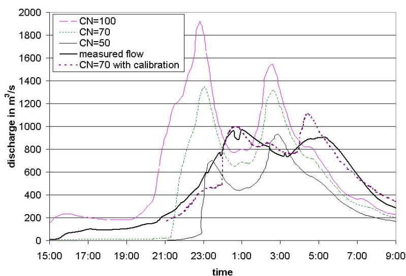
FIG. 4.21 – Comparaison entre l'hydrogramme de la crue du Verdoble des 12 et 13/11/99 reconstitué à partir des relevés limnimétriques de la station de Tautavel et différents résultats de simulations hydrologiques.
