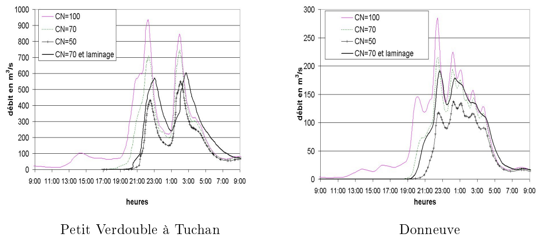
FIG. 4.19 – Résultats de simulations hydrologiques de la crue du Verdoble des 12 et 13/11/99.
