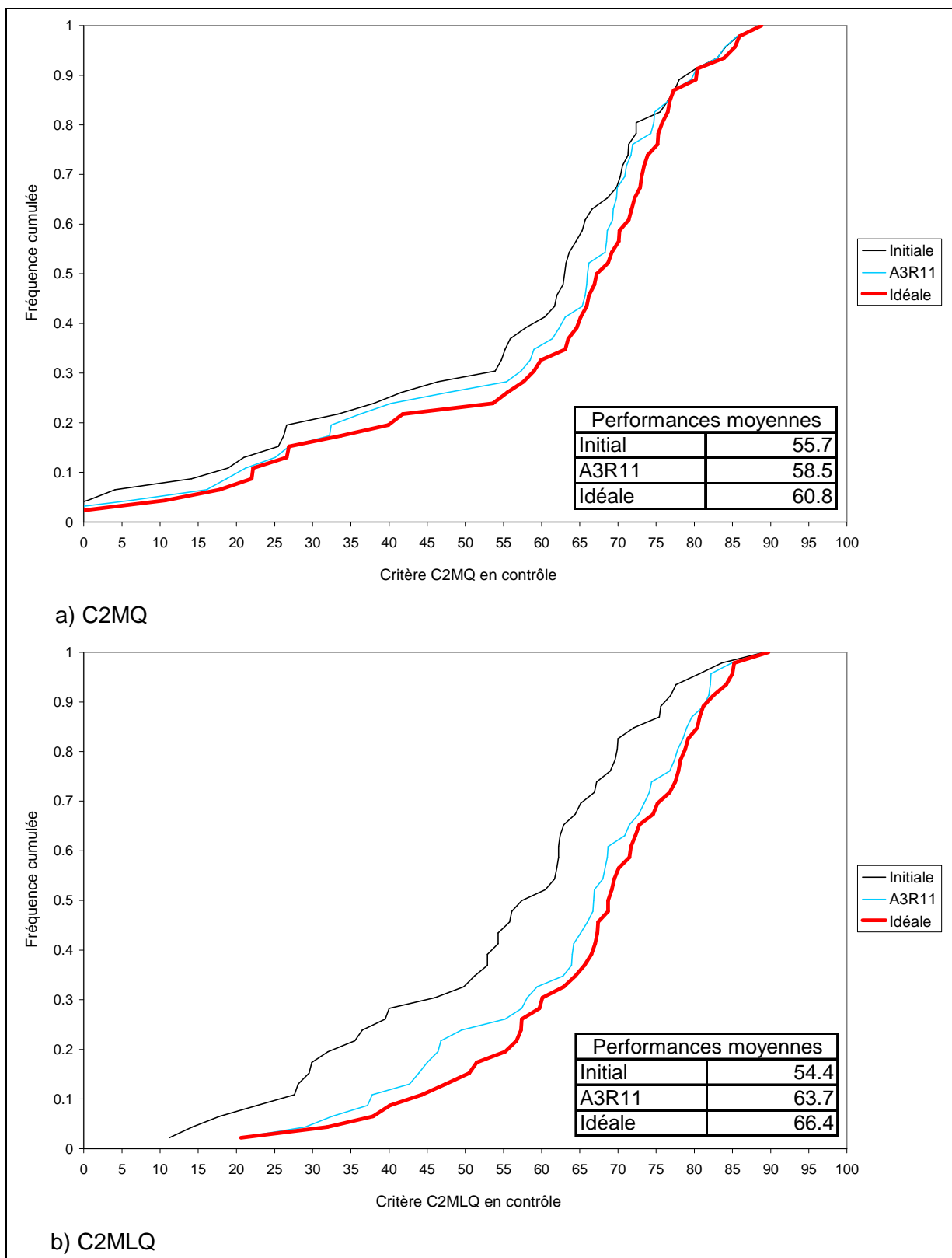
Figure 5.6 : Distributions des résultats par bassins suivant les critères C2MQ et C2MLQ pour la version initiale du modèle, la solution A3R11 et la solution "idéale"
