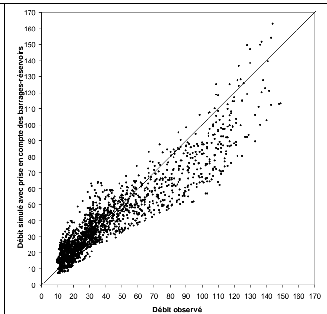
c) Comparaison entre débit observé et débit simulé avec la solution A3R11 ( m^3/s )
