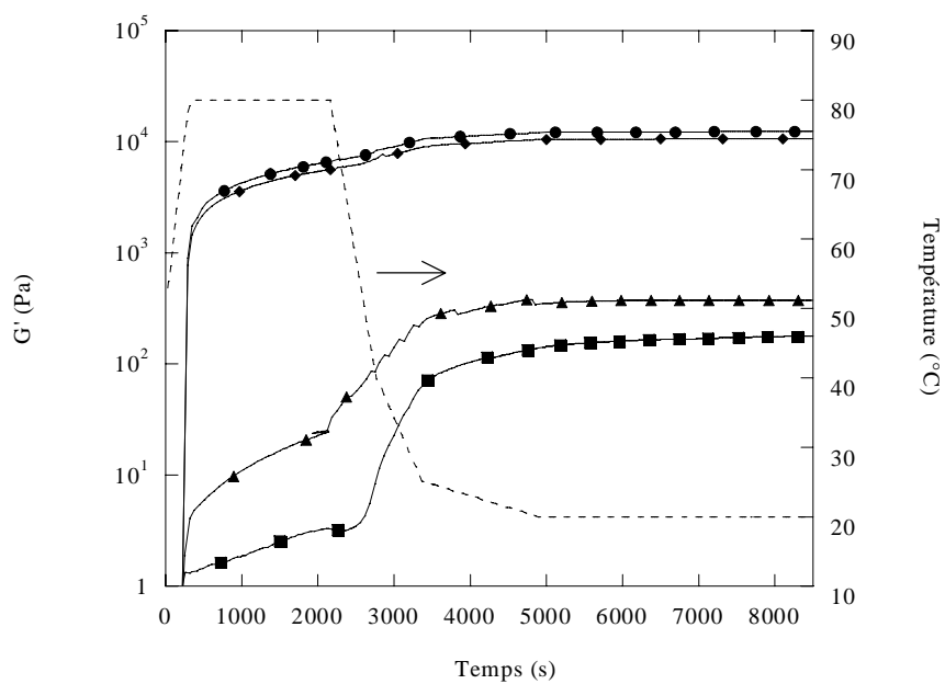
Figure IV.13. Gélification de la SAB 2 (○), 4 (◻) et 8 (△) % en absence (symboles vides) et en présence de 3 mM \text{CaCl}_2 (symboles pleins) dans NaCl 100 mM à pH 6,8.
