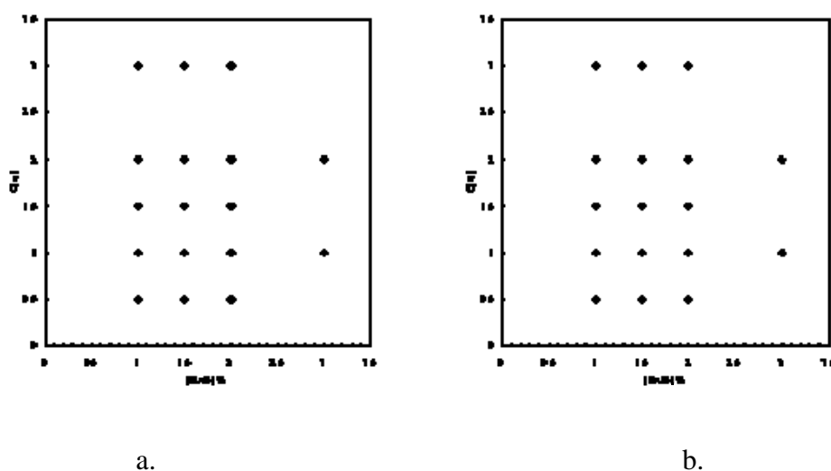
Figure IV.2 Diagrammes d'état des mélanges SAB/pectines LM (concentrations en pectines entre 0,21 et 1,3 %) observés à 20 \text{ }^\circ\text{C} (a) et après une centrifugation (2600 g, 3h) (b). Mélanges présentant une phase homogène (○) ou une séparation de phase macroscopique (⊗) (traitement thermique de 30 min à 80 \text{ }^\circ\text{C} ).
