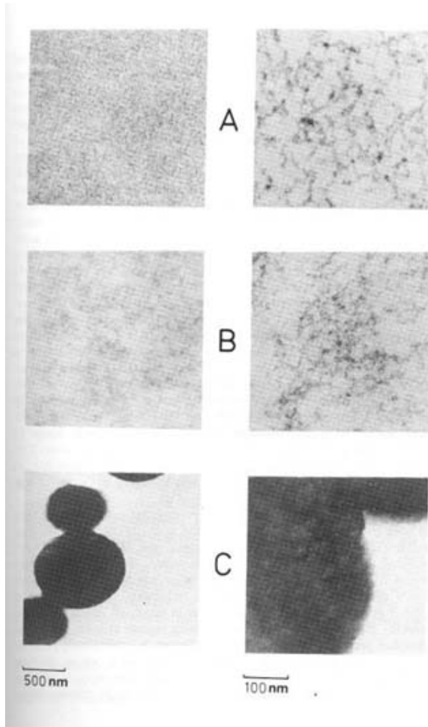
Figure I.9 Structures de gels de 10 % SAB en microscopie électronique (deux grossissements). A : gel fibrillaire clair obtenu à pH 6,5, dans l'eau; B : gel turbide obtenu en présence de NaCl 125 mM à pH 6,5; C : coagula obtenu à pH 5,1. D'après Clark et al. (1986).
