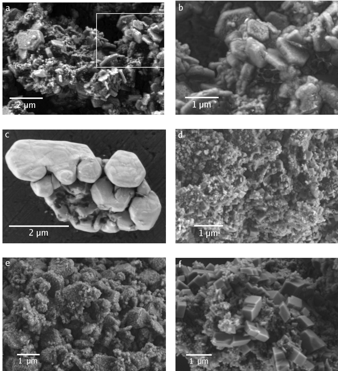
FIG. 4.13 – Photographies MEB de la fraction solide de l'expérience P_1 à 200^\circ\text{C} : après une minute de réaction (a), (b) et (c) ; après 5 minutes (d) et (e) ; après 30 minutes (f). Les angles arrondis des petites plaquettes hexagonales (a) et (b), mais aussi des plus gros éléments (c), évoquent la dissolution de la portlandite dès la première minute de la réaction. La calcite est alors visible à la surface des tablettes de portlandite sous forme de minuscules cristaux (b). À 5 minutes, la calcite est omniprésente : elle est cristallisée en rhomboédres d'une centaine de nm de côté (d). Des fantômes de portlandite, en cours de recristallisation, sont parfois conservés (e). Des cristaux de calcite plus épais ( 1\ \mu\text{m} ) apparaissent après 30 minutes de réaction (f).
