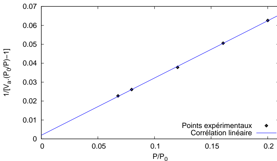
FIG. 2.11 – Isotherme d'adsorption BET à l'azote mesurée à 77\text{ K} pour la portlandite.
