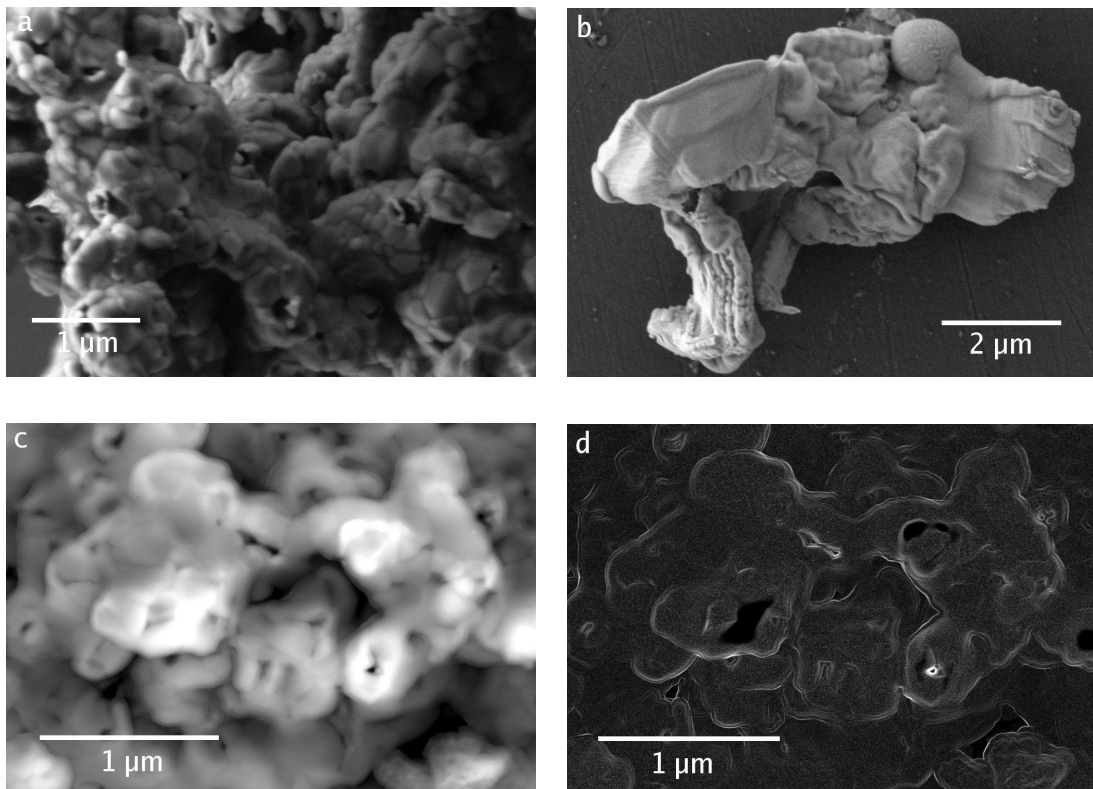
FIG. 4.18 – Photographies MEB de la fraction solide de l'expérience P_3 à 200^\circ\text{C} après une minute de réaction. La fraction fine de la poudre (a), tout comme les plus gros éléments (b), sont entièrement enrobés par une couche homogène de calcite. L'observation du même échantillon sous un faisceau plus intense fait apparaître une structure cœur (portlandite) / manteau (calcite) (c), mise en relief par une inversion de contraste (d).
