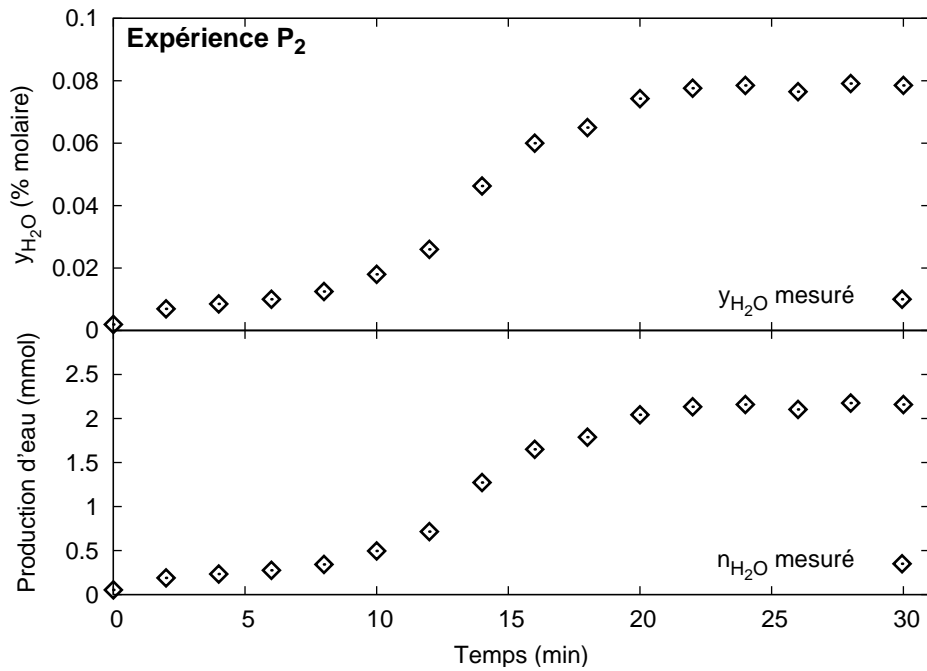
FIG. 4.8 – Évolution de la teneur en eau de la phase vapeur au cours de l'expérience P 2 à 200°C. La figure du haut représente l'évolution de la fraction molaire d'eau dans la phase vapeur, celle du bas, l'évolution du nombre de moles d'eau correspondant. L'erreur de la mesure, de l'ordre de 2%, est comprise dans la taille du symbole.
