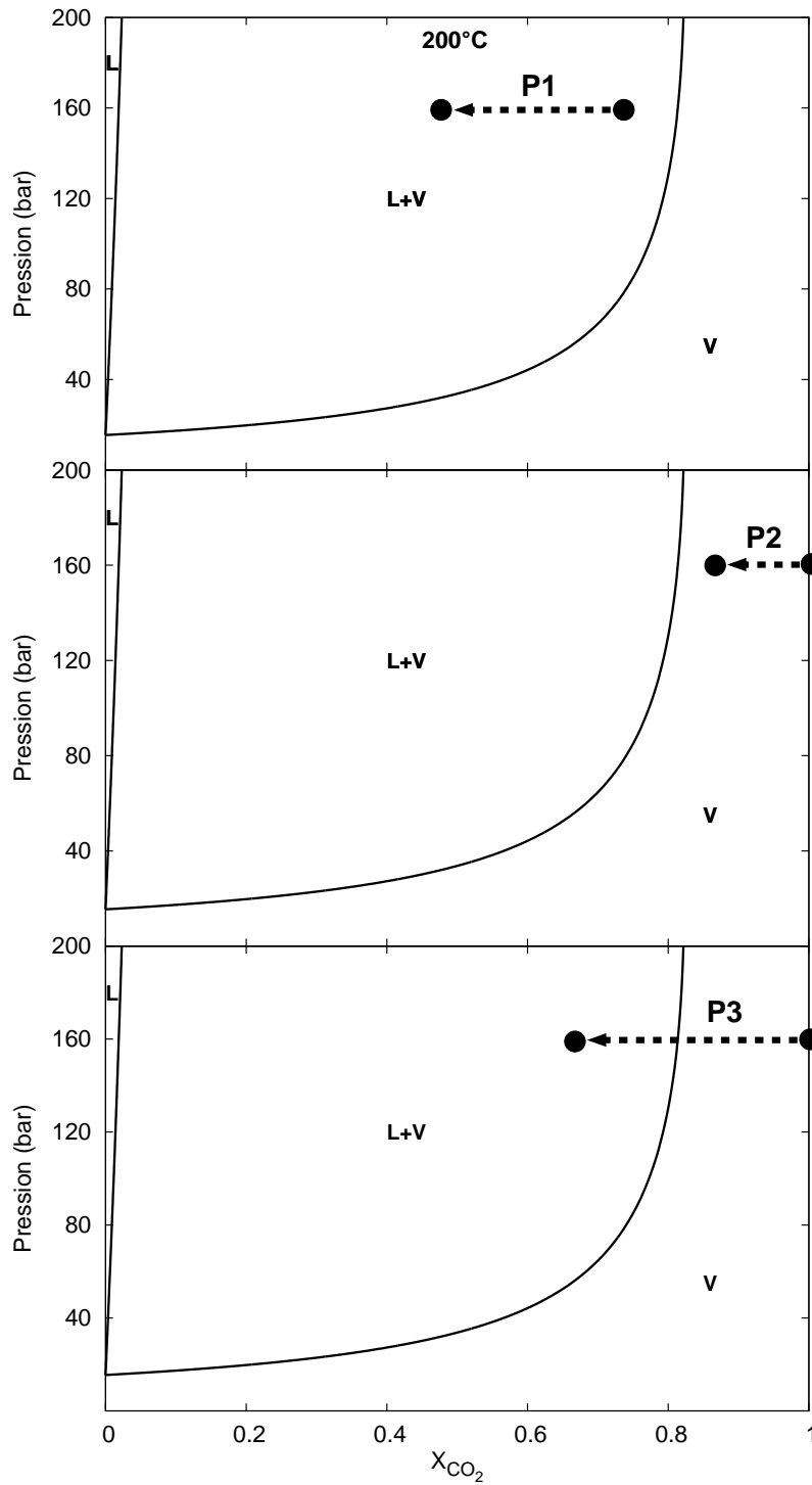
FIG. 2.2 – Évolution de la teneur en eau au cours des expériences P 1 , P 2 et P 3 à 200°C. L : liquide; V : vapeur.
