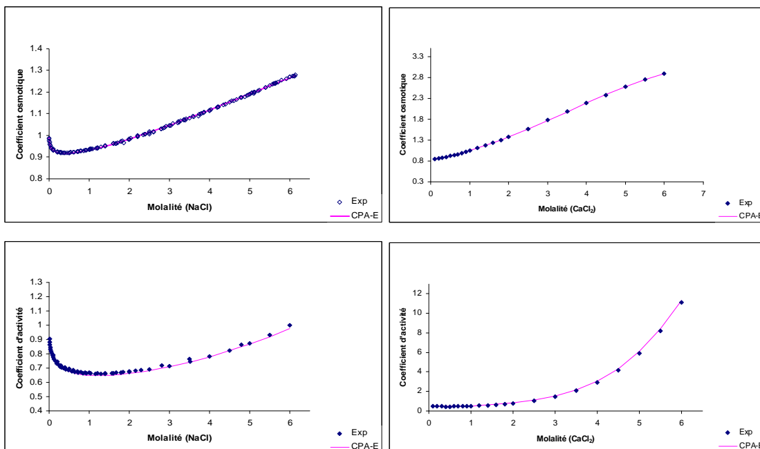
FIG.24 Coefficients osmotique et d'activité de NaCl et CaCl 2 à 25 °C, calculés avec le modèle CPA_Born en utilisant les paramètres du tableau 20.
