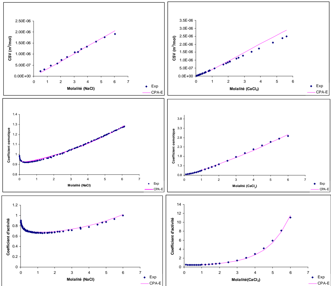
FIG.31 Propriétés de \text{NaCl} et \text{CaCl}_2 calculés au moyen du modèle \text{CPA\_Born} avec la fonction de Simonin, en utilisant les paramètres du tableau 25.
