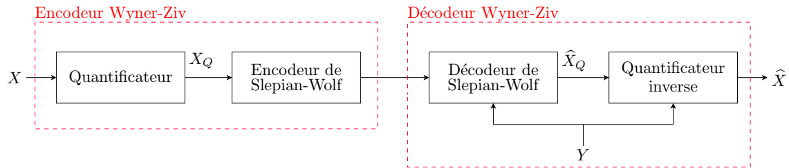
FIGURE 2.13 – Schéma d'un codeur de Wyner-Ziv.
