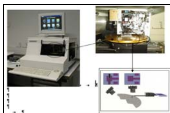
Fig. 5.6. Profilometria mecanică KLA-Tencor P-10
