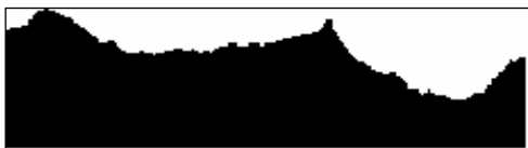
Fig. 5.16. Contour du profil obtenu par la méthode de Section Verticale sur l'éprouvette en acier inox 316L, (grossissement 50X)
