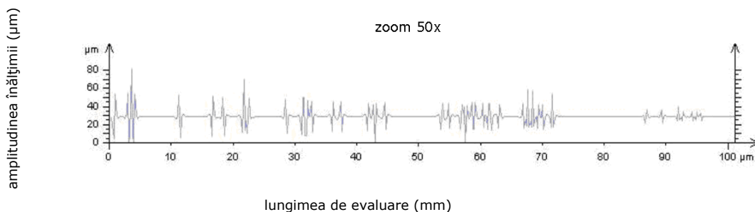
Fig. 6.1. Profilul rugozității suprafeței de rupere a epruvetei din oțel XC 65 netratat termic, realizat prin modul de scanare VSI, (puterea de mărire la microscop 50x)
