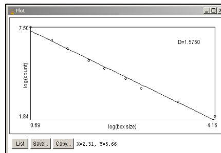
Fig. 5.29. Dimensiunea fractală obținută în programul Image J : \Delta=1,57
