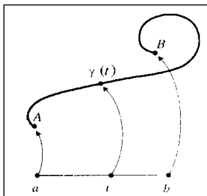
Fig.1.5. Curba A^B [Tricot C., 1999]
