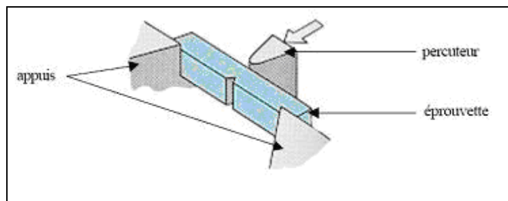
Fig. 6.15. Principe du choc Charpy
