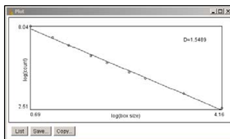
Fig. 5.45. Dimensiunea fractală obținută în programul Image J : \Delta=1,54
