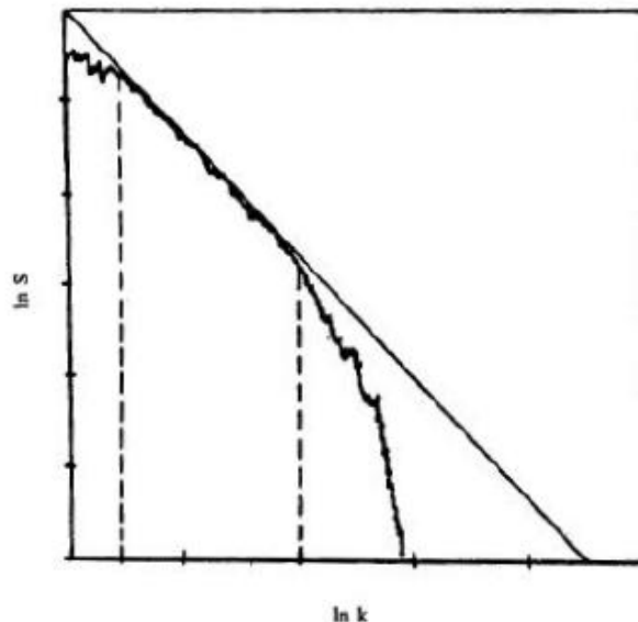
Fig. 2.7. Spectru Fourier caracteristic pentru profilul unei suprafețe de rupere [Cherepanov G.P. ș.a., 1995]
