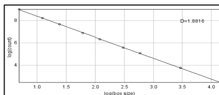
Fig.5.19. Calculul dimensiunii fractale a profilului de rupere: \Delta=1.88 cu programul Image J
