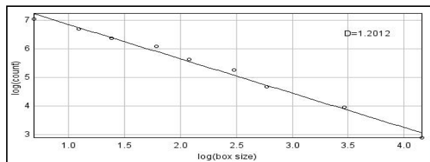
Fig.6.8. La dimension fractale du profil de rugosité de la surface de rupture par le programme Image J : \Delta=1,20
