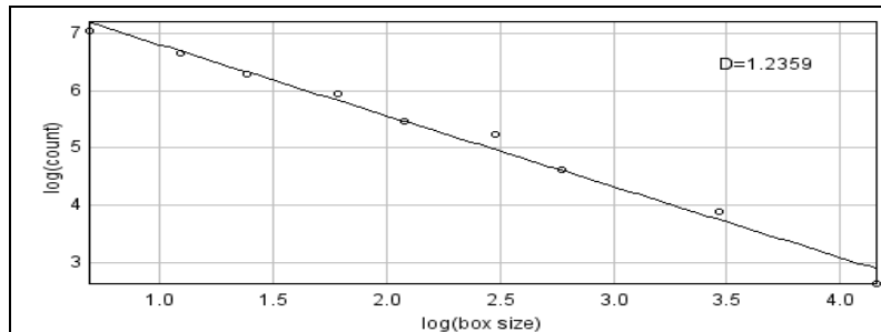
Fig. 6.6. La dimension fractale du profil de rugosité de la surface de rupture par le programme Image J : \Delta=1,23
