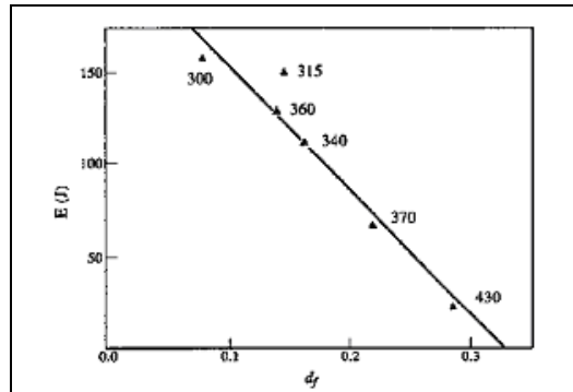
Fig.3.5. L'énergie à l'impact E en fonction de la dimension fractale de la surface de rupture, d_f . Les chiffres indiquent la température à laquelle l'essai a été effectué [Cherepanov, 1995]
