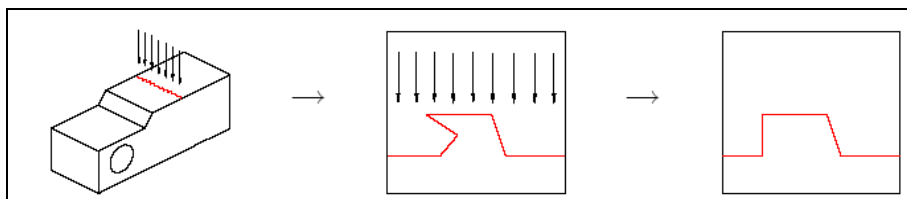
Fig. 3.4. Exemple d'utilisation de la technique de mesure du profil [Katowski P, 2006]
