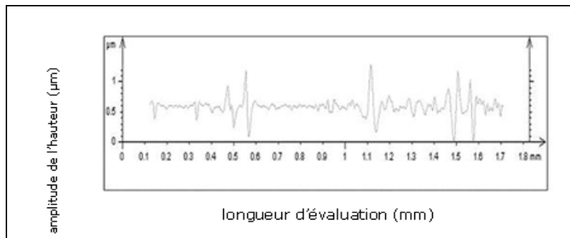
Fig. 5.63. Profil de la rugosité de la surface de rupture pour l'échantillon en verre de silice
