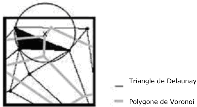
Fig. 6.18. Triangulation de Delaunay et le polygone de Voronoi
