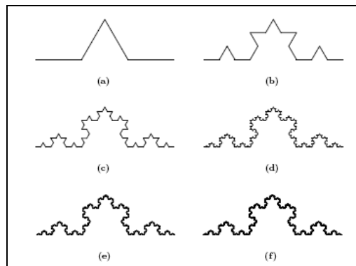
Fig.1.1.1. Courbe de Von Koch (par six itérations)
