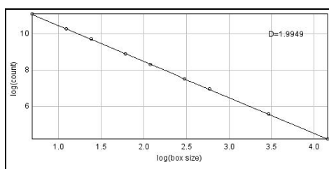
Fig. 6.4. Dimensiunea fractală a profilului rugozității suprafeței de rupere a probei din oțel XC 65 călit în programul Image J: \Delta=1,99
