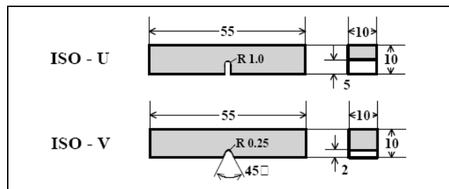
Fig. 6.17. Eprouvettes Charpy normalisées
