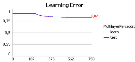
Figure 204 - Graphe d'apprentissage d'un Perceptron Multicouches à 1 neurone sur la couche cachée sur la base de chiffres
