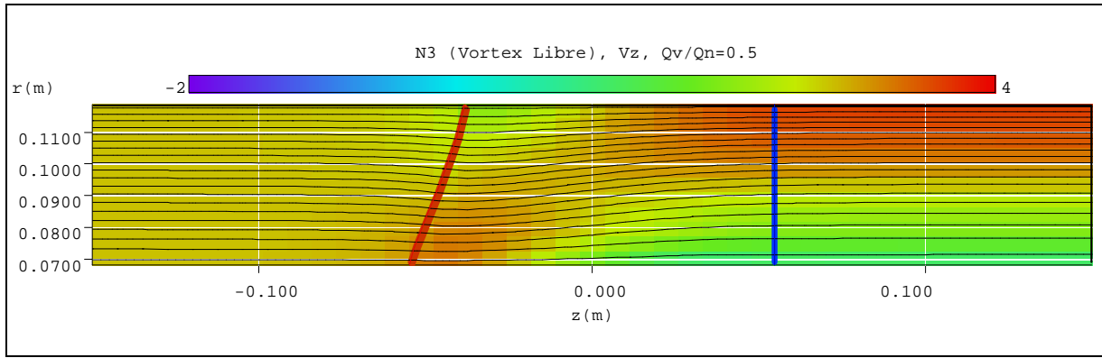
Figure III.36 Vitesses axiales - Pompe N3 en débit partiel ( Q_v/Q_n = 0,5 ) empilement des pales sur l'arrière.
