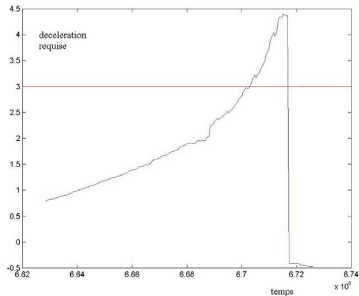
Figure 67 : décélération requise en arrivée sur virage
