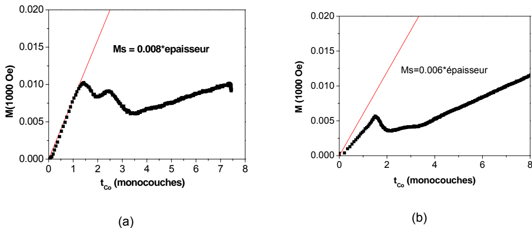
Figure 5.18 - Evolution M(H = 1000 \text{ Oe}) et M_s(t_{Co}) . (a) Pour un dépôt Co/Au/Si(111)-0.2° ( U = -1.4 \text{ V} ). (b) Pour un substrat Au/mica.
