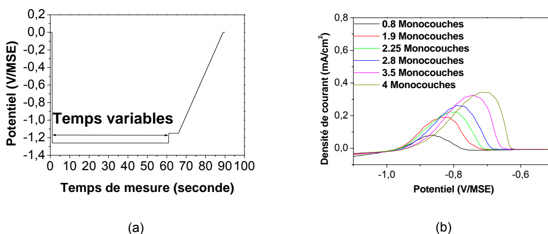
Figure 4.7 : (a) Séquence de potentiel utilisée pour réaliser des dépôts de cobalt d'épaisseur variable à -1.26 VMSE. La concentration en \text{CoSO}_4 est 1 \text{ mM} . Le potentiel est ensuite fixé à -1.15 VMSE pour stabiliser le dépôt. Une rampe de potentiel ( 50 \text{ mV/seconde} ) est ensuite appliquée jusqu'à 0 \text{ V/MSE} pour dissoudre entièrement le film de cobalt. (b) Pics de dissolution du cobalt en fonction de l'épaisseur du film. Noter le décalage progressif de la montée du pic anodique avec l'épaisseur de cobalt.
