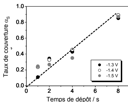
Figure 4.16 : Evolution du taux de couverture de la surface \alpha_s en fonction du temps de dépôt. Données issues des images STM des figures 4.10, 4.11, 4.12. Noter que les épaisseurs de cobalt varient entre 0 et 2 monocouches car les îlots ont une hauteur biatomique. Noter en outre que \alpha_s dépend peu du potentiel appliqué, conformément aux mesures électrochimiques (cf. figure 4.8 ).
