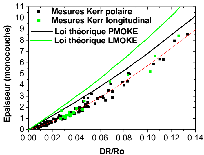
Figure 5.8 - Corrélations entre l'épaisseur t_{Co} et \Delta R/R_0 pour un ensemble d'expériences PMOKE et MOKE longitudinal. Noter le bon accord entre les différentes mesures qui se placent sur une même courbe. La courbe en rouge est le meilleur polynôme du 3 ème degré représentant les mesures expérimentales, la courbe verte est la-courbe théorique du système à trois couches solution/Co/Au(100 nm).
