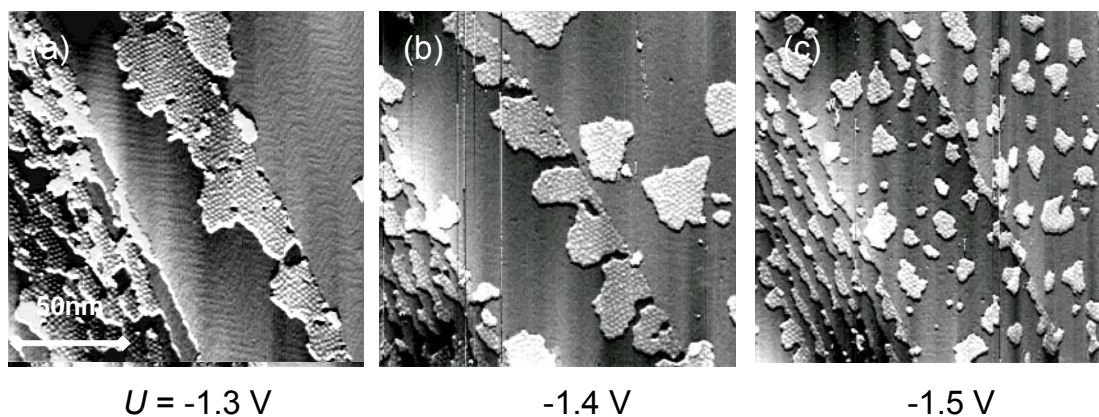
Figure 4.9 - Images STM in situ en mode « différentiel » pour mieux révéler le contraste de surface (170 nm x 170 nm) montrant la nucléation d'un dépôt Co/Au(111) à différents potentiels : (a) -1.3 V ; (b) -1.4 V ; (c) -1.5 V. Le temps de dépôt est 2s (a) et 1s (b, c). Noter l'évolution de la distribution des îlots de cobalt (hauteur biatomique). Le taux de couverture \alpha_S \sim 0.25 dans les trois images.
