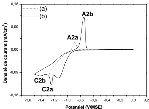
Figure 4.6 : Voltammogrammes mesurés dans une solution 1 mM de \text{CoSO}_4 de \text{pH}=3.5 à une vitesse de balayage de 10 mV/s. Courbe (a) : la borne cathodique de balayage est -1.28 V_{MSE} . Noter que dans ce cas, la charge de dissolution sous le pic anodique est équivalente à deux plans atomiques. Courbe (b) : idem mais pour une borne cathodique -1.5 V_{MSE} .
