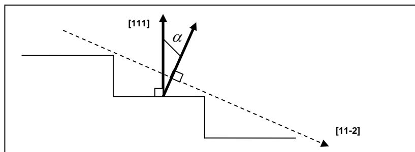
Figure 2.13 – L'angle \alpha est l'angle entre l'axe optique [11-2] et la normale aux terrasses [111]. L'augmentation du miscut entraîne la diminution de la largeur des marches.
