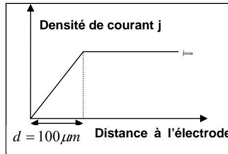
Figure 2.6 – Profil de concentration des espèces Mz+ résultant de leur consommation dans la réaction de réduction M^{z+} + ze^- \rightarrow M . L'épaisseur de la couche de diffusion est environ 100 \mu\text{m} pour une électrode stationnaire.
