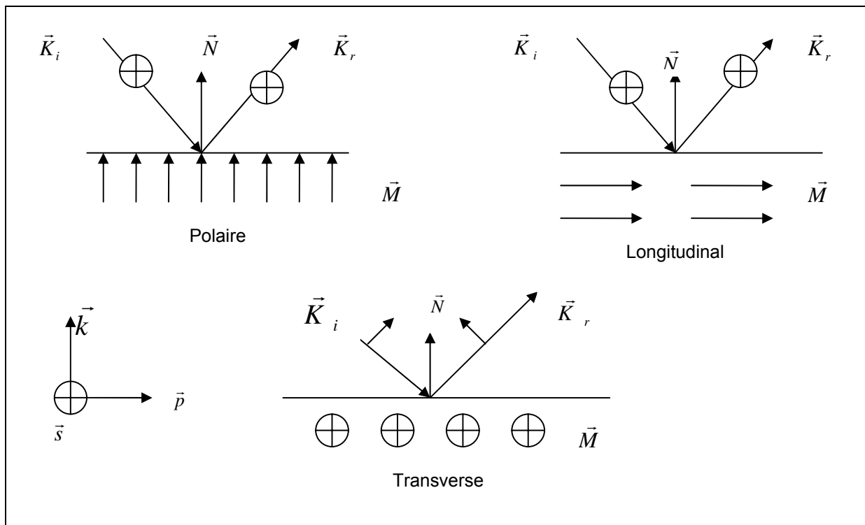
Figure A2.2 - Les trois types d'effet Kerr
