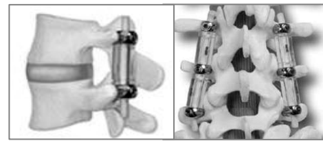
Figure 48 : Instrumentation dynamique : Dynesys.
