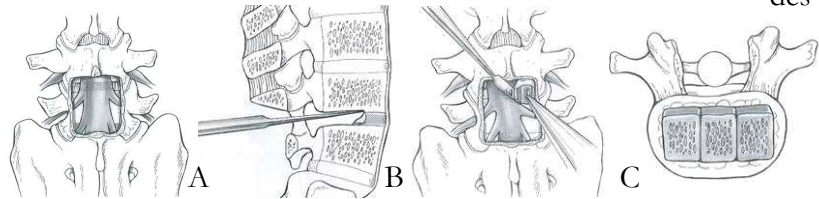
Figure 38 : PLIF : A. laminectomie (ici pour 2 niveaux) B. dissectomie et avivement des plateaux C. insertion du greffon Larson'99 .
