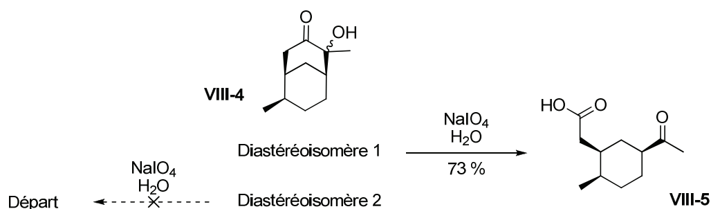
Schéma VIII-13 – Différence de réactivité entre diastéréoisomères vis-à-vis de la coupure oxydante.
