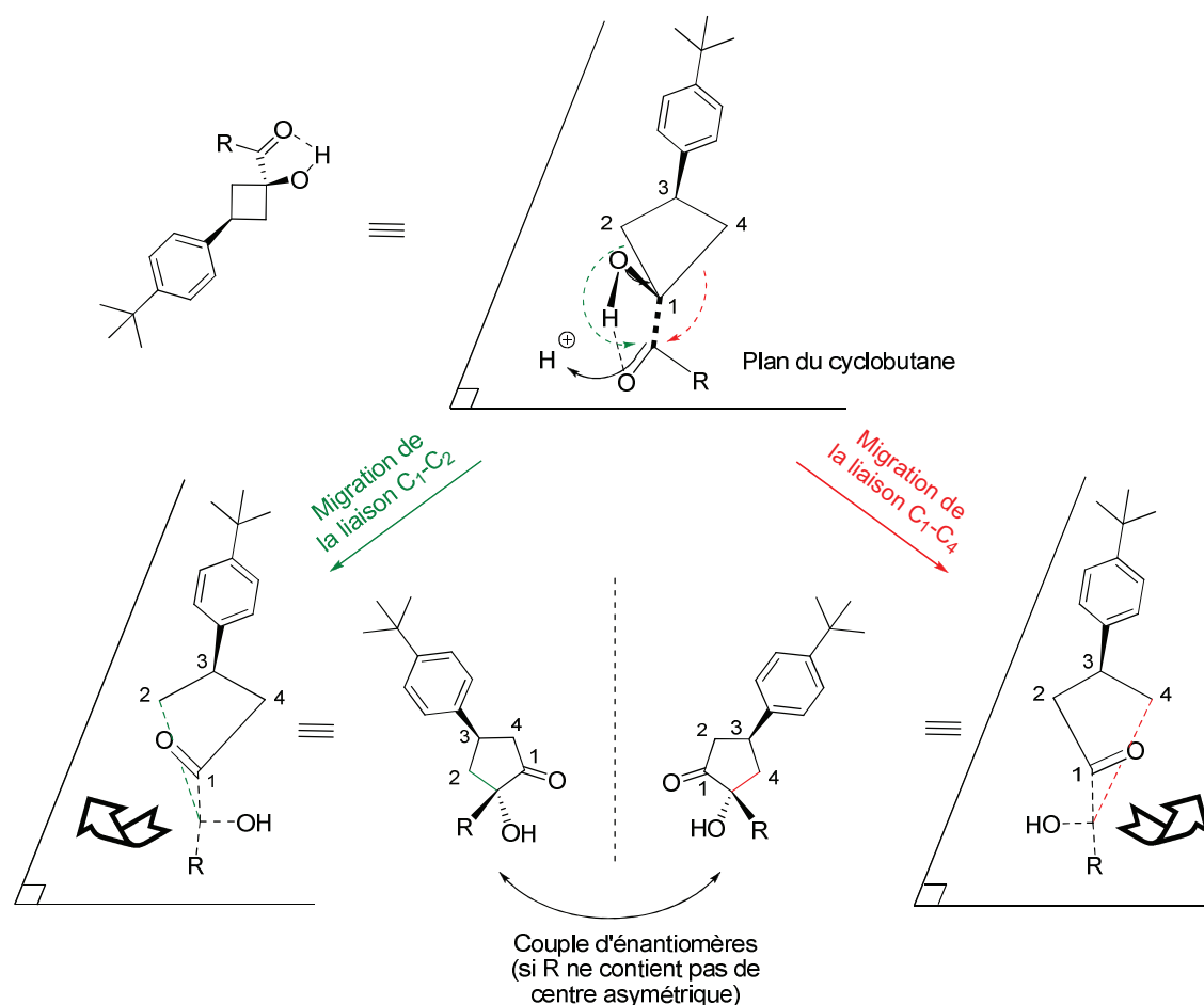
Schéma V-16 – Agrandissement de cycle diastéréocontrôlé.
