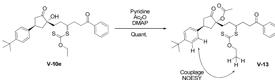
Schéma V-17 – Vérification de la stéréochimie par une expérience NOESY.
