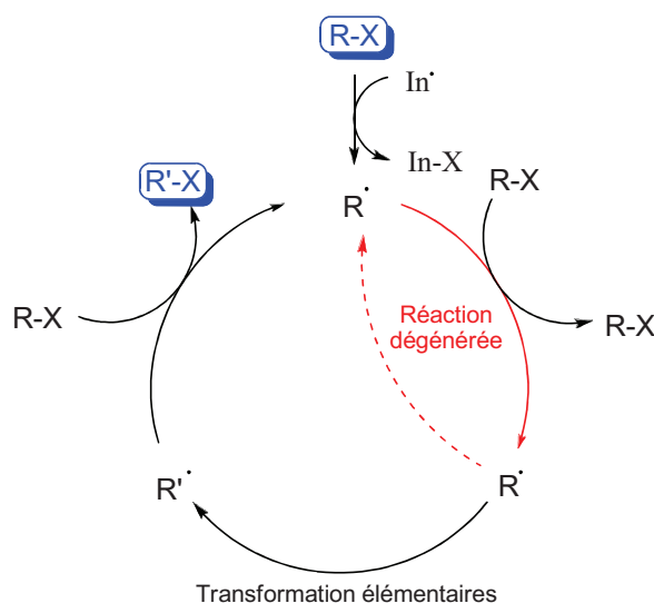
Schéma I-15 – Réaction radicalaire par transfert d'atome ou de groupe.
