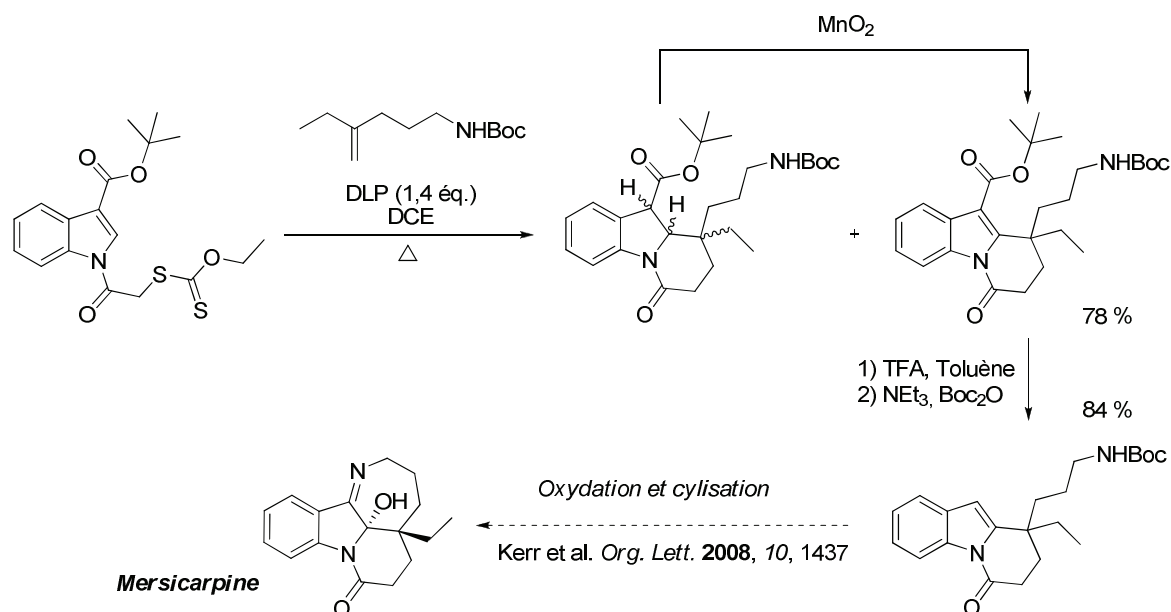
Sch\u00e9ma II-22 – Application de la chimie des xanthates \u00e0 la synth\u00e8se formelle de la mersicarpine.
