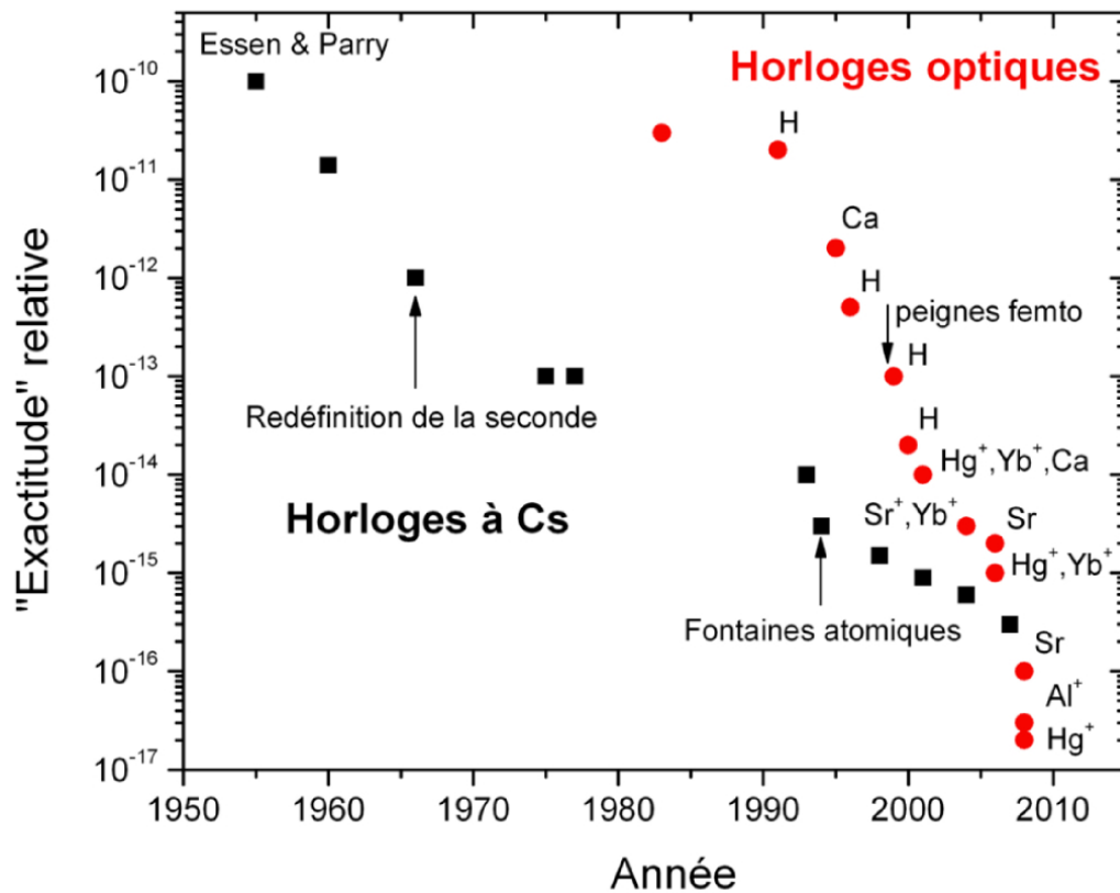
FIGURE 2 – L'évolution de l'exactitude des horloges atomiques au cours des 60 dernières années.
