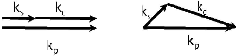
Figure 27 : Géométrie d'accord de phase colinéaire à gauche et non colinéaire à droite.
