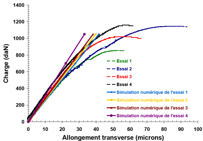
Figure VIII.10 – Charge vs allongement, comparaison essais/simulations élastiques sur échantillon en carbone/PPS en mode II avec quatre séquences d'empilement : 0° sens chaîne pour l'essai 1, 0° sens trame pour l'essai 2, 0°/+20°/-20°/0°/-20°/+20°/0° pour l'essai 3 et 0°/+45°/0°/+45°/0°/-45°/0° pour l'essai 4 (essais en trait pointillé sans marque, simulations numériques en trait plein avec marques)
