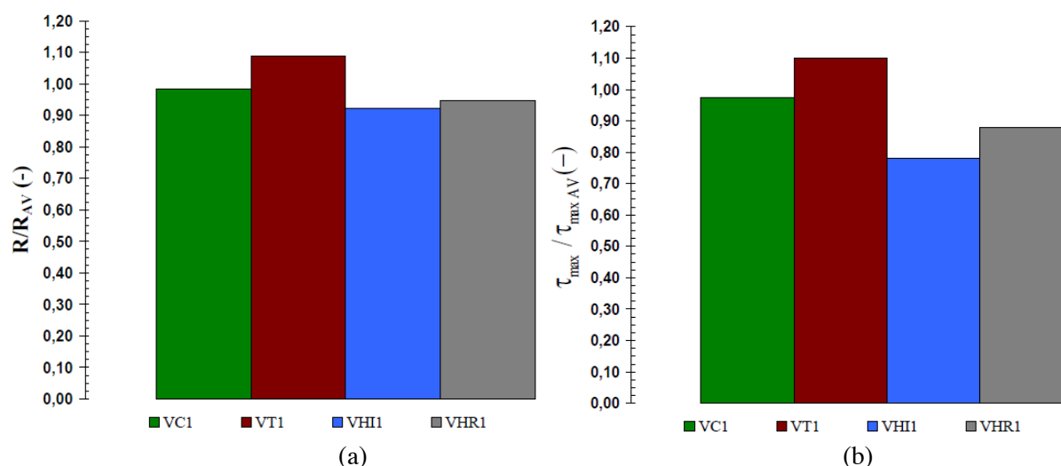
Figure XI.18 – Résultats des essais de flexion trois points à appuis rapprochés après vieillissements (distance entre appuis de 1 mm) (a): Ratio R/R_{AV} , (b): Ratio \tau_{max} / \tau_{maxAV}
