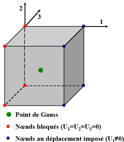
Figure VII.2 – Élément unitaire nécessaire à la simulation numérique
