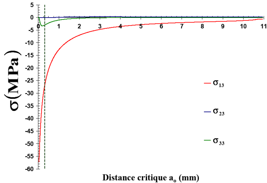
Figure IX.21 – Evolution des contraintes antiplanes le long de l'interface -20^\circ/+20^\circ (en pointillés noirs la distance critique égale à un pli)
