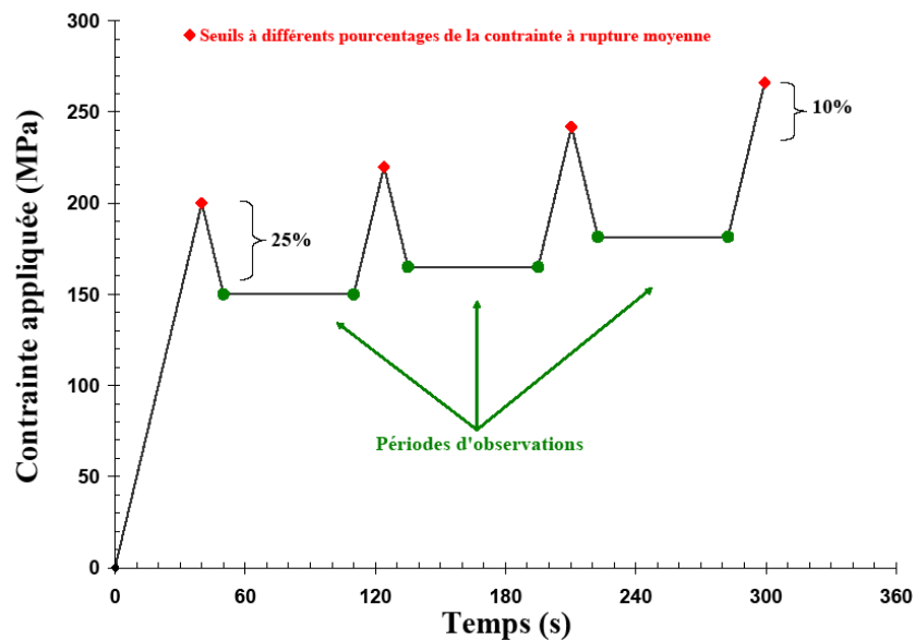
Figure IX.14 – Consigne imposé lors des essais de traction plane avec observations in-situ de l'endommagement
