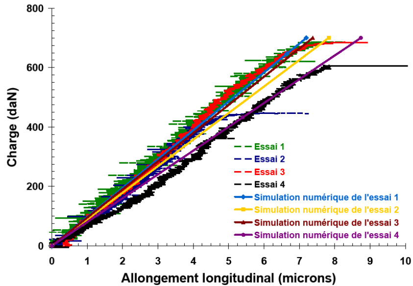
Figure VIII.9 – Charge vs allongement, comparaison essais/simulations élastiques sur échantillon en carbone/PPS en mode I avec quatre séquences d'empilement : 0° sens chaîne pour l'essai 1, 0° sens trame pour l'essai 2, 0°/+20°/-20°/0°/-20°/+20°/0° pour l'essai 3 et 0°/+45°/0°/+45°/0°/-45°/0° pour l'essai 4 (essais en trait pointillé sans marque, simulations numériques en trait plein avec marques)
