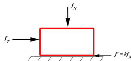
Figure IX.3 – Relation entre effort normal et effort tangentiel par la loi de Coulomb
