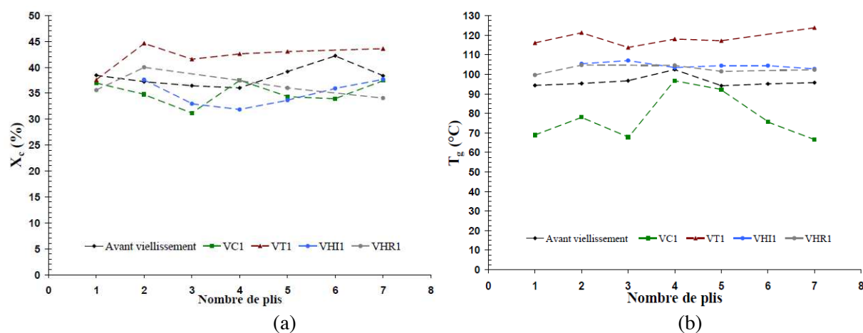
Figure XI.15 – Evolutions des propriétés physico-chimiques par plis obtenues par essais de mdsc avant et après vieillissements ; (a) : T_g , (b) : X_c
