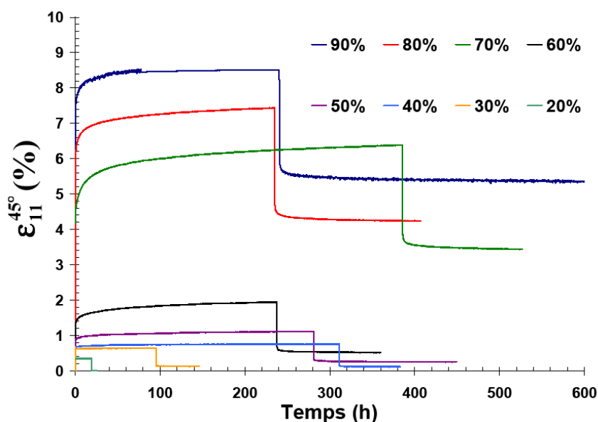
Figure IV.14 – Déformation longitudinale vs temps, essais de fluage-recouvrance pour l'ensemble des contraintes imposées (20, 30, 40, 50, 60, 70,80 et 90% de la contrainte moyenne à rupture) sur éprouvettes découpées à 45° de composite tissé satin 5 carbone/PPS
