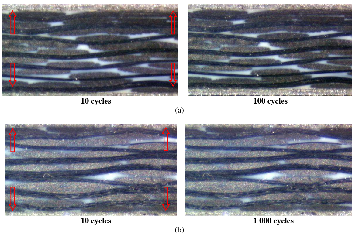
Figure X.18 – Observations optiques in-situ lors des essais Arcan-Mines en mode I (traction) et en fatigue sur du carbone/PPS consolidé à sept plis tissés à 0° : (a) Essai 1 soit \sigma_{max} = 90\% Y_T^{Statique} , (b) Essai 2 soit \sigma_{max} = 80\% Y_T^{Statique} (flèches rouges : sens de sollicitation)
