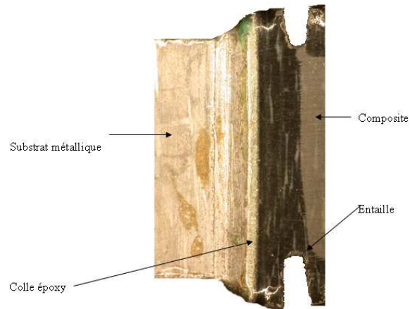
Figure V.4 – Détail de l'éprouvette pour essais Arcan-Mines sur composite tissé satin 5 de carbone/PPS
