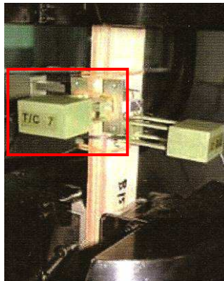
Figure III.29 – Instrumentation d'une éprouvette de traction avec trois capteurs extensométriques permettant de mesurer les déplacements dans les trois directions (rectangle rouge : celui chargé de la mesure de la contraction de l'éprouvette lors de l'essai)
