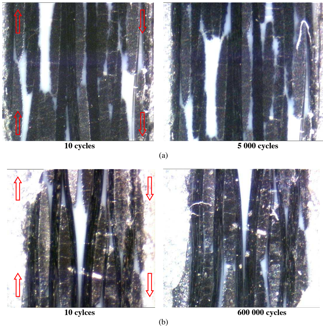
Figure X.19 – Observations optiques in-situ lors des essais Arcan-Mines en mode I (traction) et en fatigue sur du carbone/PPS consolidé à sept plis tissés à 0^\circ : (a) Essai 1 soit \tau_{\max} = 95\% S^{\text{Statique}} , (b) Essai 2 soit \tau_{\max} = 90\% S^{\text{Statique}} (flèches rouges : sens de sollicitation)
