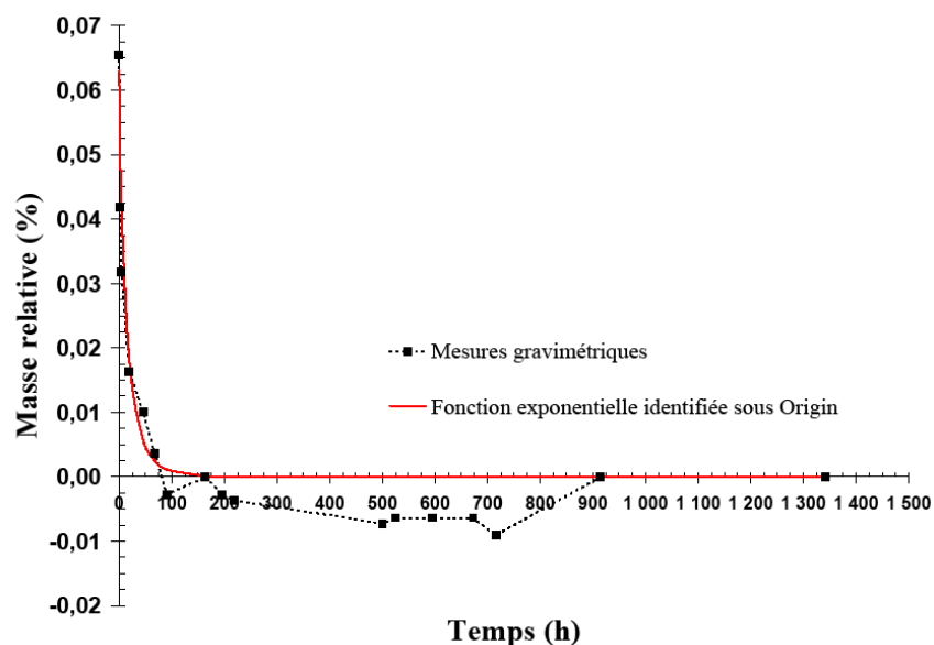
Figure XI.8 – Masse relative vs temps, comparaison entre la courbe expérimentale et celle de la fonction exponentielle (XI.6) identifiée sous Origin lors du maintien à 70°C du carbone/PPS consolidé (pesées en trait pointillé avec marques, modèle en trait plein sans marque)
