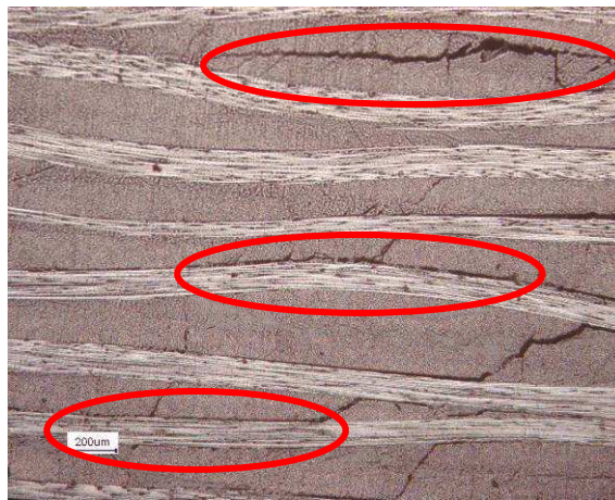
Figure III.24 – Décohésions des couches observées par microscopie optique après essais de flexions trois points pour une distance entre appuis de 11mm (en rouge les fissures délaminantes)
