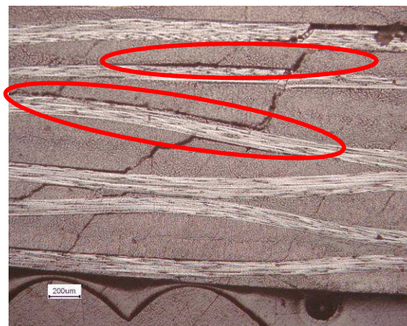
Figure XI.20 – Décohésions des couches observées par microscopie optique après essais de flexions trois points pour une distance entre appuis de 11mm (en rouge les fissures délamifiantes) pour une éprouvette vieilli par immersion dans de l'eau à 70°C
