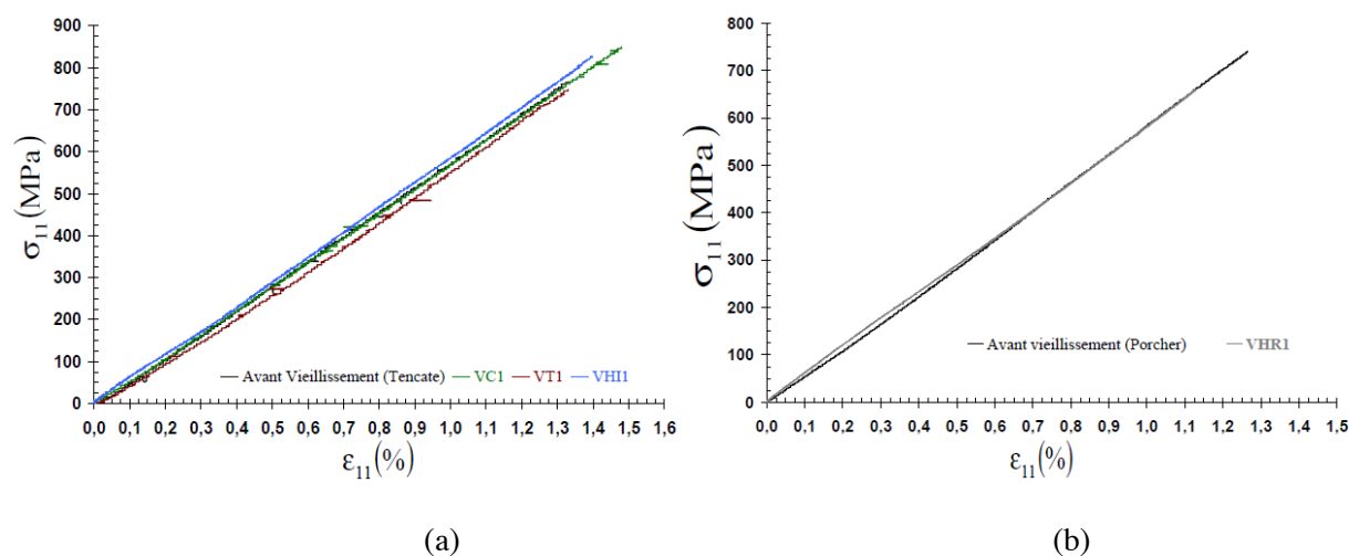
Figure XI.17 – Contrainte vs Déformation longitudinale, essais de traction dans le sens chaîne avant et après vieillissements ; (a): épreuves de chez Tencate, (b): épreuves de chez Porcher
