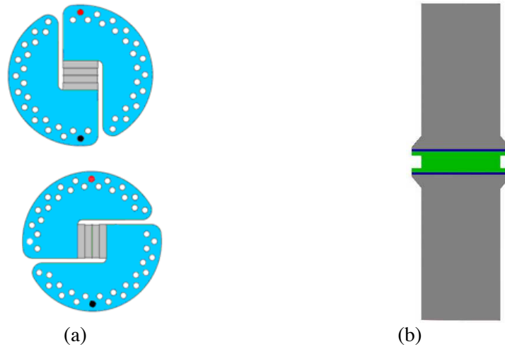
Figure V.1 – (a) Illustrations de deux configurations utilisées : traction (angle 0^\circ ) et cisaillement (angle 90^\circ ) avec en bleu : les disques en acier, en gris : les substrats métalliques, en vert : l'échantillon en composite, en rouge : le point d'application de la charge, en noir : le point de fixation, (b) Vue de profil de l'assemblage hybride et collé (en bleu : l'adhésif époxy)
