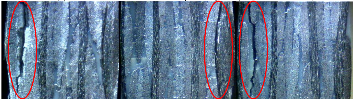
(e) Palier à 90% de la contrainte à rupture moyenne (soit environ 410MPa)
