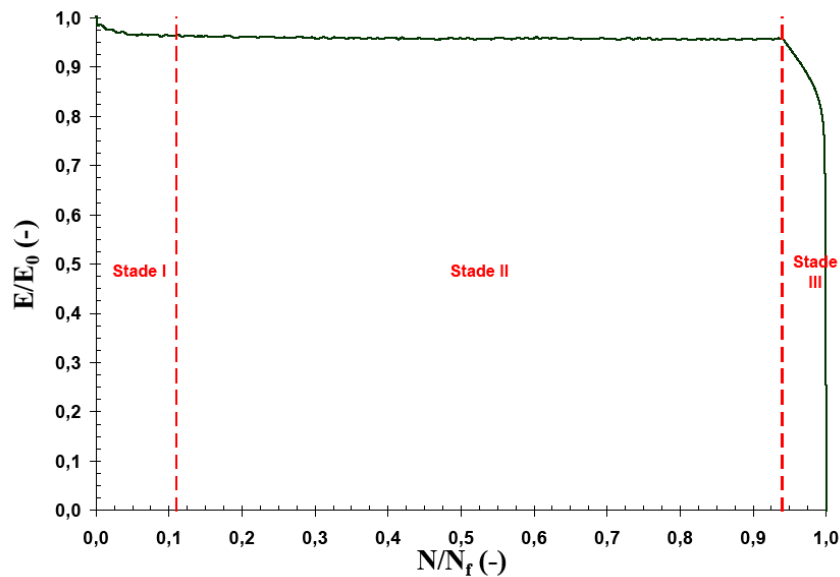
Figure X.2 – Evolution de la rigidité en fatigue de type traction-traction pour une éprouvette de carbone/époxy
