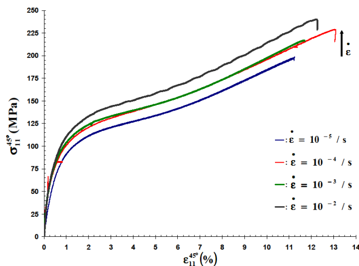
Figure III.8 – Contrainte vs déformation, essais de traction à 45°
