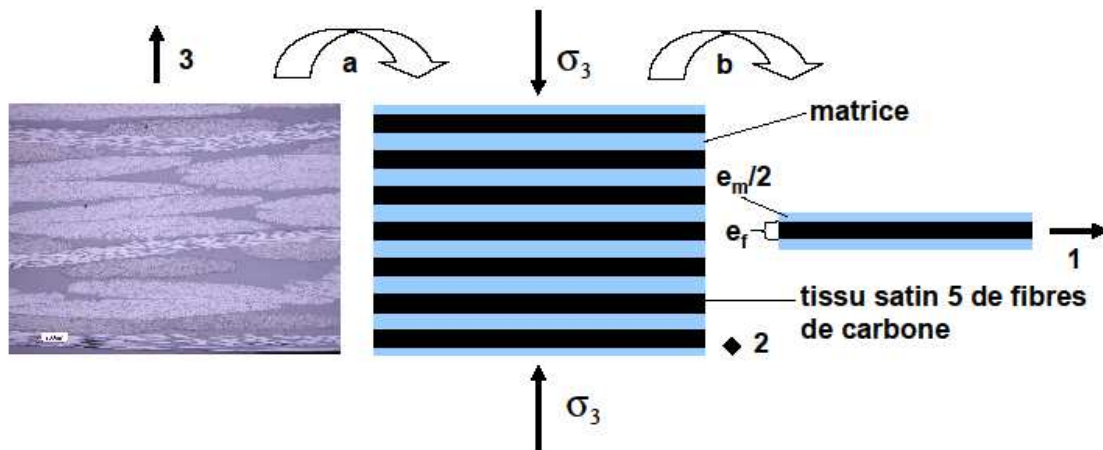
Figure III.15 – Représentations du composite tissé satin 5 carbone/PPS constitué de 7 plis à 0° lors d'un essai de compression
