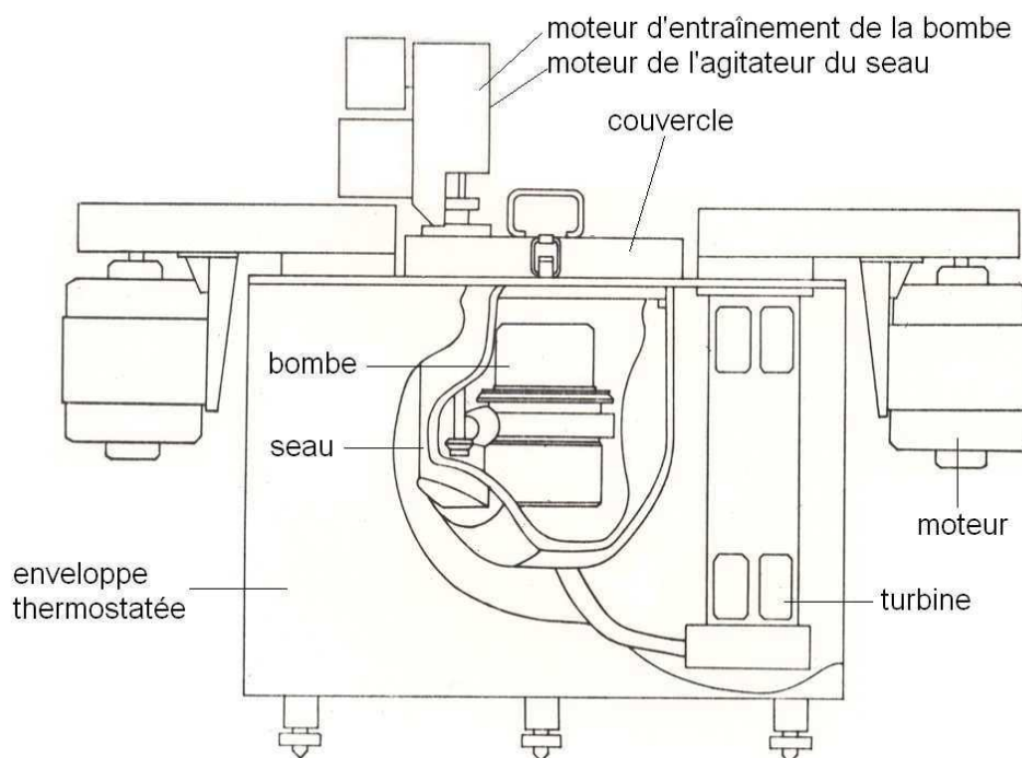
Figure 6 : vue du calorimètre assemblé.
