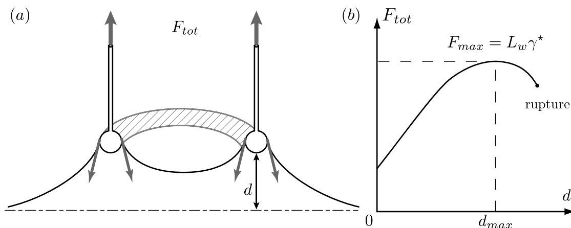
FIGURE A.2 (a) Résultantes des forces capillaires F_{tot} exercées par le liquide sur l'anneau de platine à une distance d au-dessus du bain. (b) Courbe typique de la force F_{tot} exercée sur l'anneau en fonction de la hauteur d au dessus du bain. La force est maximale lorsque les forces résultantes aux lignes de contact sont purement verticales.
