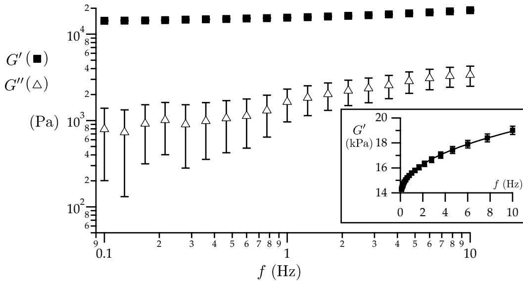
FIGURE 4.10 Modulus de cisaillement G' et de pertes G'' de l'élastomère utilisé en fonction de la fréquence, mesuré trois heures après le moulage. Les échelles sont logarithmiques. En insert est représenté le détail de l'évolution de G' en échelle linéaire. Un ajustement par une loi de puissance et une constante est réalisée pour extrapoler la valeur à fréquence nulle. On observe que l'élastomère possède un bon comportement élastique car G' est constant pour ces basses fréquences et que G'' \ll G' .
