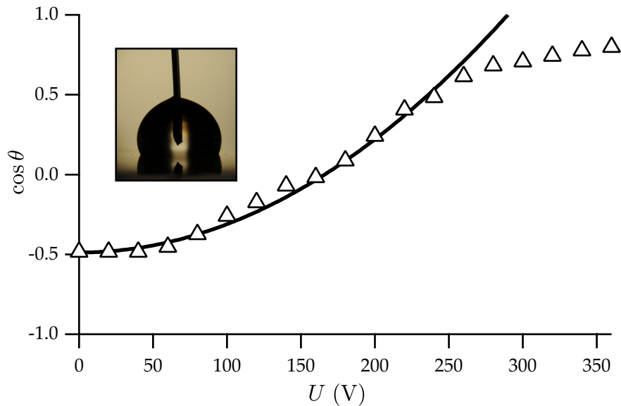
FIGURE 2.33 Expérience classique d'électromouillage. Le liquide est de l'eau avec une concentration de \text{Na}^+\text{Cl}^- à 10^{-2} \text{ mol L}^{-1} , et le substrat est du PDMS réticulé de permittivité relative 2,7 et d'épaisseur 9,5 \mu\text{m} . Les triangles sont les points expérimentaux, et la taille des points correspond à l'erreur sur la mesure de l'angle de contact. La courbe noire correspond à la courbe théorique (2.126). On observe un phénomène de saturation vers U \approx 250 \text{ V} . En insert, l'image d'une de ces gouttes, où on aperçoit l'électrode de platine en contact avec le liquide.
