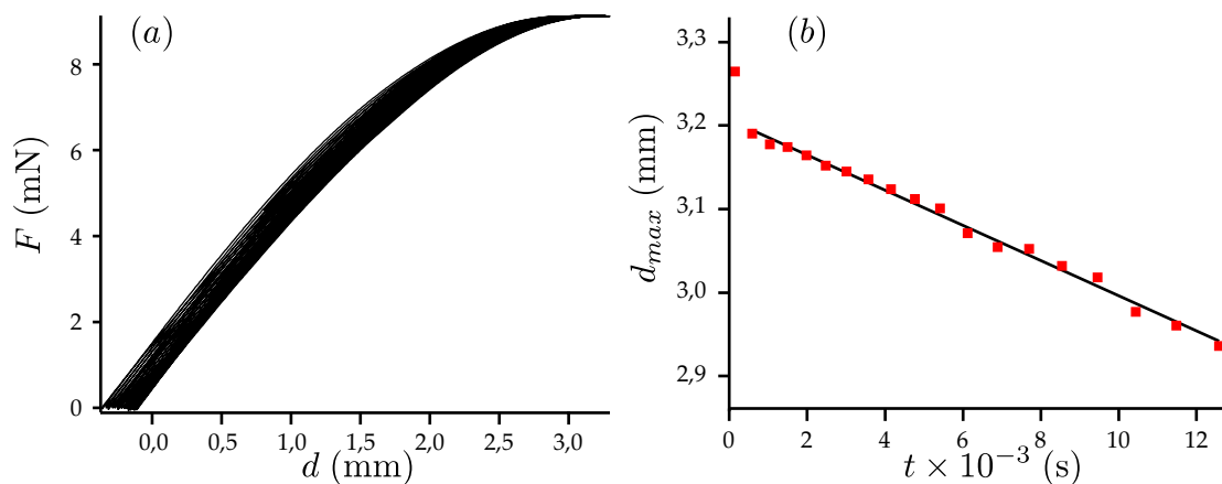
FIGURE A.3 (a) Force mesurée par le tensiomètre en fonction du déplacement vertical du plateau pour de multiples allers-retours du plateau dans le temps. On observe un maximum vers d_{max} \approx 3 mm. La largeur observée dans le sens horizontal est due à l'évaporation, qui fait baisser le niveau du bain. (b) Représentation de l'évaporation pendant les 3h20min de l'expérience. Le niveau où la force atteint son maximum d_{max} baisse régulièrement dans le temps au taux de 21 \text{ nm s}^{-1} .
