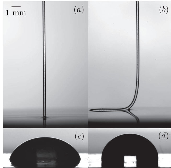
FIGURE 4.20 (a,b) Images d'un capillaire d'élastomère, décrit à la section 4.2, de diamètre 300 \mu\text{m} et de densité 1,02 \times 10^3 \text{ kg m}^{-3} , amené en contact avec un mélange eau/éthanol. De (a) à (b), l'angle de contact est augmenté continûment en abaissant la concentration en éthanol. La capillaire subit une déformation au dessus d'un angle critique. (c,d) Détermination indépendante de l'angle de contact en utilisant les mêmes mélanges que dans (a) et (b) et le même élastomère dans une géométrie plane. À gauche, l'angle de contact en avancée est de 60^\circ avec une solution à 50% en volume d'éthanol (de tension de surface \gamma = 29 \text{ mN m}^{-1} ). À droite, l'angle d'avancée est de 95^\circ pour une solution à 5% d'éthanol dans l'eau (de tension de surface \gamma = 55 \text{ mN m}^{-1} ).
