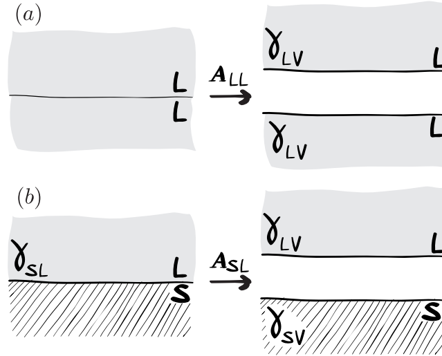
FIGURE 1.15 Relation entre le travail d'adhésion et les tensions de surface. (a) Pour séparer en deux un volume de liquide, il faut créer deux interfaces liquide-vapeur. Le coût énergétique est donc de A_{LL} = 2\gamma_{LV} . (b) Pour créer une interface liquide-solide, il faut d'abord créer une interface liquide-vapeur, et une interface solide-vapeur, ce qui coûte une énergie \gamma_{SV} + \gamma_{LV} . En regroupant ces deux interfaces, on réduit le coût de création des deux interfaces originales A_{SL} = \gamma_{SV} + \gamma_{LV} - \gamma_{SL} grâce aux interactions liquide-solide.
