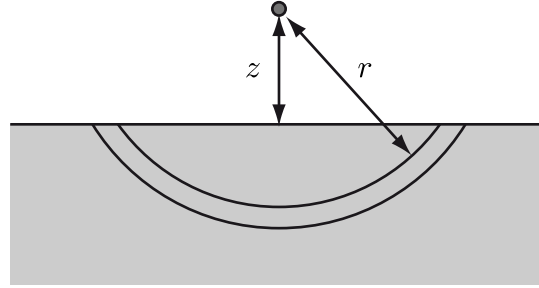
FIGURE D.1 Interaction entre un point et un demi-espace infini. L'intégration se fait soit par des coquilles de rayon r si on utilise l'interaction entre deux points, soit par des portions de cylindres de rayon r si on utilise l'interaction entre un point et une ligne infinie, perpendiculaire au plan du schéma.
