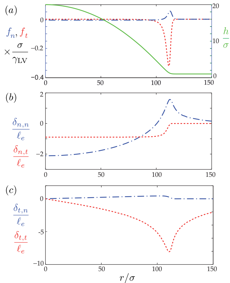
FIGURE 4.33 (a) Rappel de la distribution des forces de la Figure 4.32. Le profil radial de la goutte est en vert, les forces tangentielles en rouge (en négatif cette fois-ci car le centre de la goutte est en r = 0 ), les forces normales en bleu. (b) Déplacement normal de la surface du solide induit par ces forces : en rouge tangentielles, en bleu normales. (c) Déplacement tangentiel de la surface du solide induit par ces forces : en rouge tangentielles, en bleu normales. L'existence des termes croisés (déplacement normal induit par les forces tangentielles et inversement) provient du fait que le substrat possède pour ce calcul un module d'Young \nu = 0,35 . S'il était incompressible ( \nu = 1/2 ), ces déplacements seraient nuls.
