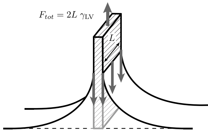
FIGURE A.1 Résultante des forces capillaire exercées par le liquide sur une plaque de platine.
