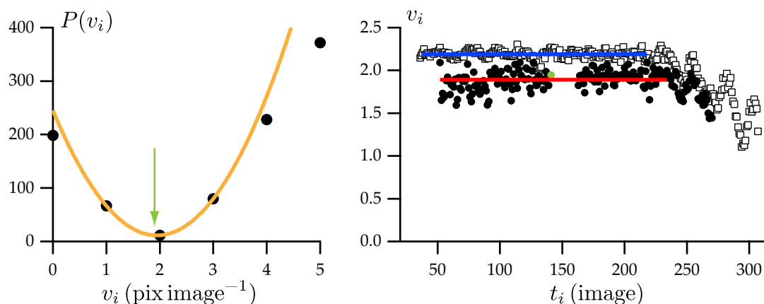
FIGURE 5.12 Mesure de la vitesse de la ligne de contact et du wafer . (a) Calcul de la corrélation P(v) (5.29) entre trois images successives de la séquence pour un point sur la ligne de contact [en vert sur (b)]. v_i représente donc le décalage vertical en pixels entre deux images successives. Un ajustement par une parabole proche du minimum donne la vitesse la plus probable, ici v = 1,95 \text{ pix image}^{-1} . Le minimum est presque à zéro, ce qui indique que la corrélation est fiable. (b) Vitesse le long des lignes détectées sur la Figure 5.11. On retient la moyenne de ces vitesses, avant que le wafer freine. On trouve ici la vitesse de la plaque en bleu U_p = 2,19 \text{ pix image}^{-1} et U_c = 1,89 \text{ pix image}^{-1} , soit U_p = 44,7 \text{ cm s}^{-1} et U_c = 38,6 \text{ pix image}^{-1} .
