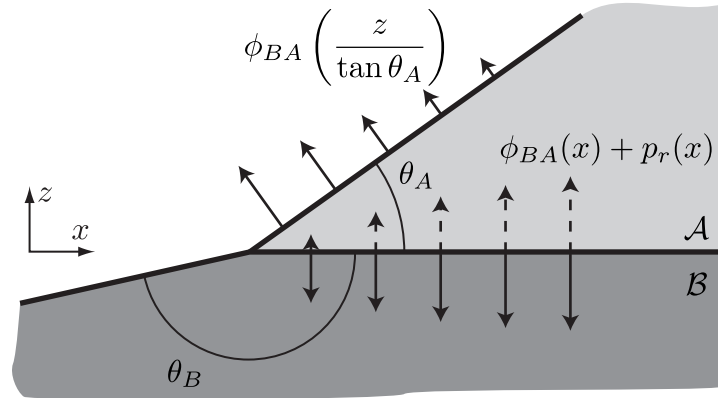
FIGURE 2.28 Schéma du calcul de la force exercée par un coin de liquide \mathcal{B} d'angle d'équilibre \theta_B sur un autre coin de liquide \mathcal{A} d'angle d'équilibre \theta_A au voisinage de la ligne de contact. D'après l'équation (2.73), la force se réduit au calcul des potentiels sur les interfaces de \mathcal{A} : l'interface \mathcal{S}_A entre \mathcal{A} et la vapeur, et l'interface \mathcal{S}_{AB} entre \mathcal{A} et \mathcal{B} . Sur \mathcal{S}_A , le potentiel est \phi_{BA}(z) , donné par l'équation (2.74). Sur l'interface \mathcal{S}_{AB} , le potentiel est \phi_{BA}(x) et est compensé par la répulsion p_r(x) , la somme étant donnée à l'équation (2.79). La force totale à l'équilibre est au final -\gamma_B \sin \theta_B selon z , et \gamma_B(1 + \cos \theta_B) selon x . Ce schéma ne représente pas la distribution des forces.
