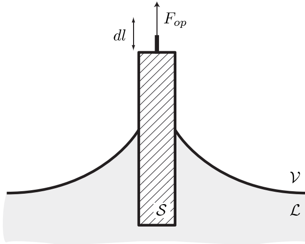
FIGURE 2.3 Translation dl d'une plaque plongée dans un bain. Lors de la translation, la surface mouillée de la plaque est remplacée par de la surface sèche. Le travail de l'opérateur est égal à l'énergie gagnée par le système, ce qui nous permet d'exprimer la force F_{op} = \gamma_{LV} \cos \theta_Y (2.13) par unité de longueur de ligne de contact.
