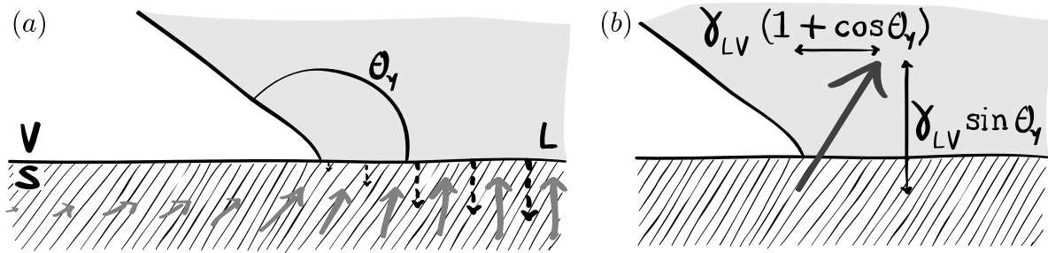
FIGURE 2.18 Forces agissant sur le solide (zone hachurée) par le liquide (zone grise) au voisinage de la ligne de contact. (a) Distribution des forces agissant sur le solide. À cause de l'attraction longue portée du liquide, le solide est attiré vers le liquide (flèches grises pleines). À mesure que l'on s'éloigne de la ligne de contact, la répulsion dans le liquide augmente (flèches noires en pointillés), et vient compenser l'attraction loin de la ligne de contact. L'absence de liquide dans une zone à gauche de la ligne de contact nous garantit le fait que la force tangentielle est toujours orientée vers la droite, même pour \theta_Y > 90^\circ . (b) Forces résultantes de cette distribution dans le solide : la force normale à l'interface est \gamma_{LV} \sin \theta_Y , et la force tangentielle est \gamma_{LV} + \gamma_{SV} - \gamma_{SL} = \gamma_{LV}(1 + \cos \theta_Y) .
