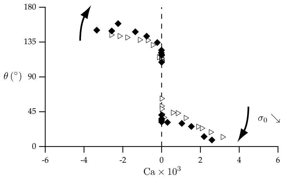
FIGURE 4.40 Angle apparent \theta en fonction du nombre capillaire pour un substrat en étirement ( \blacktriangleright ) en comparaison avec le même substrat non étiré ( \blacklozenge ), de module d'Young E = 15 kPa, et d'épaisseur initiale h = 2,1 mm.
