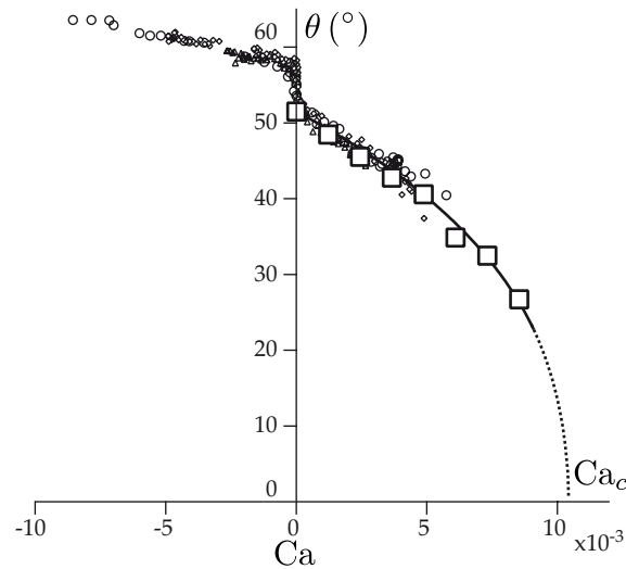
FIGURE 5.3 Angle de contact dynamique apparent en fonction du nombre capillaire pour des huiles silicone de PDMS sur des substrats fluorés. La figure et les données expérimentales en (□) sont issues de [203] et en (○, △, ◇) de [201]. La vitesse est positive lorsque le liquide recule sur le solide. La ligne représente une solution numérique donnée par un modèle hydrodynamique complet (5.23). Ca_c désigne le nombre capillaire critique auquel on attend la transition de mouillage dynamique par extrapolation en pointillés de la courbe numérique.
