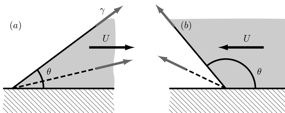
FIGURE 5.6 (a) Transition de mouillage dynamique. Lorsque l'angle baisse, la force maximale est atteinte pour \theta = 0 pour laquelle la dissipation dans le coin est maximale. (b) Transition de démouillage dynamique. Lorsque l'angle tend vers \pi et au contraire, la dissipation ne diverge pas. Rien ne retient alors le mouvement de la ligne de contact, il ne devrait donc pas exister de transition de démouillage.
