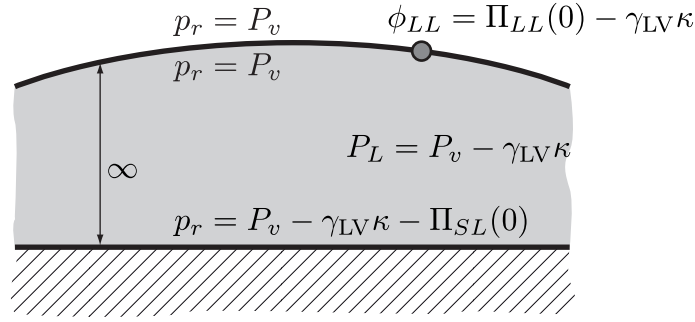
FIGURE 1.26 Répulsion p_r dans un film macroscopique de liquide, dont l'interface liquide-vapeur possède la courbure \kappa (négative sur ce schéma). Le potentiel attractif à la surface est \phi_{LL} et est donc moins négatif (attractif) que \Pi_{LL}(0) . Le potentiel thermodynamique P_L correspond lui à la pression de Laplace P_v - \gamma_{LV}\kappa . La surpression à l'intérieur de la goutte est bien positive dans ce cas.
