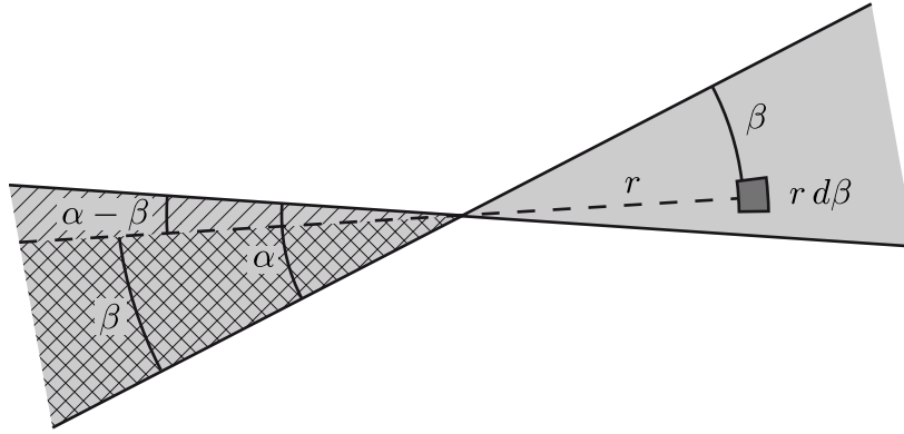
FIGURE D.3 Schéma de l'intégration de l'interaction entre deux dièdre opposés de même angle \alpha . On se ramène au calcul d'un point avec un dièdre aligné \Pi^{PD}(r, \alpha) donné à la Figure D.2.
