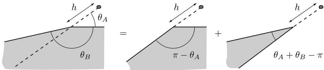
FIGURE 2.29 Décomposition de l'interaction \phi(h, \theta_A, \theta_B) exercée par un dièdre d'angle \theta_B > 0 sur un point à la distance h du coin, et faisant un angle \theta_A > 0 tel qu'indiqué. D'après cette construction, on trouve : \phi(h) = \Pi^{PD}(h, \pi - \theta_A) + \Pi^{PD}(h, \theta_A + \theta_B - \pi) .
