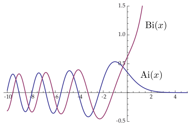
FIGURE D.4 Fonctions d'Airy Ai(x) et Bi(x) .
