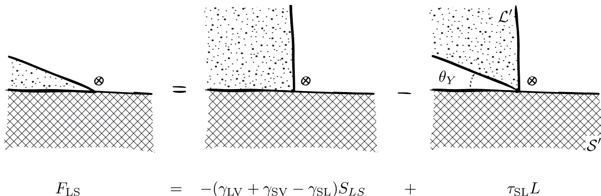
FIGURE 3.8 Domaines d'intégration de l'énergie libre pour l'interaction solide-liquide. Ce domaine peut être décomposé en une contribution proportionnelle à la surface de l'interface liquide-solide, ainsi qu'une contribution proportionnelle à la longueur de la ligne de contact. La région tachetée représente le domaine \mathcal{L}' dans l'équation (3.27) et la région hachurée correspond à \mathcal{S}' . Le terme surfacique correspond à -(\gamma_{LV} + \gamma_{SV} - \gamma_{SL})S_{LS} et le terme linéique à \tau_{SL}L .
