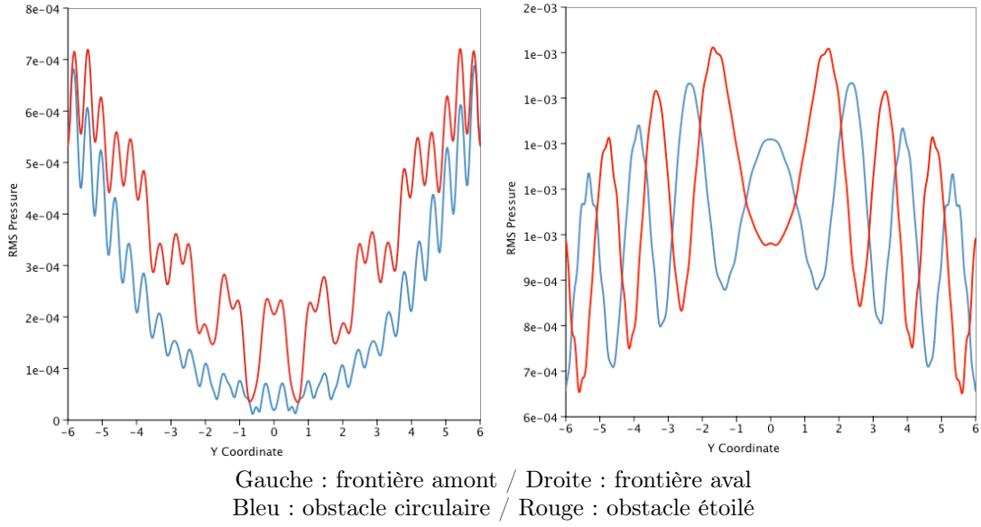
FIGURE 5.13 – Coupes 1D de la pression RMS le long des frontières amont et aval du domaine DF
