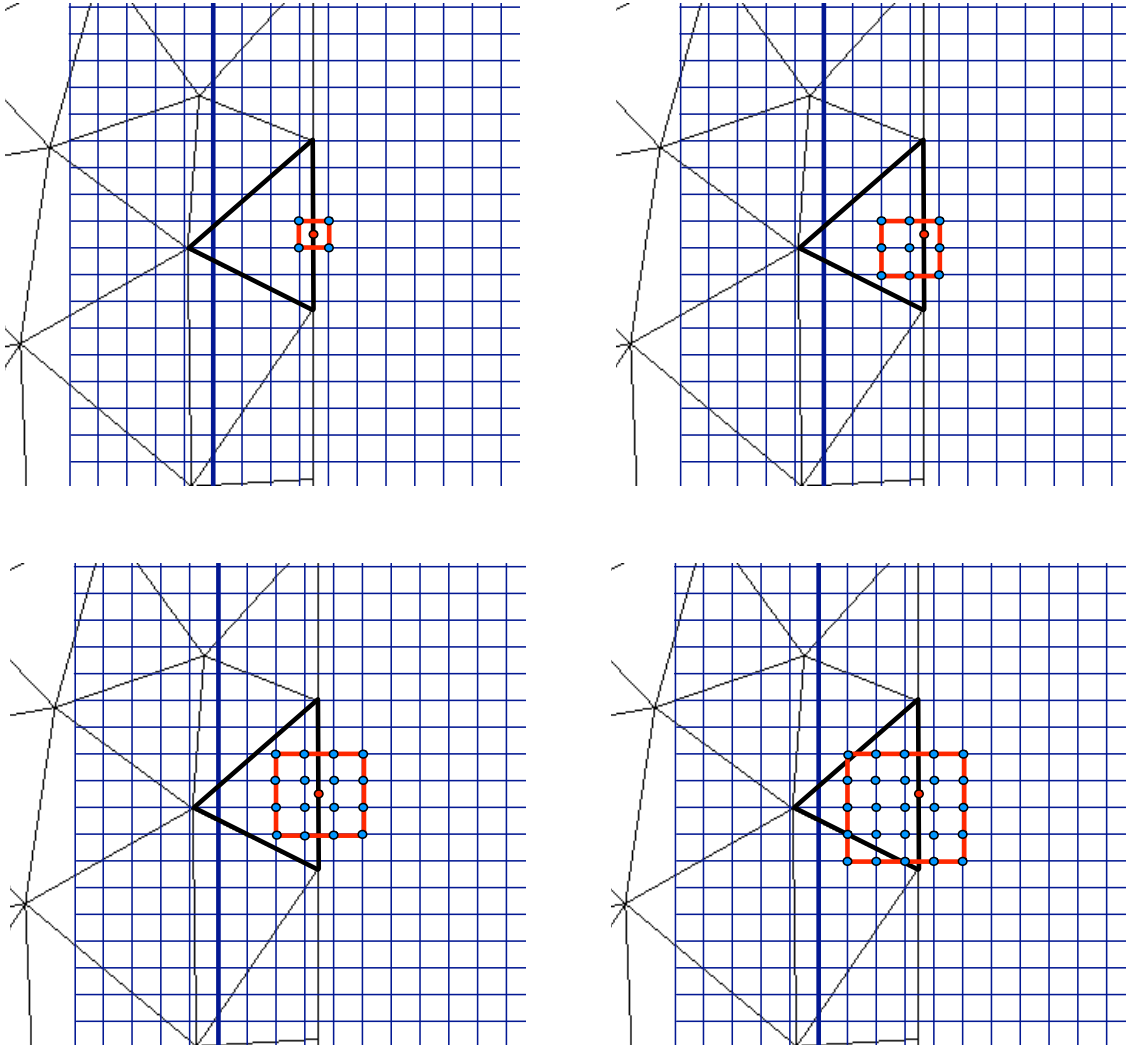
Degré de liberté Lagrangien DG ( \gamma_{(k)} ) \rightarrow \bullet \bullet \leftarrow Stencil d'interpolation
