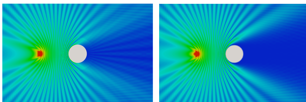
Champ de densité RMS, 0 < \rho_1^{\text{RMS}} < 5 \cdot 10^{-3}
