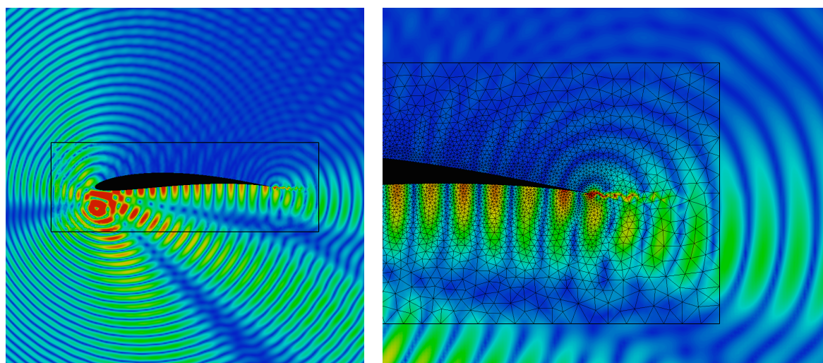
Norme euclidienne du vecteur vitesse acoustique, 0 < |\mathbf{v}_1| < 2 \times 10^{-3}
