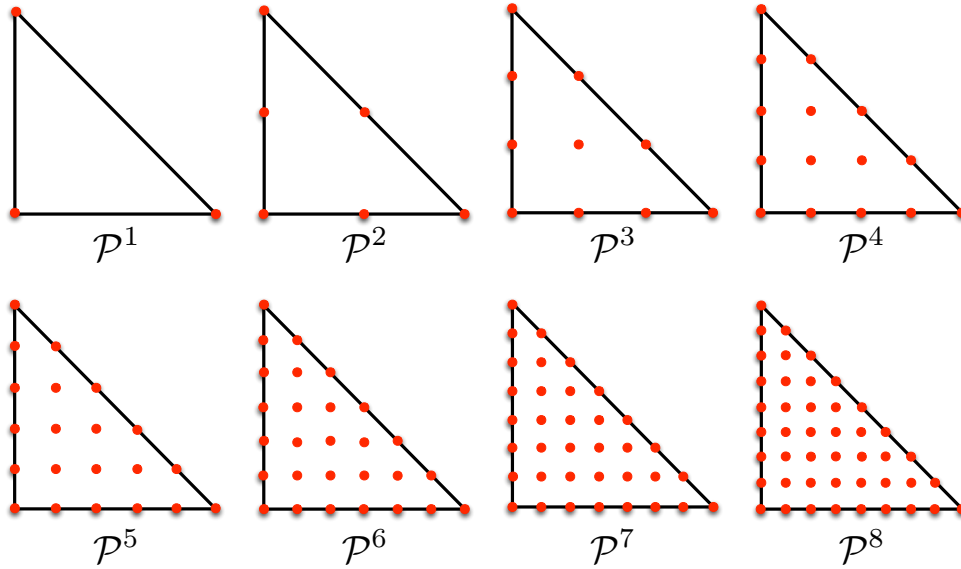
FIGURE 2.7 – Représentation des degrés de liberté dans le triangle unité muni de fonctions de bases Lagrangiennes d'ordre 1 à 8.
