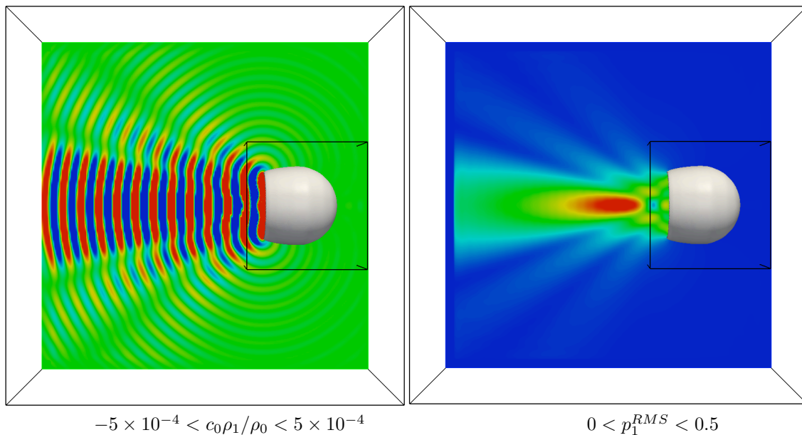
Gauche : champ de pression instantané couplé Droite : champ de pression RMS couplé
