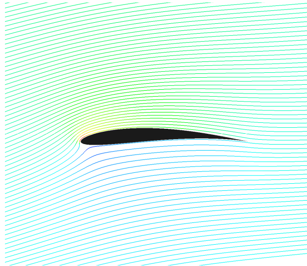
Lignes de courant colorées par la norme euclidienne du vecteur vitesse
