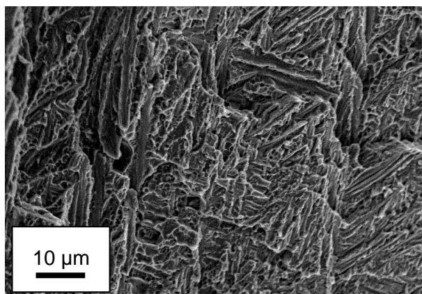
Figure 24 : Evolution du mécanisme de rupture à température ambiante en fonction de la teneur locale en oxygène, pour la couche ex-β des gaines en Zy-4 oxydées et trempées à l'eau à température ambiante.
