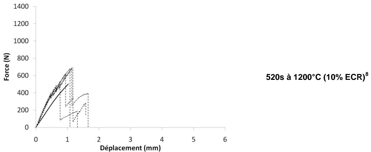
Figure 59 : Courbes de force-déplacement obtenues par RCT sur les gaines sablées (en lignes continues) et sur gaines intégrès (en pointillés).
