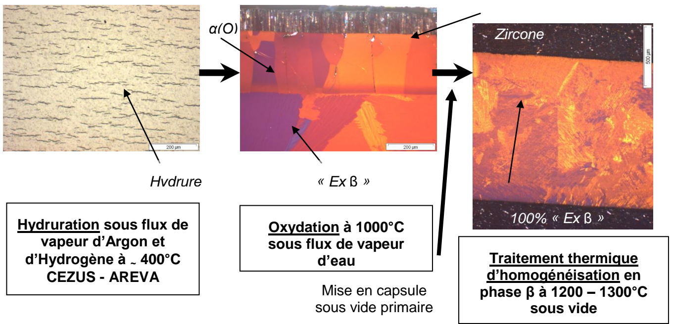
Figure 98 : Illustration du protocole de préparation de « matériaux modèles » - Observation de la microstructure à chaque étape.
