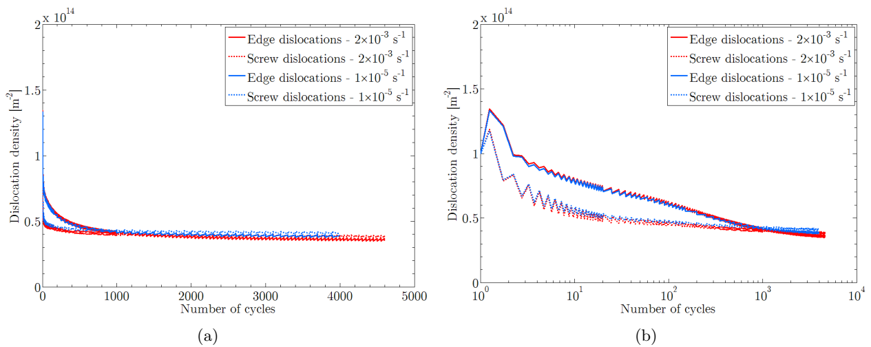
Fig. 5.6. Prédiction des évolutions des densités de dislocations mobiles coin et vis au cours du chargement cyclique pour une amplitude de déformation de \pm 0.35\% et deux vitesses de déformation (a) en échelle linéaire et (b) en échelle logarithmique. Modèle tenant compte de la distribution initiale de taille de sous-grains.
