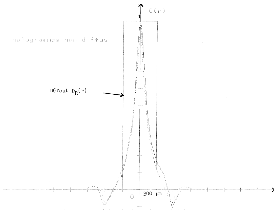
Figure 66. Traitement d'un disque de rayon R = 300 \mu\text{m} représentant le défaut D_R seul, par pseudo-filtrage de Wiener de paramètre de bruit \epsilon = 0,1 : réponse percussive globale après traitement G(r) (en traits pleins : courbe expérimentale, en pointillés : courbe théorique).
