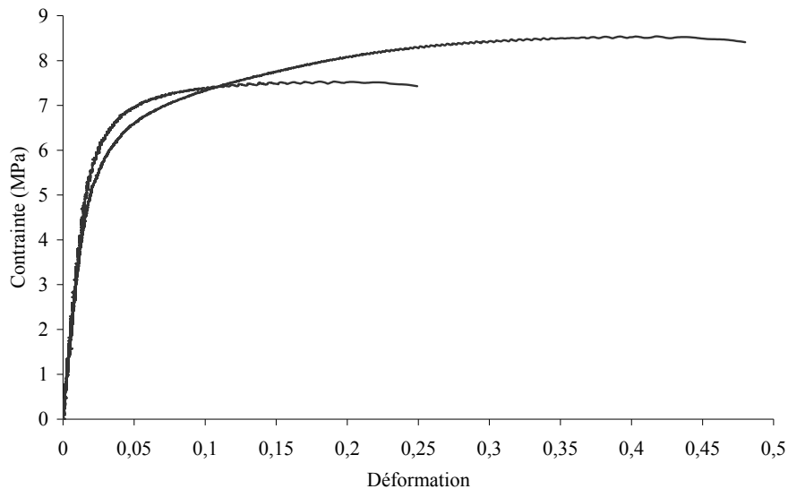
Figure 2.51 Comportement en traction (0°) à 7 N.s -1 , 2 spécimens - colle XPU
