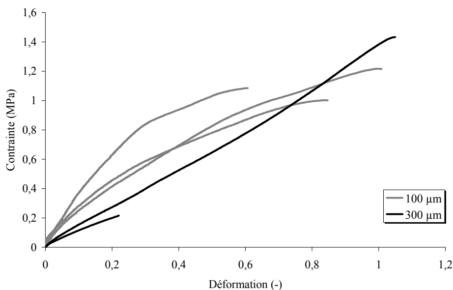
Figure 2.55 Comportement en cisaillement ( 90^\circ ) à 7 \text{ N}\cdot\text{s}^{-1} , 3 spécimens à 100 \mu\text{m} , 2 spécimens à 300 \mu\text{m} - colle FMV
