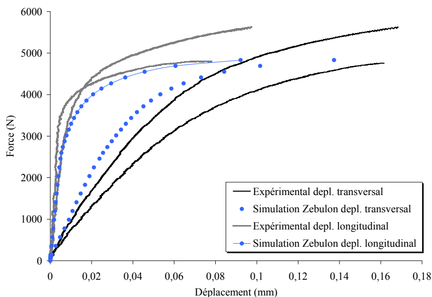
Figure 3.17 Simulation des essais Arcan-Mines à 30^\circ - colle XPU
