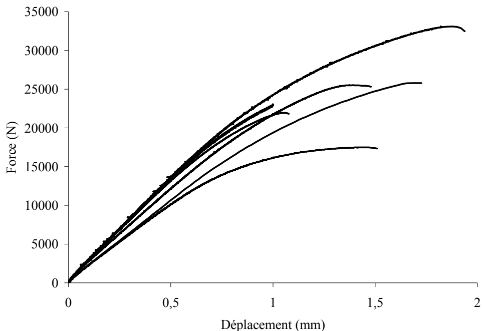
Figure 2.61 Courbe force-déplacement entre substrats centraux à 1 \text{ N}\cdot\text{s}^{-1} , 7 spécimens – colle XPU
