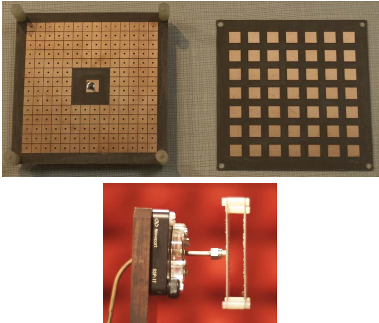
Figure R15 – Antenne Fabry-Pérot avec antenne patch carré : patch et HIS, FSS, puis antenne assemblée.
