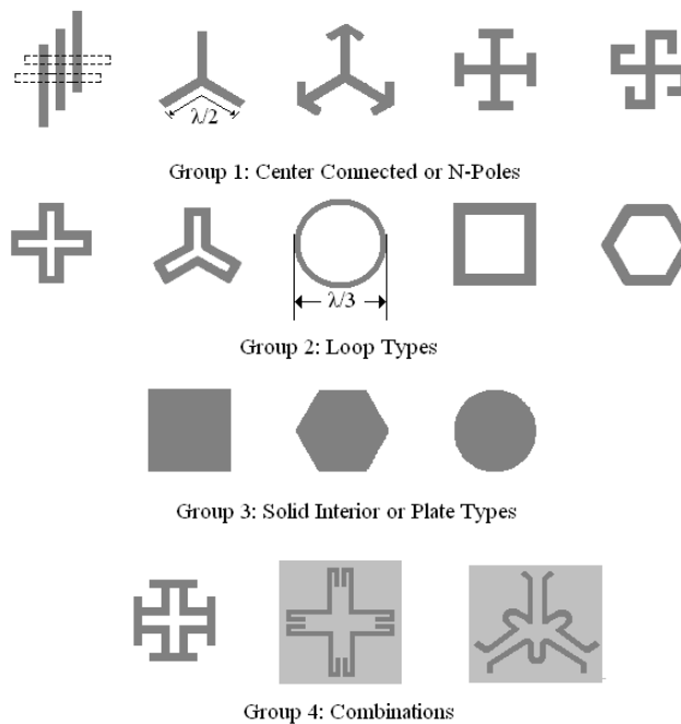
Figure R4 – Les quatre grands groupes d'éléments des FSS. Les éléments sont classés de faibles bandes passantes sur la gauche à grandes bandes passantes sur la droite [25].
