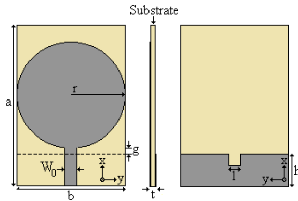
Figure R5 – Géométrie de l'antenne monopole circulaire imprimé avec encoche.
