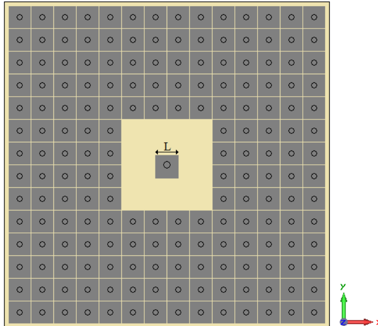
Figure R10 – Géométrie de l'antenne patch carré associée à une surface haute impédance.
