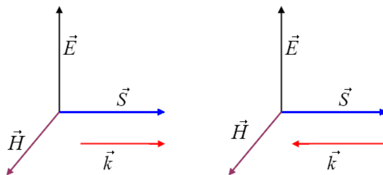
Figure R2 – Schéma montrant les vecteurs de Poynting d'une onde électromagnétique. A gauche, les matériaux classiques et à droite les métamatériaux.
