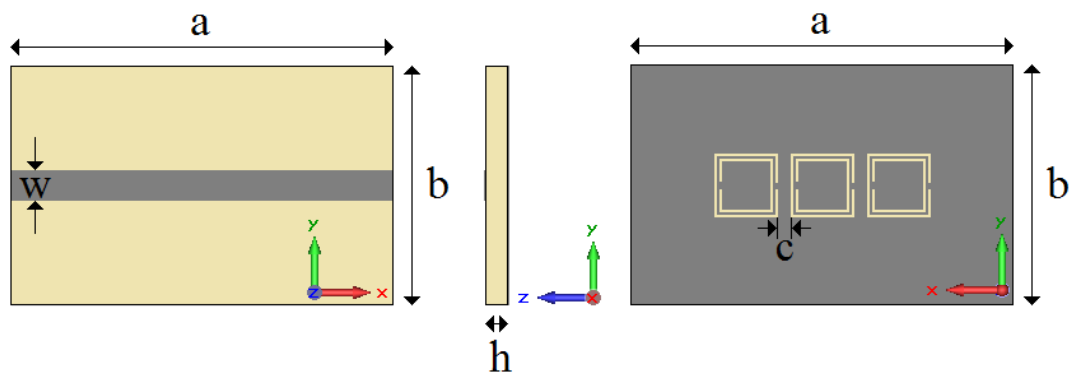
Figure R8 – Géométrie du filtre utilisant trois cellules CSRR gravées dans le plan de masse.
