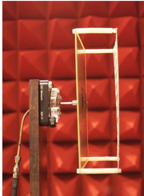
Figure R16 – Antenne Fabry-Pérot avec antenne à fente en U : antenne à fente en U et HIS, FSS, puis antenne assemblée.
