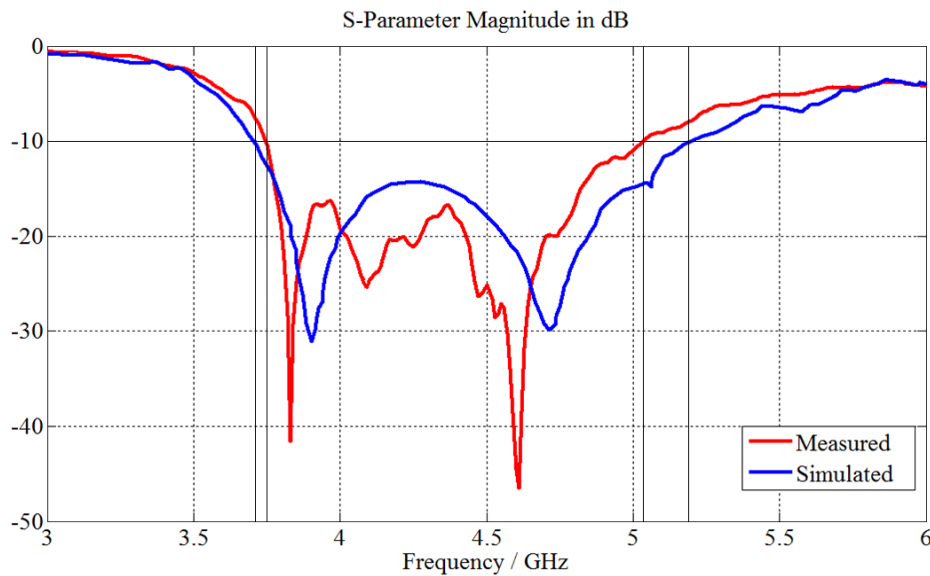
Figure R13 – Adaptation de l'antenne rectangulaire à fente en U associée à une surface haute impédance (simulation en bleu et mesure en rouge)
