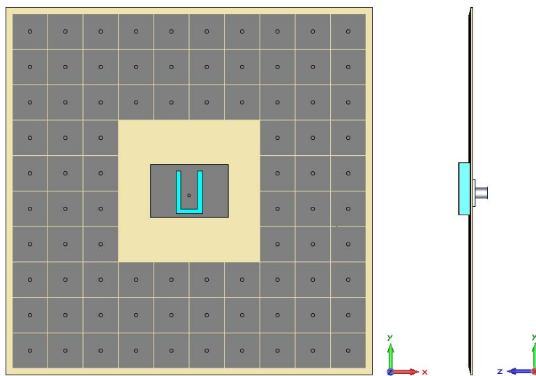
Figure R12 – Géométrie de l’antenne rectangulaire à fente en U associée à une surface haute impédance.
