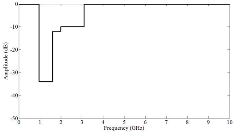
Fig. 4.17 – FCC mask.
