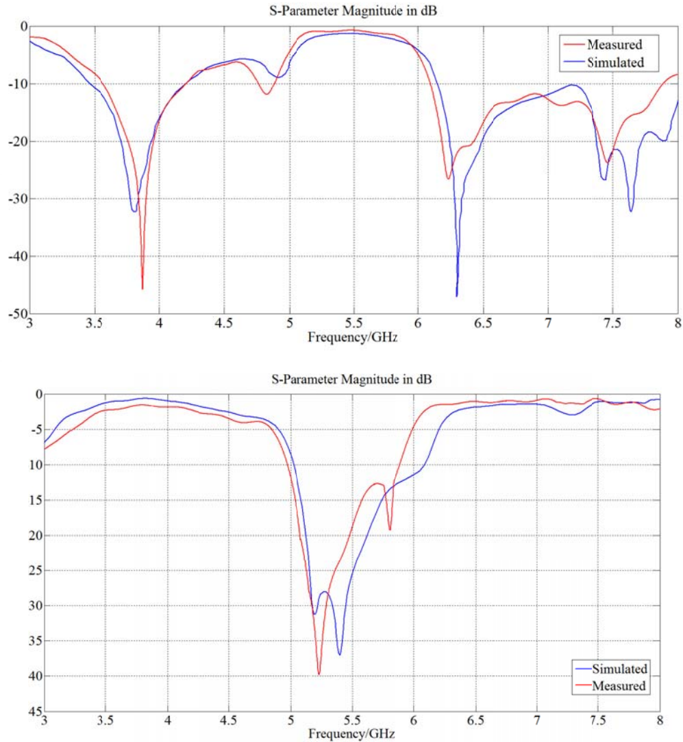
Figure R9 – Modules des paramètres S11 (a) et S21 (b) du filtre à 3 cellules CSRR gravées dans le plan de masse d'une ligne microruban (simulation en bleu et mesure en rouge).
