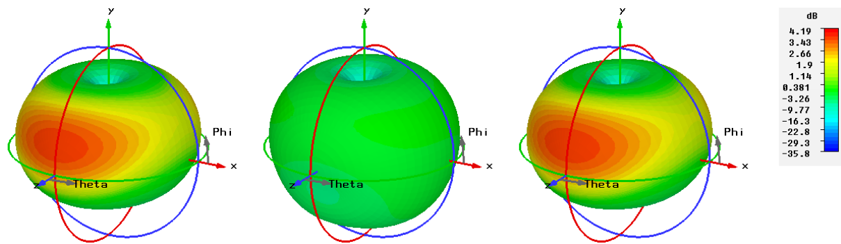
Figure R7 – Diagrammes de rayonnement 3D en gain réalisé de l’antenne monopole imprimé circulaire à 4 GHz, 5.9 GHz and 6.5 GHz.
