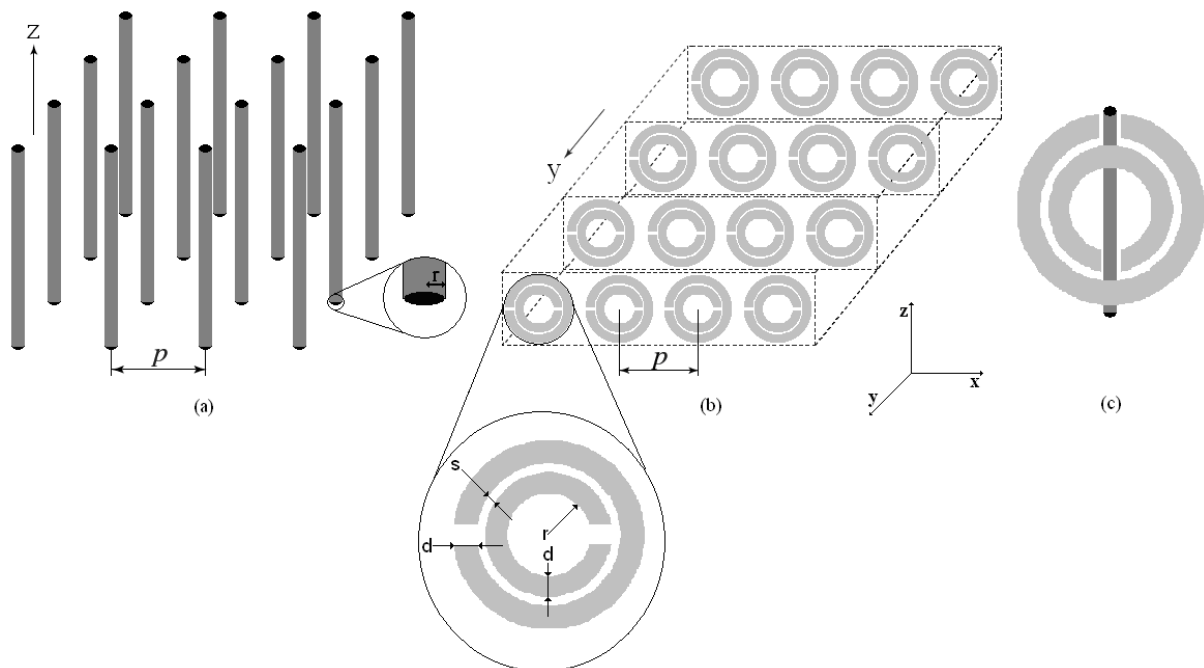
Figure R1 – Métamatériaux réalisés avec des diélectriques et des métaux: (a) permittivité négative et perméabilité positive, (b) permittivité négative et perméabilité positive, (c) permittivité négative et perméabilité négative DNG [15].
