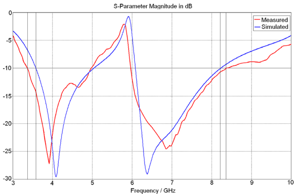
Figure R6 – Adaptation de l'antenne monopole imprimé circulaire, mesure (rouge) et simulation (bleue).
