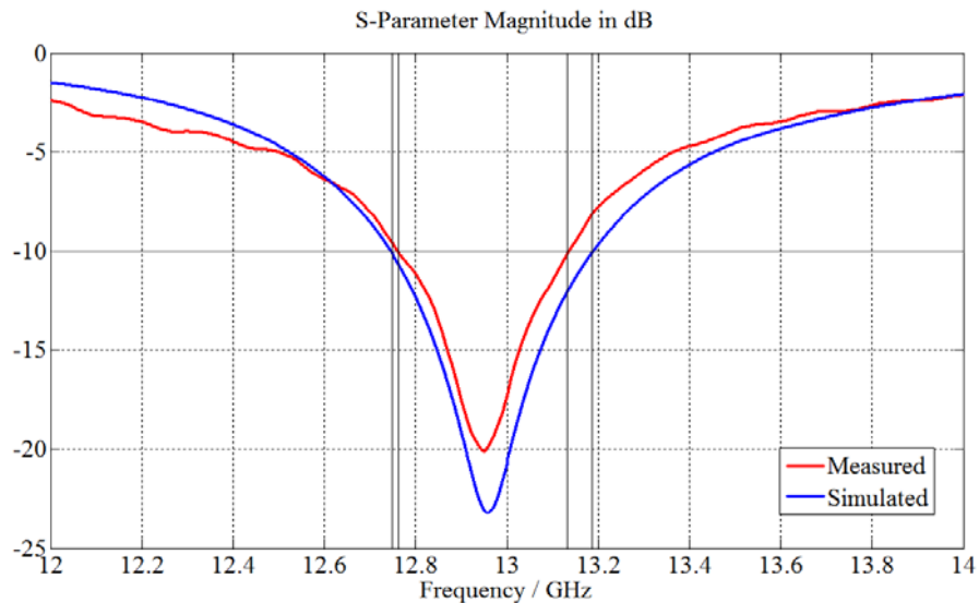
Figure R11 –Adaptation de l’antenne patch carré associée à une surface haute impédance (simulation en bleu et mesure en rouge)
