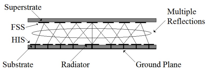
Figure R14 – Principe de l'antenne Fabry-Pérot
