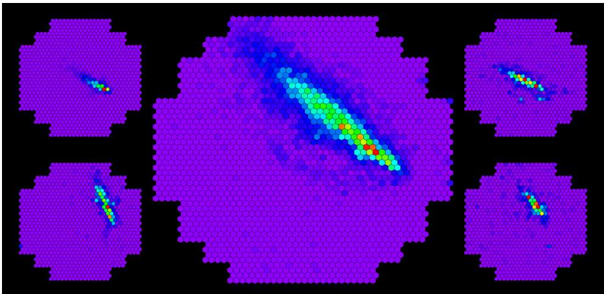
FIGURE 5.24 – Premiers événements enregistrés par le réseau de télescopes H.E.S.S. II. Au centre la caméra de CT5 et de part et d'autre les caméras des télescopes CT1 à CT4. Crédit : http://www.mpi-hd.mpg.de/hfm/HESS/ .
