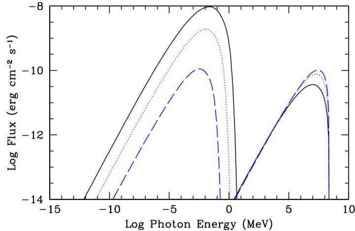
FIGURE 4.11 – Spectre d’émission caractéristique des PWN (à gauche le pic synchrotron et l’émission Compton inverse à droite) pour différents âges du PWN : 1000 ans (ligne continue), 2000 ans (pointillés rouges) et 5000 ans (tirets bleus). L’effet du choc retour du SNR sur le PWN a lieu après et n’est pas pris en compte ici. Figure issue de [Slane 2010b].
