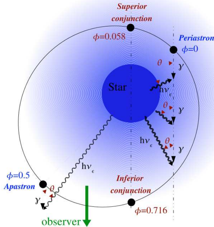
FIGURE 4.17 – Géométrie orbitale du système LS 5039 (figure tirée de [Aharonian 2006a]). Les configurations particulières (périastron, apastron, conjonctions inférieures et supérieures) sont représentées avec les phases orbitales \phi associées. L'absorption des rayons gamma au TeV par interaction avec les photons de l'étoile compagne et création de paires est plus importante lorsque l'objet compact est proche de l'étoile et que l'angle \theta est grand, donc au moment de la conjonction supérieure pour cette configuration [Dubus 2008].
