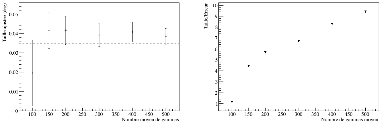
FIGURE 9.9 – Gauche : taille ajustée en fonction du nombre de gammas dans la source simulée pour une taille intrinsèque de 0.035^\circ (valeur représentée par la ligne pointillée rouge). Droite : significativité estimée (taille ajustée divisée par l'erreur correspondante) des tailles intrinsèques ajustées en fonction du nombre de gammas. Chaque point correspond encore ici aux valeurs ajustées d'une seule réalisation.
