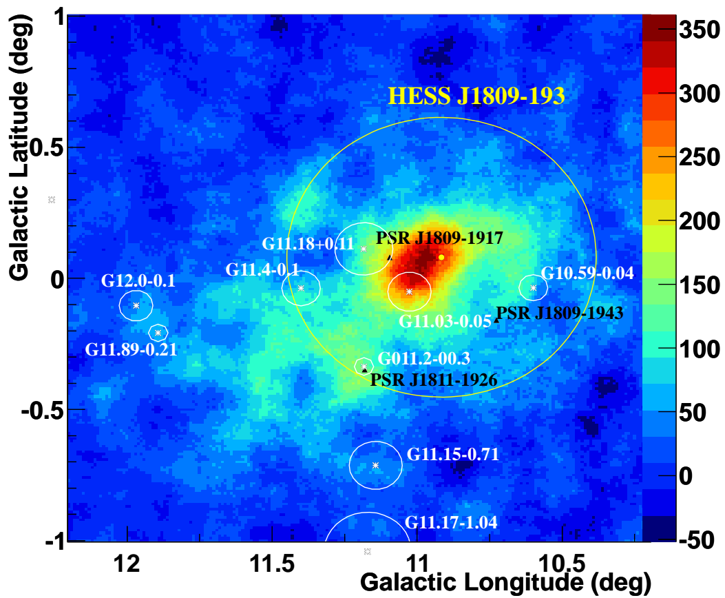
FIGURE 7.15 – Carte d'excès corrélée à 0.089^\circ de la source HESS J1809-193 avec différentes contreparties possibles présentes dans le champ de vue (SNRs du catalogue Green en rose et pulsars en rouge et noir).
