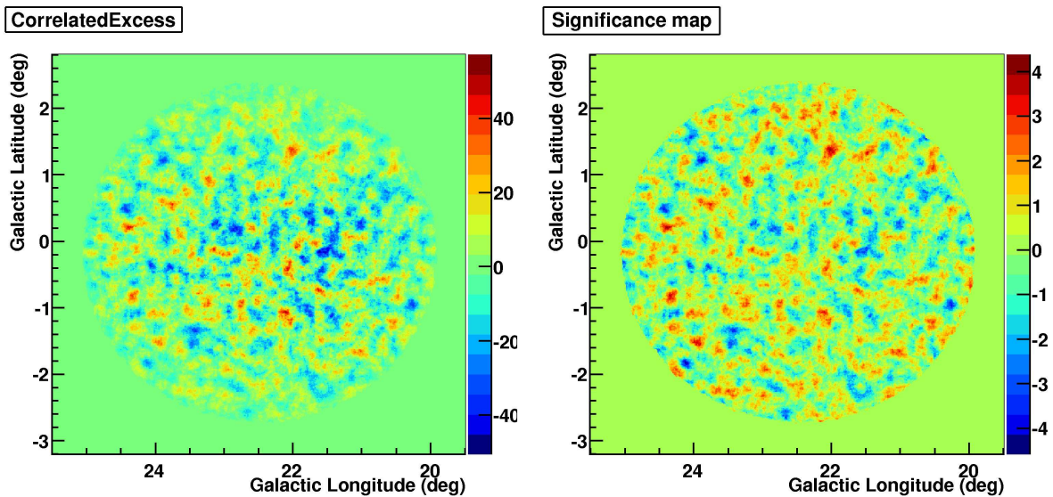
FIGURE 7.6 – Exemple de simulations de cartes d'excès et de significativité (corrélées avec un rayon = 0.089^\circ ) obtenues à partir des cartes ON et OFF de la figure 7.5.
