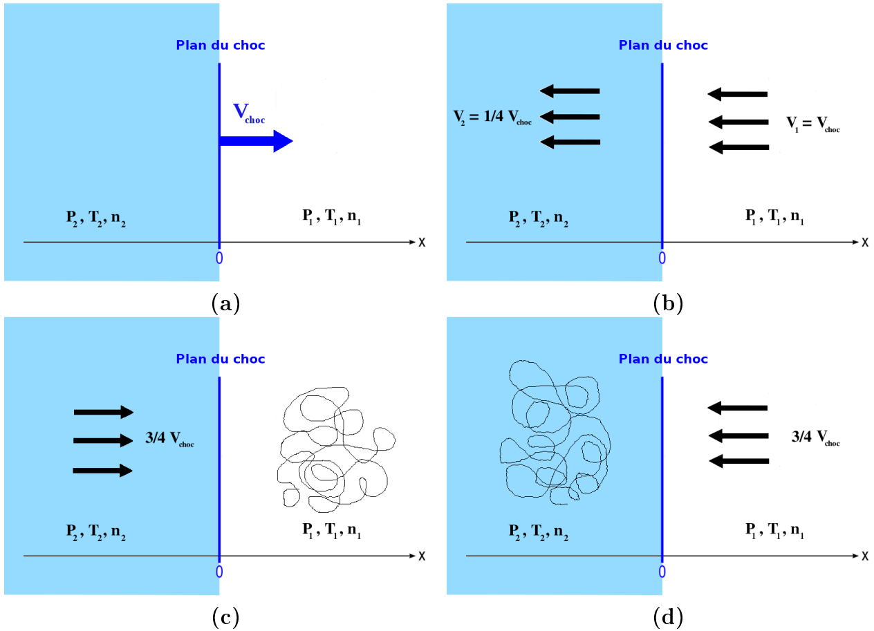
FIGURE 2.8 – Représentation d'un choc fort unilatéral et dynamique des particules accélérées dans chaque référentiel, dans le cas où l'indice adiabatique \gamma vaut 5/3 (gaz parfaits monoatomiques). Le milieu aval est représenté en bleu et le milieu amont en blanc. (a) : une onde de choc se propage à vitesse V_{choc} à travers le gaz interstellaire situé en amont du choc (en blanc), de densité n_1 , pression P_1 et température T_1 . En aval du choc (représenté en bleu clair), la densité, pression et température sont n_2 , P_2 et T_2 et sont reliées au milieu amont par les relations de Rankine-Hugoniot. Les vitesses sont données ici en norme. (b) : dans le référentiel du choc (où le choc est immobile), la vitesse des particules en amont est V_1 = V_{choc} . Le rapport des vitesses est égal au taux de compression (qui vaut 4 pour un gaz parfait), on a donc V_2 = V_1/r = V_{choc}/4 . (c) : dans le référentiel amont où le gaz interstellaire est stationnaire, les particules voient le choc arriver à une vitesse de 3/4 V_{choc} . (d) : inversement, dans le référentiel aval les particules voient le gaz interstellaire arriver vers elles à une vitesse de 3/4 V_{choc} également.
