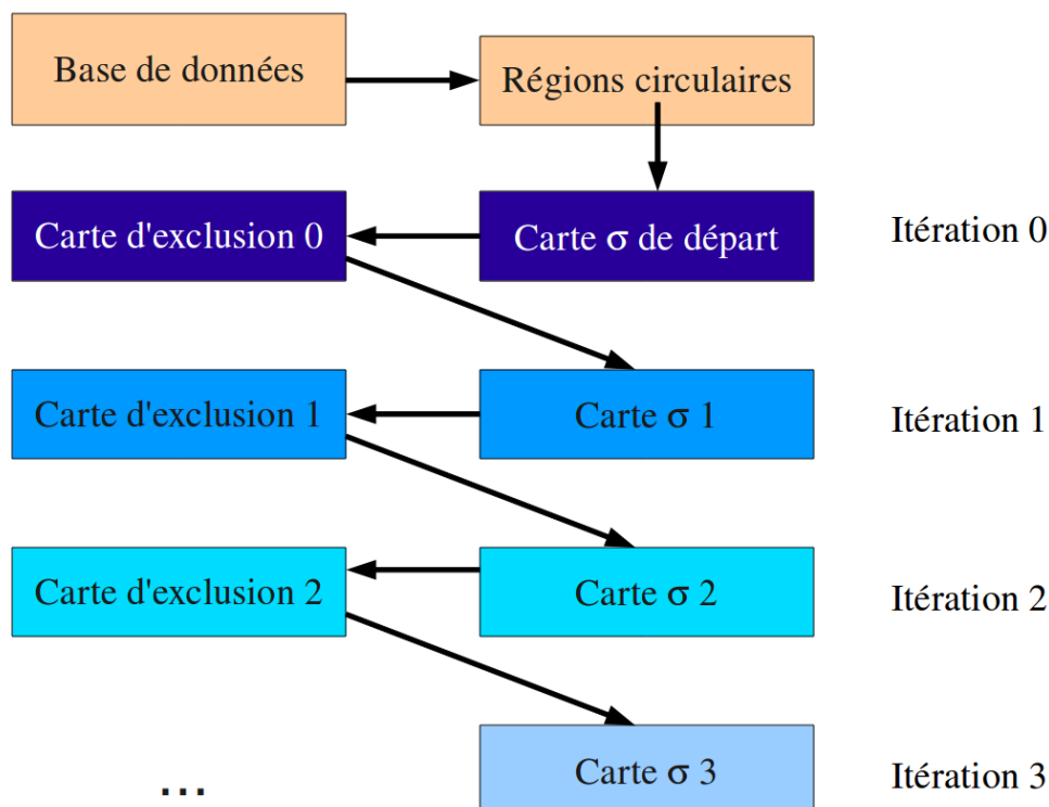
FIGURE 7.10 – Représentation schématique de la procédure des itérations successives. Les régions circulaires sont issues de la base de données collective et utilisées pour créer la carte de significativité de départ (itération 0). La carte d'exclusion personnalisée numéro 0 est produite à partir de cette carte et sera utilisée pour créer la carte de significativité à l'itération 1, etc.
