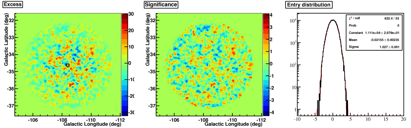
FIGURE 7.9 – Gauche : carte d’excès corrélé avec un rayon de 0.089^\circ du champ de vue de la galaxie Pictor A obtenue avec la configuration teak . La position et taille de la région ON utilisée est symbolisée par le cercle noir. Milieu : carte de significativité de ce champ de vue. Droite : Distribution de significativité correspondante et ajustement avec une fonction gaussienne.
