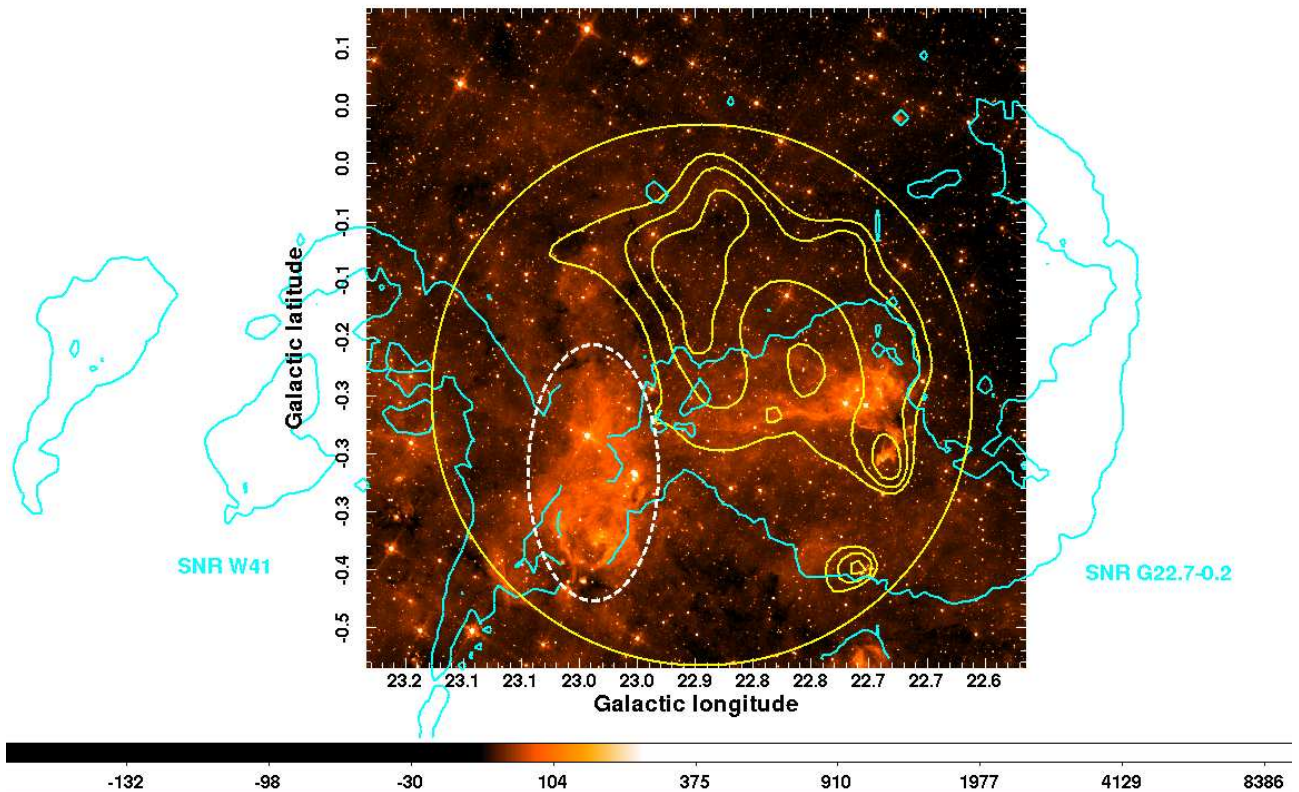
FIGURE 9.19 – Couleur : image infrarouge du satellite Spitzer à 5.8 \mu\text{m} autour de la position ( l=22.9^\circ , b=-0.2^\circ ) [Reach 2006]. Cyan : images des SNRs G22.7-0.2 et W41 à 1.4 GHz lors du MAGPIS [Helfand 2006]. Jaune : excès corrélé observé en rayons X par XMM-Newton entre 1 et 2 keV (ID : 06544802). Le cercle jaune correspond au champ de vue du satellite. La région d'interaction entre les deux SNRs vue par [Reach 2006] et indiquant la présence potentielle de nuages H_{II} compressés par les SNRs est entourée par l'ellipse en tirets blancs. La morphologie de l'émission diffuse en rayons X ne semble pas correspondre aux contreparties à d'autres longueurs d'onde. De plus, on n'observe pas d'émission X au niveau de la zone d'interaction IR.
