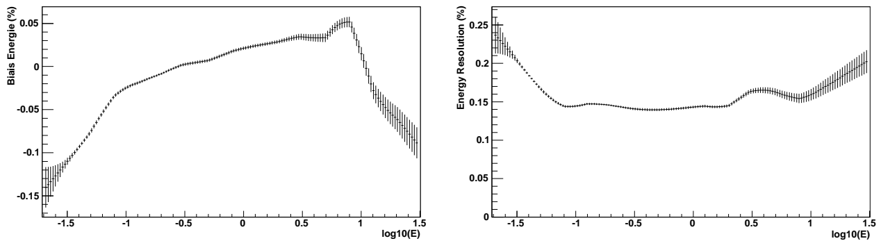
FIGURE 6.20 – Biais (à gauche) et résolution (à droite) en énergie obtenus avec la méthode Oak pour la configuration ash, à 70% d'efficacité optique, pour un angle zénithal de 18^\circ et un offset de 0.5^\circ .
