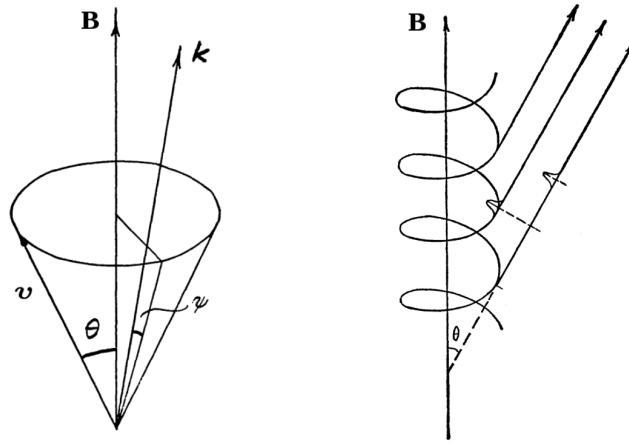
FIGURE 3.1 – Schématisation du cône de vitesse d'un électron se propageant le long d'une ligne de champ. L'angle \theta entre \vec{v} et \vec{B} reste constant. \vec{k} représente le vecteur d'onde. L'électron a une trajectoire hélicoïdale autour de la ligne de champ et émet des photons synchrotron à intervalles réguliers dans une direction donnée (à une fréquence \omega_g correspondant à sa vitesse angulaire) [Ginzburg 1965, Ginzburg 1969].
