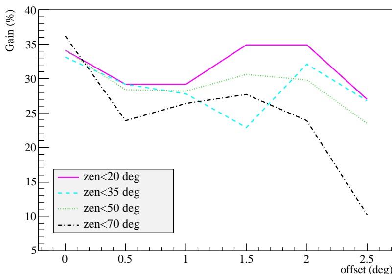
FIGURE 8.14 – Gain moyen par rapport à la reconstruction Hillas seule obtenu en choisissant systématiquement la meilleure méthode de reconstruction pour différentes bandes en angle zénithal ( zenith < 20^\circ , 35^\circ , 50^\circ et 70^\circ ).
