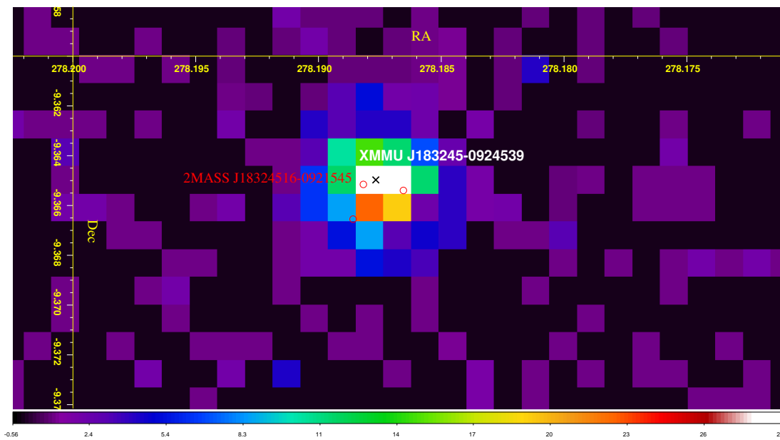
FIGURE 9.25 – Carte en coups non lissée de la source XMMU J183245-0921539. La croix noire correspond au centre gravité de la source X et les sources IR du catalogue 2MASS les plus proches sont représentées par les cercles rouges.
