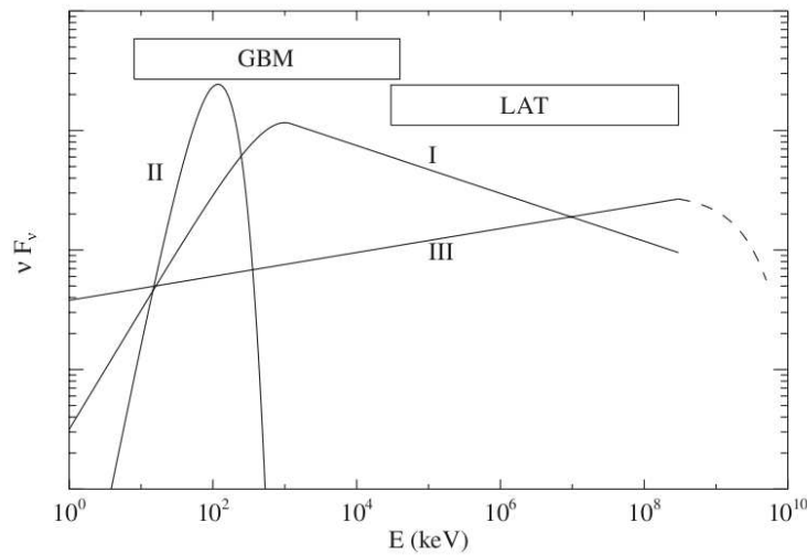
FIGURE 4.26 – Schématisation des trois composantes spectrales formant l'émission prompt de GRBs observés par Fermi [Zhang 2011]. I : composante non thermique, II : composante quasi-thermique, et III : composante supplémentaire en loi de puissance qui s'étend à plus haute énergie mais présenterait une coupure dans la gamme en énergie accessible par Fermi (environ 1 TeV).
