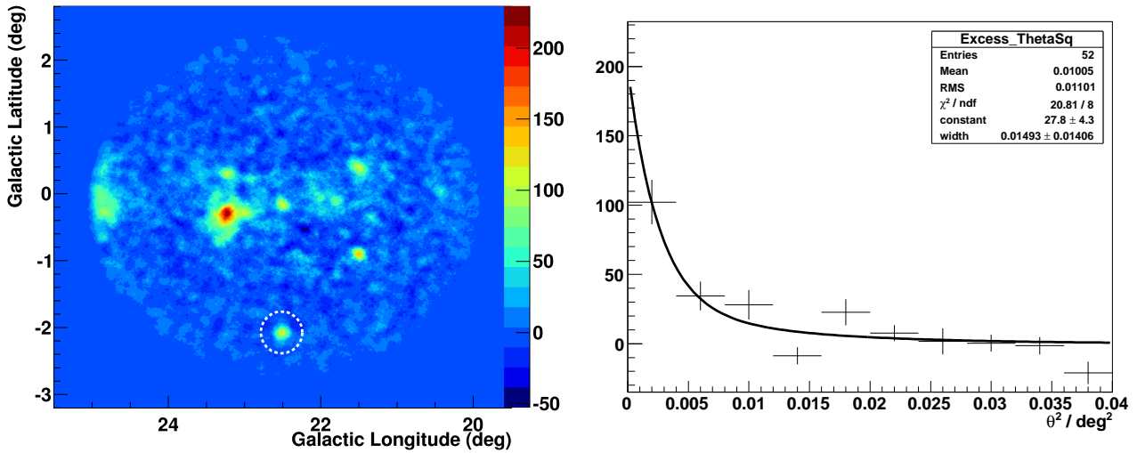
FIGURE 9.7 – A gauche : carte d'excès corrélé avec un rayon égal au r_{68} du champ de vue avec une source ponctuelle simulée repérée par le cercle pointillé. A droite : distribution en \theta^2 correspondante ajustée par la fonction F_{simu} . La largeur intrinsèque obtenue (width) est bien compatible avec une source ponctuelle.
