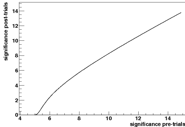
FIGURE 6.21 – Evolution de la significativité corrigée en fonction de \sigma_{pre-trials} pour un nombre d'essais égal à 8.4 \times 10^6 .
