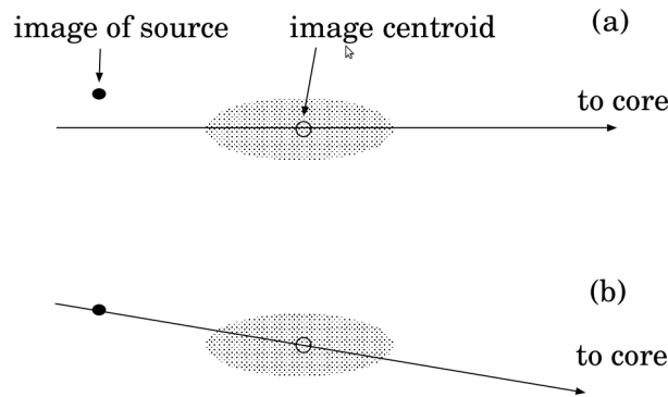
FIGURE 6.8 – (a) Reconstruction standard de la direction du gamma incident (b) Reconstruction basée sur l'hypothèse que le gamma provient de la direction de la source observée. Figure issue de [Hofmann 2000].
