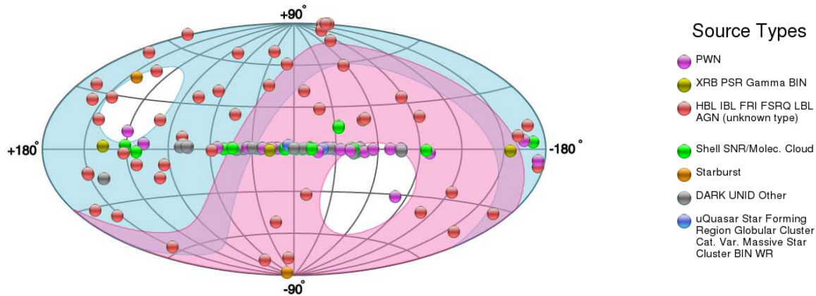
FIGURE 5.13 – Sources du catalogue TeVcat en coordonnées galactiques et visibilité accessibles par VERITAS/MAGIC (en bleu) ainsi que pour H.E.S.S. (en rose). Crédit : http://tevcatalog.uchicago.edu/ .
