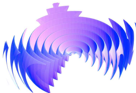
FIGURE 2.4 – Vue 3D de la structure des couches de courant pour un rotateur oblique. À la traversée d'une couche, le champ magnétique est inversé. Cette structure se propage radialement à une vitesse proche de la vitesse de la lumière. Figure issue de [Pétri 2007].
