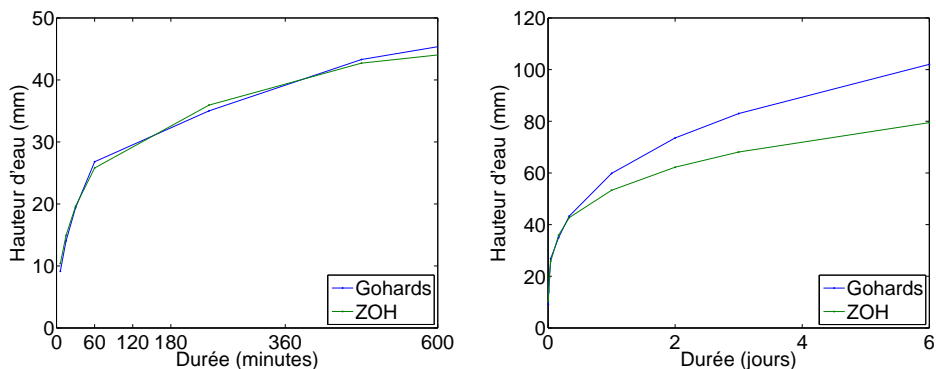
FIGURE 8.3.: Hauteur d'eau en fonction de la durée pour des pluies de période de retour T = 10 ans.
