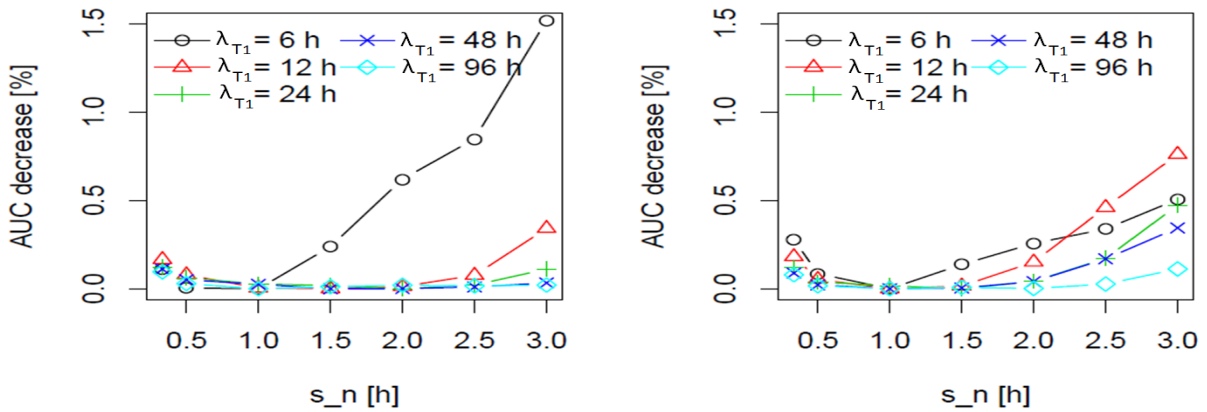
FIGURE 3.10 – Sensibilité des performances de détection au choix de s_n – Déclin des performances de détection vis-à-vis des performances optimales (i.e. AUC(s_n^*) ), pour les approches Gallego (à gauche), et Lindeberg (à droite), en fonction de la valeur de s_n . Les performances de l'approche Gallego, qui apparaissent moins sensibles à la valeur de s_n que les performances de l'approche Lindeberg, le sont plus dès lors que la durée moyenne inter-ruptures est petite (i.e. \lambda_{T_1} = 6 h, courbe noire). Les résultats présentés ici ont été obtenus pour un ratio c = 5 entre la durée moyenne d'un épisode de production nulle, et la durée moyenne d'un épisode de production élevée.
