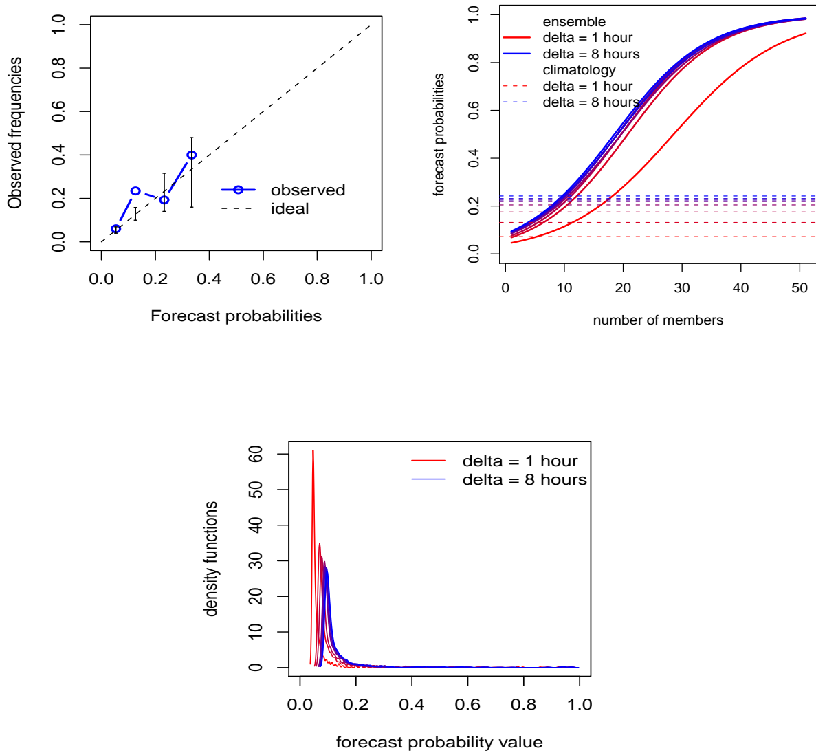
FIGURE A.6 – Diagramme de fiabilité (en haut à gauche), valeurs en fonction du nombre de membres m (en haut à droite), et distribution (en bas) des probabilités prédites p_{\delta,m} d'apparition d'une rupture dans les intervalles temporels I_{\delta} . Les résultats montrés ici ont été obtenus avec l'approche d'agrégation A2 , un seuil \hat{\tau} = 30\% P_n et un modèle de régression logistique.
