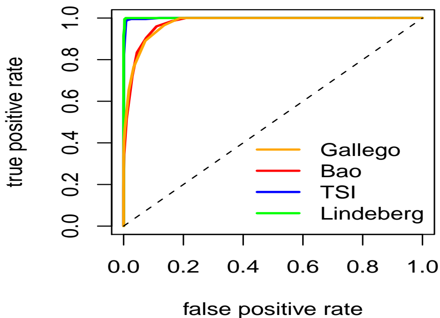
FIGURE 3.11 – Courbe ROC – Représentation du compromis existant entre les deux types d’erreur de classification des variations d’un signal pour les approches Bao, Gallego, TSI et Lindeberg. La proximité des courbes bleue et verte (superposées) avec le coin supérieur gauche de la figure montre l’aptitude des approches TSI et Lindeberg à classer parfaitement ou presque les variations d’un signal. Les résultats montrés ici ont été obtenus pour des valeurs de paramètres définissant des ruptures proches \lambda_{T_1} = 6 h et c = 5 , d’amplitude A = 50\% P_n et de durée moyenne \lambda_{T_2} = 3 h, et pour une forte intensité de bruit j = 2 . La valeur d’échelle maximale a quant à elle été fixée à s_n = s_n^* .
