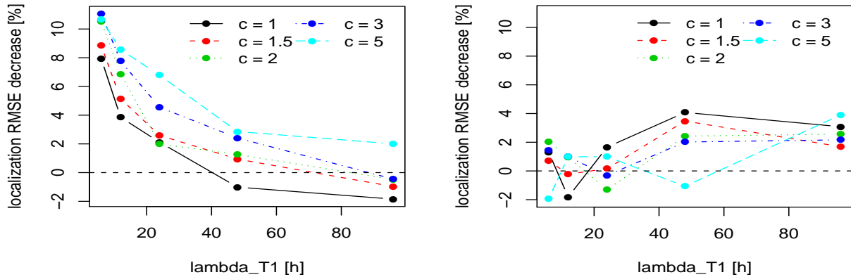
FIGURE 3.12 – Performances de localisation et durée inter-ruptures : comparaison approches uni- et multi-échelles – Réduction de (la racine carré de) l'erreur quadratique moyenne de localisation d'une rupture pour les approches Gallego et Lindeberg (resp. à gauche et à droite), vis-à-vis de l'utilisation d'une unique échelle globalement optimale, en fonction des paramètres \lambda_{T_1} et c . Ces résultats sont en contraste avec ceux obtenus pour la détection, puisque c'est l'approche de combinaison d'échelles Gallego qui obtient de meilleures performances que l'approche Linderberg, dès lors que les ruptures d'un signal sont proches. La tendance s'inverse toutefois quelque peu dès lors que la durée moyenne inter-ruptures augmente.
