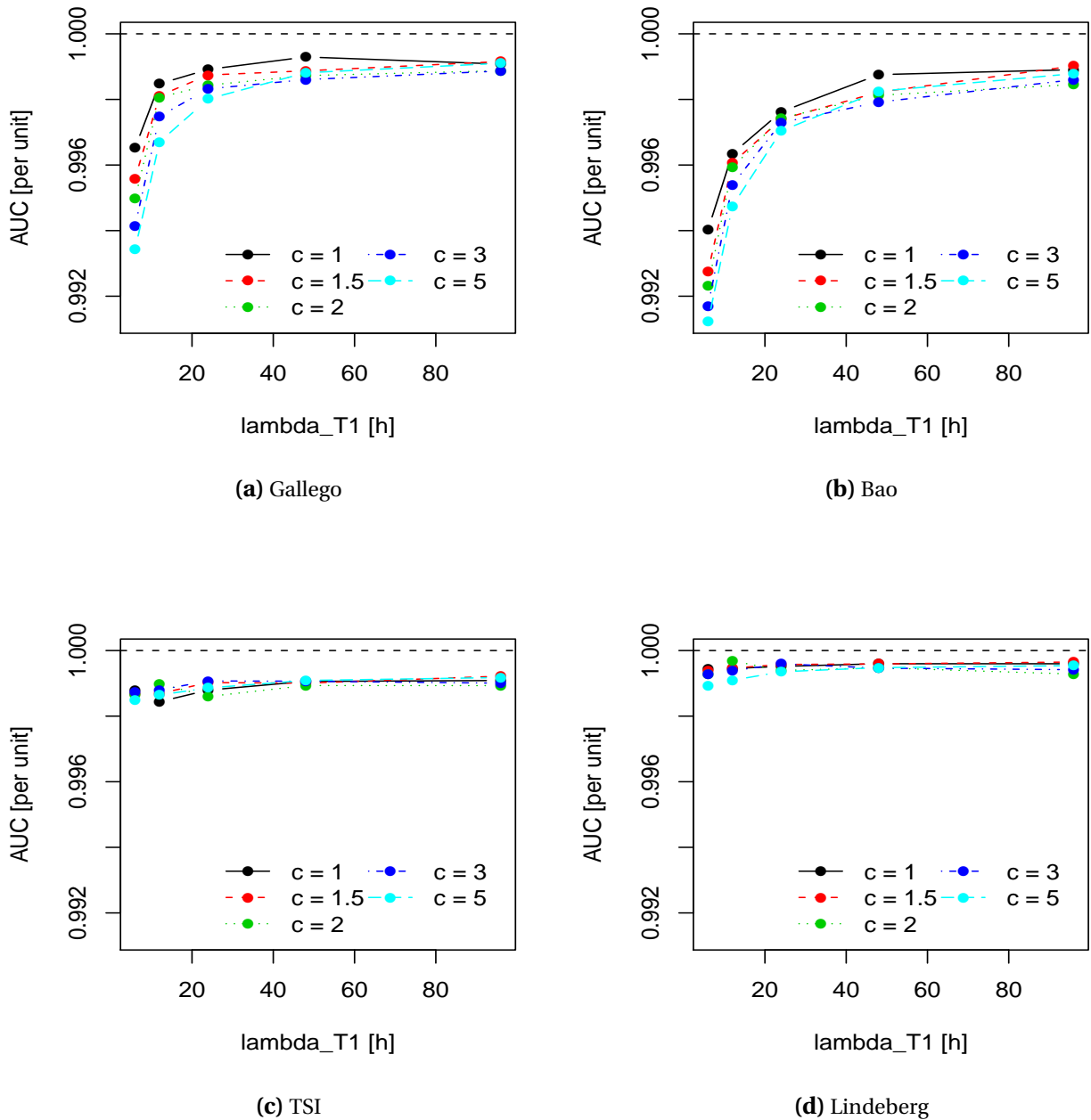
FIGURE 3.8 – Performances de détection optimales en fonction de la durée inter-ruptures – AUC maximale (i.e. pour une valeur d'échelle maximale s_n^* = \operatorname{argmax}_{s_n} AUC(\lambda_{T_1}, c) ), représentée en fonction de la durée moyenne d'un épisode de production nulle \lambda_{T_1} et du ratio définissant la durée moyenne d'un épisode de production élevée c , pour les approches : Gallego, Bao, TSI et Lindeberg. Alors que les performances des approches faisant intervenir une procédure locale de sélection d'échelle (i.e. Lindeberg et TSI) se maintiennent, celles des approches basées sur une combinaison d'échelles (i.e. Gallego et Bao) déclinent lorsque diminue la durée moyenne inter-ruptures.
