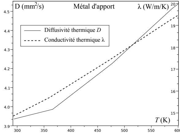
FIGURE 6.7 – Diffusivité et conductivité thermiques vs T
