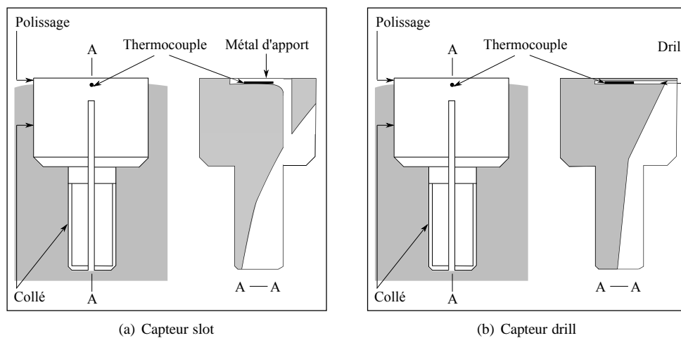
FIGURE 6.2 – Capteurs slot et drill
