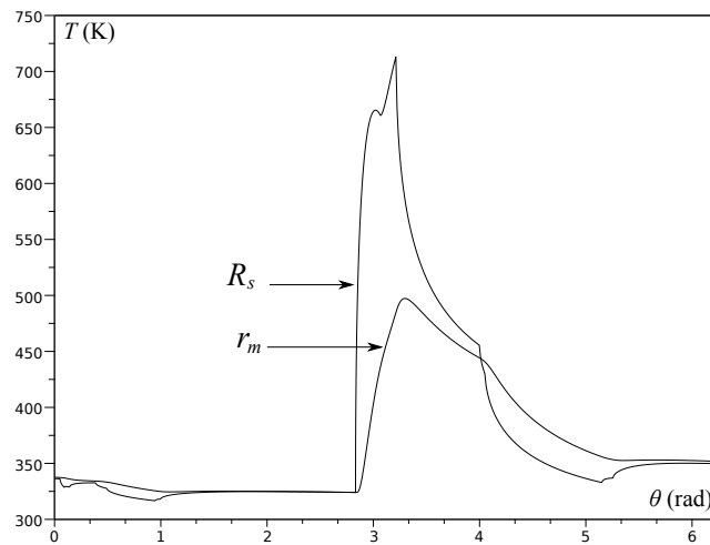
FIGURE 7.3 – Température simulée aux rayons R_s et r_m .
