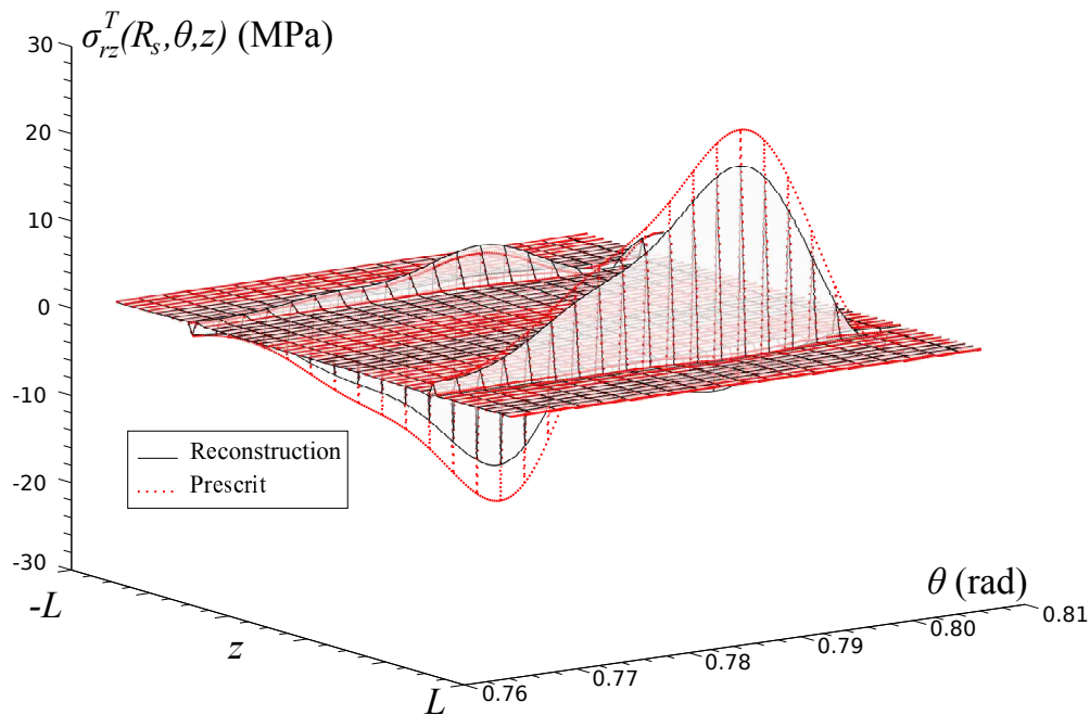
FIGURE 9.5 – Reconstruction de la contrainte ( rz ) pour N_z^m = 500
