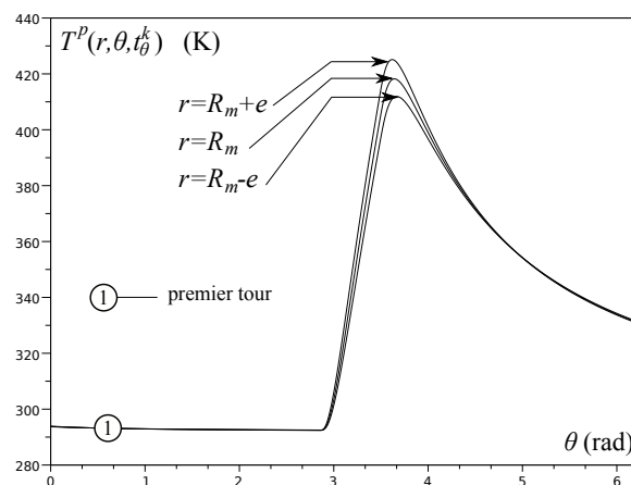
FIGURE 5.10 – Température d'entrée à différentes profondeurs
