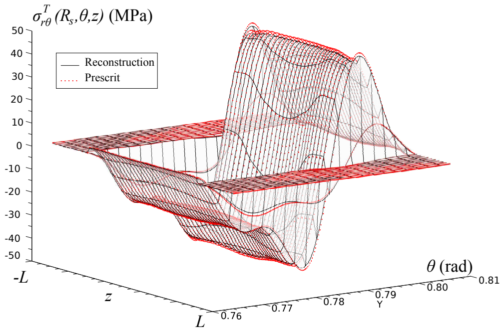
FIGURE 9.4 – Reconstruction de la contrainte ( r\theta ) pour N_z^m = 500
