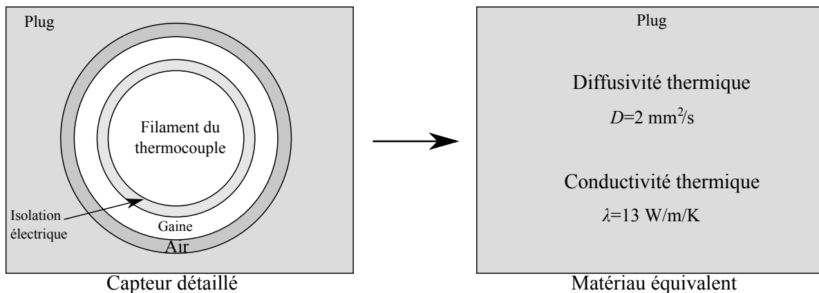
FIGURE 6.6 – Matériau équivalent
