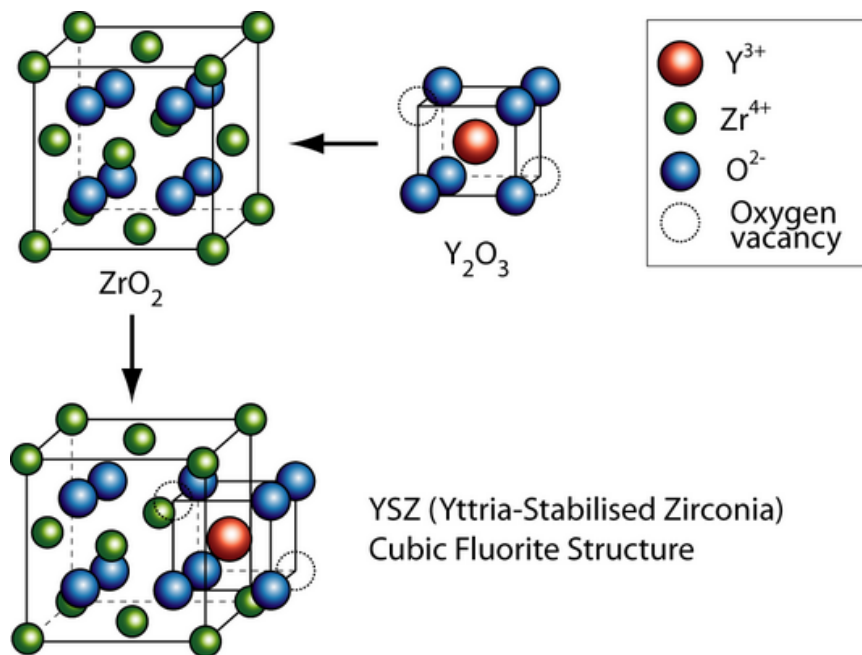
Figure I.2. Structure cristalline de l'électrolyte YSZ.
