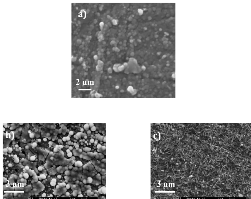
Figure II.3. Micrographies MEB des couches minces d'oxyde de cérium déposées par CBD à 60°C sur acier inoxydable 316L, avec un temps d'immersion de (a) 2 heures (épaisseur~330 nm), (b) 6 heures (~1 \mu\text{m} ), avant recuit et (c) 6 heures après recuit à 600 °C durant 4 heures sous air.
