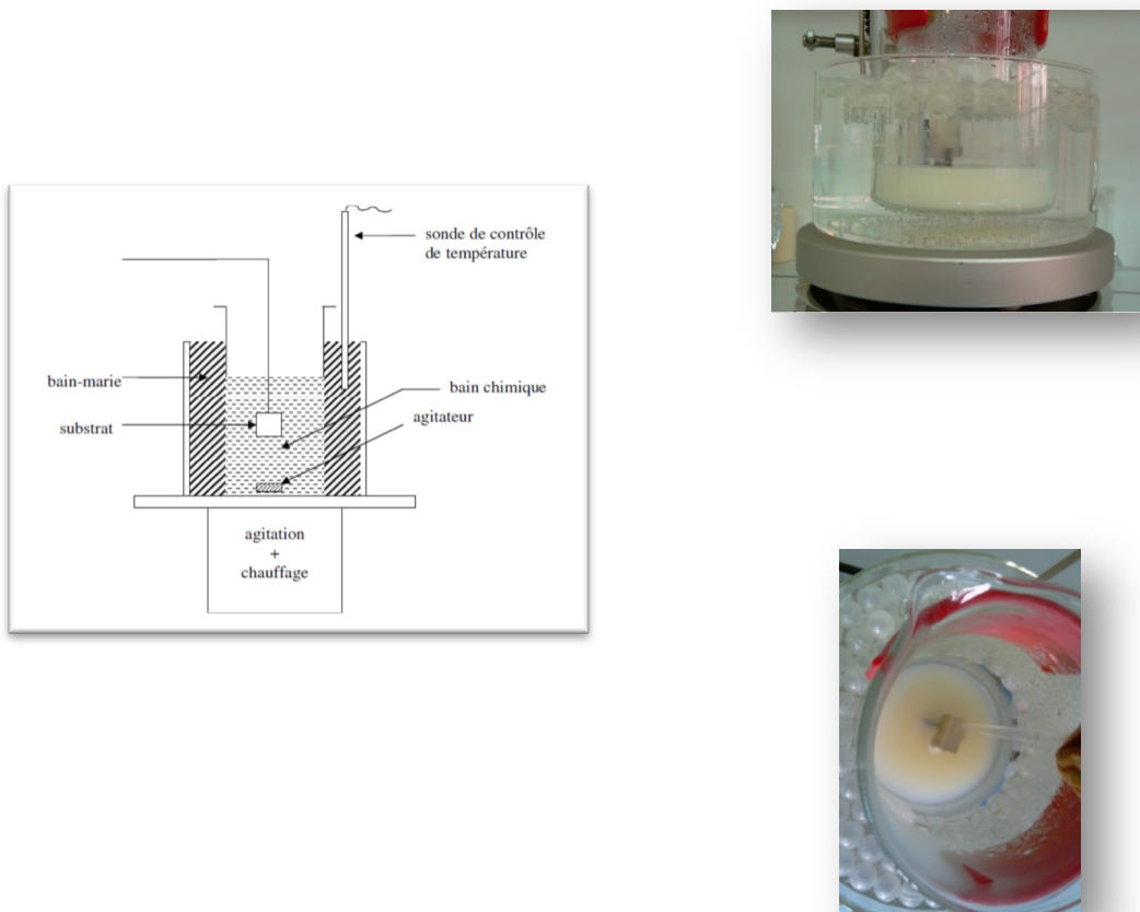
Figure II.1. Schéma du montage expérimental pour les dépôts par CBD, et photographies du dispositif utilisé.
