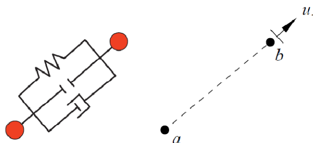
Figure II-21: Le connecteur « AXIAL ». (122)
