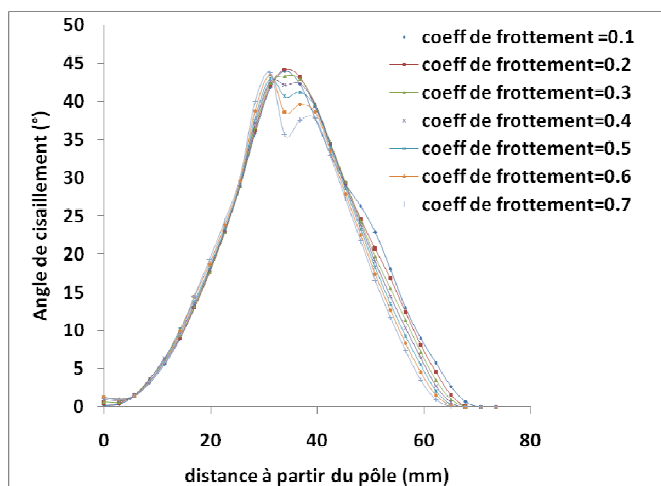
Figure IV-19 : Distribution des angles de cisailement pour le modèle non-linéaire.
