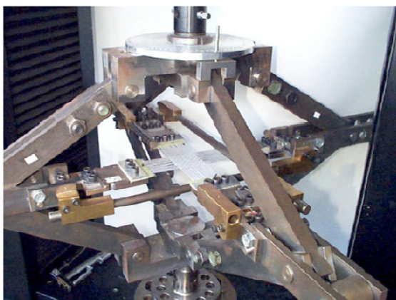
Figure II-2 : Dispositif de traction biaxiale et réponse de tissu à différentes valeurs de k (59)
