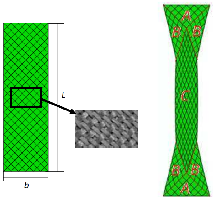
Figure II-5 : « Bias test » : éprouvette avant et après déformation
