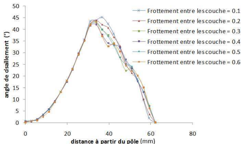
Figure IV-24 : Evolution des angles de cisaillement pour la couche orienté à (0°/90°)
