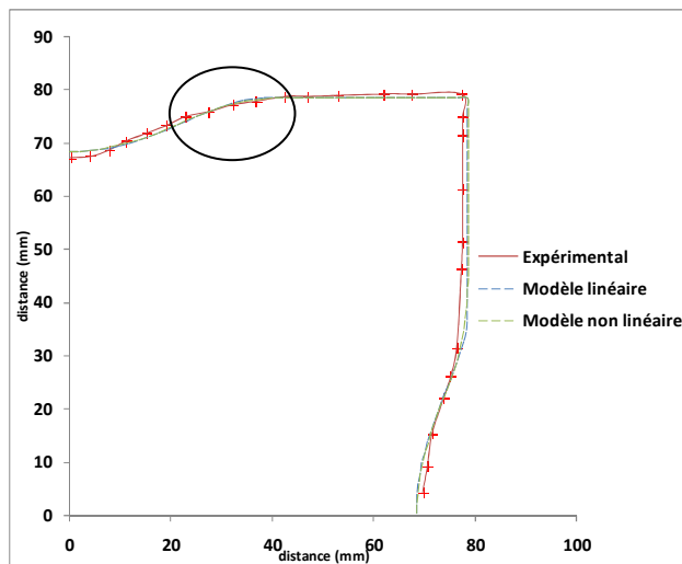
Figure III-14 : Profils de l'avalement de l'embouti (0°/90°)
