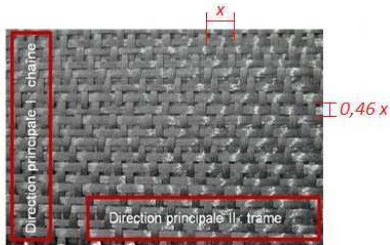
Figure IV-9 : La surface du renfort G1151
