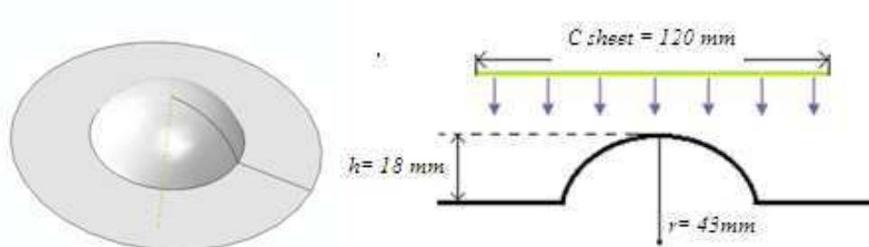
Figure I-26 : Géométrie de l'outillage.
