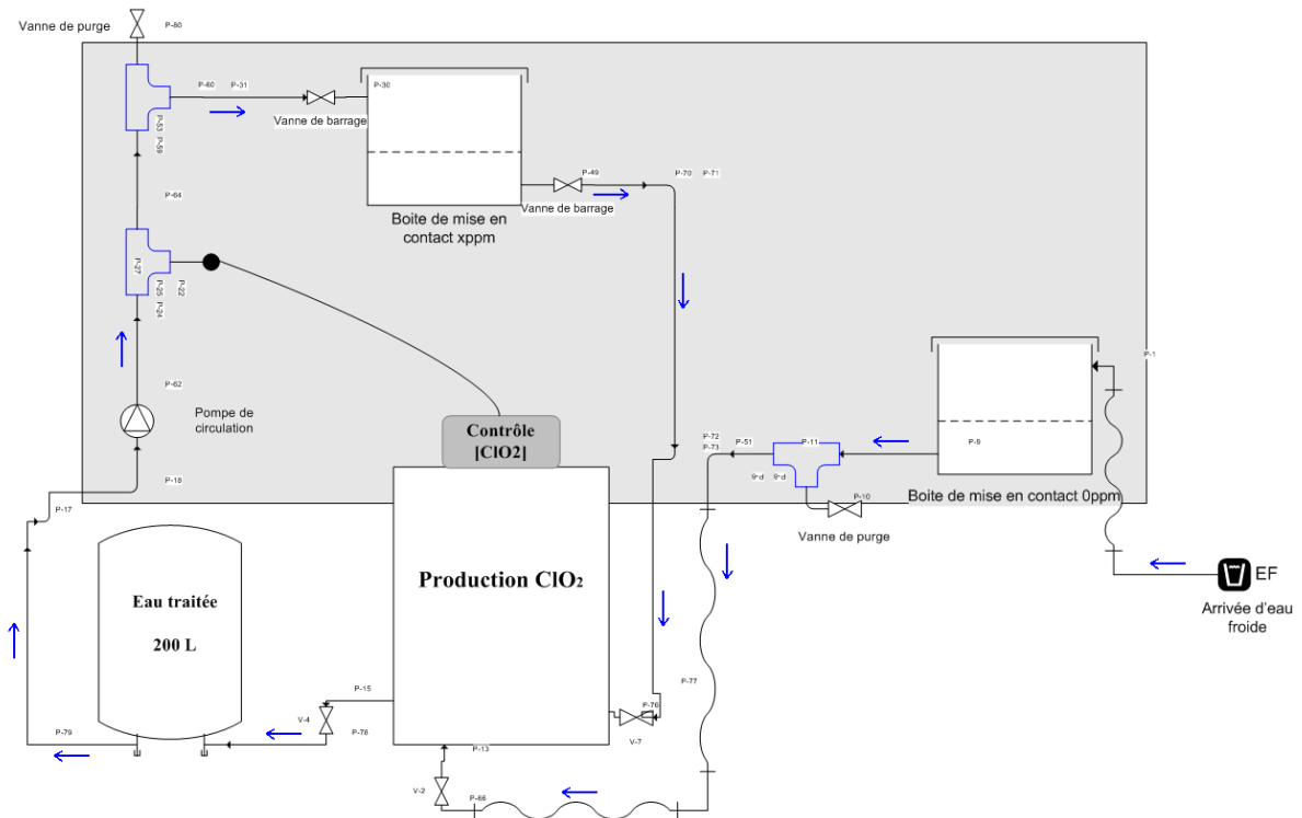
Figure 2-5 : Banc du vieillissement au DOC.
