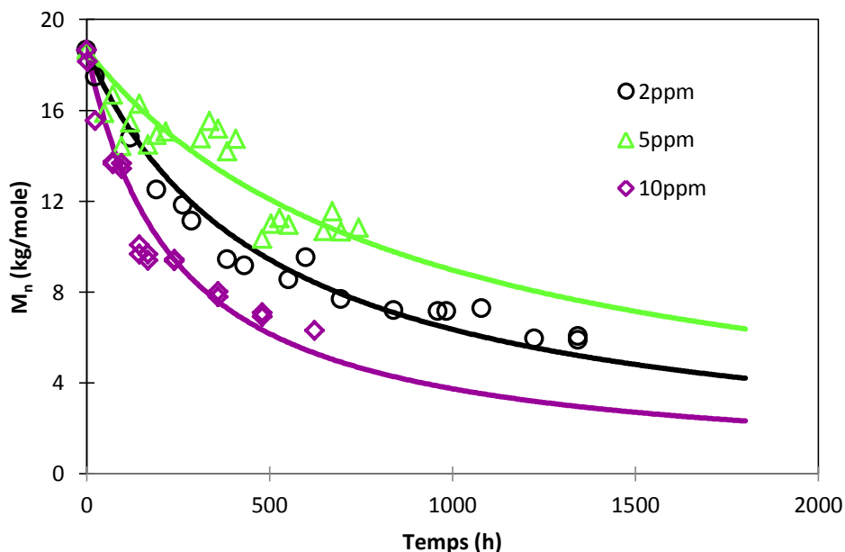
Figure 6-5 : Evolution de la masse molaire moyenne en nombre ( M_n ) du PA 6,6 à 17°C dans des solutions de 2, 5 et 10 ppm de DOC. Comparaison entre la théorie (traits continus) et l'expérience (symboles).
