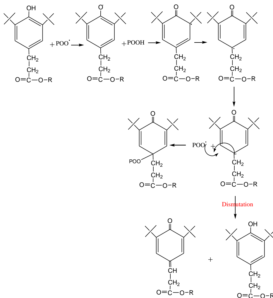
Figure 1-37 : Mécanisme réactionnel des phénols.
