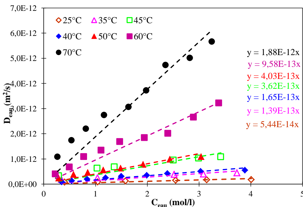
Figure 3-7 : Variation du coefficient de diffusion d'eau en fonction de la concentration d'eau à l'équilibre entre 25 et 70°C pour HR ≤ 50%.
