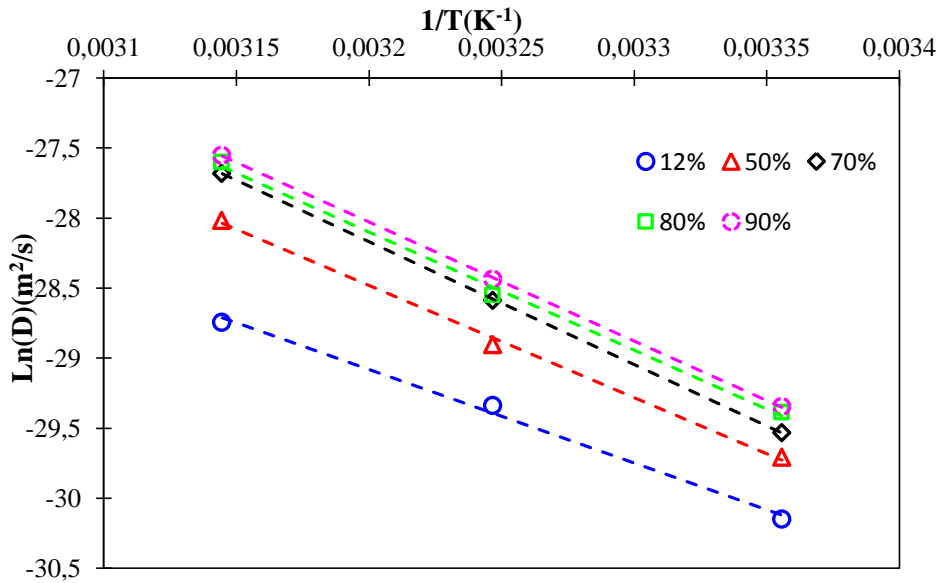
Figure 3-10 : Graphe d'Arrhenius du coefficient de diffusion d'eau dans le PA 6,6 entre 25 et 45°C entre 10 et 90 % HR [2].
