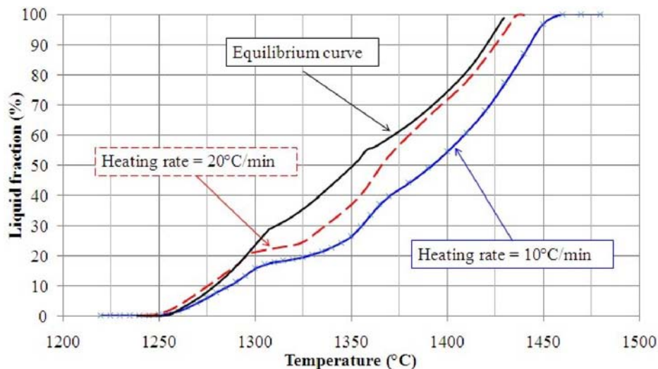
Fig. 3.9. Fraction liquide en fonction de la température obtenue par DSC et Thermo-Calc.
