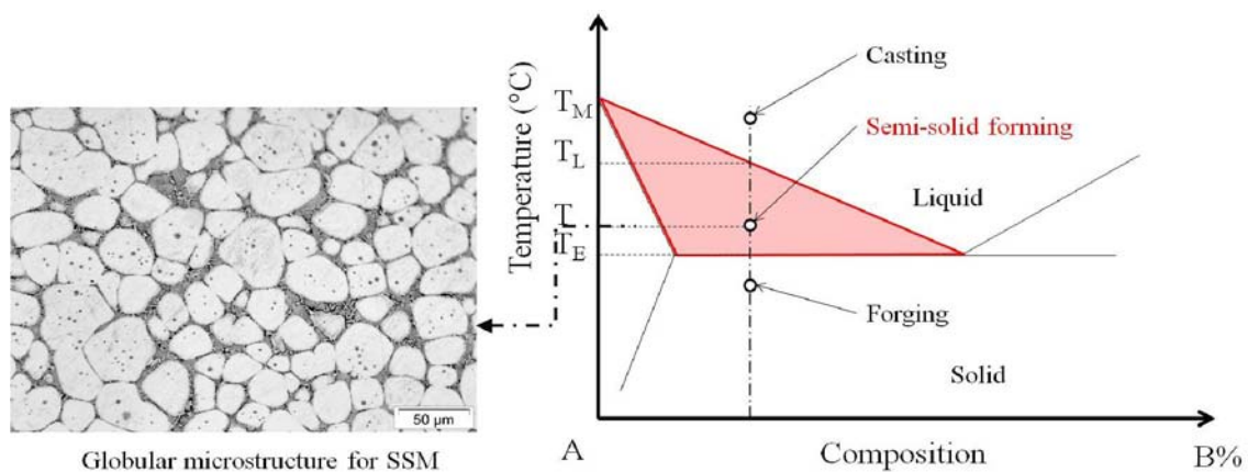
Fig. 1.2. Domaine de température typique pour les différents procédés.
