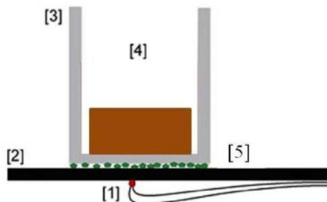
Fig. 2.27. Schéma du creuset dans lequel l'échantillon est placé. [1] Thermocouple Pt/Pt-10%Rh, [2] support en platine, [3] creuset, [4] échantillon, [5] poudre \text{Al}_2\text{O}_3 pour empêcher la soudure de pièces en platine.
