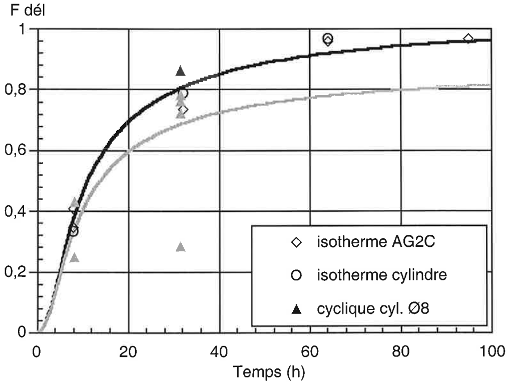
Figure VI.34 : évolution de la fraction de délamination à l'interface oxyde / métal en fonction du temps de pré-oxydation, comparaison des éprouvettes pré-oxydées en isotherme et sous oxydation cyclique.
