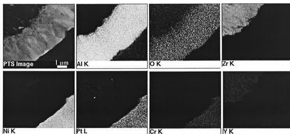
Figure III.27 : cartographies réalisées en microanalyse X sur la couche d'alumine et ses interfaces avec la zircone et la sous-couche, échantillon avec un substrat yttrié oxydé 192h à 1100°C.
