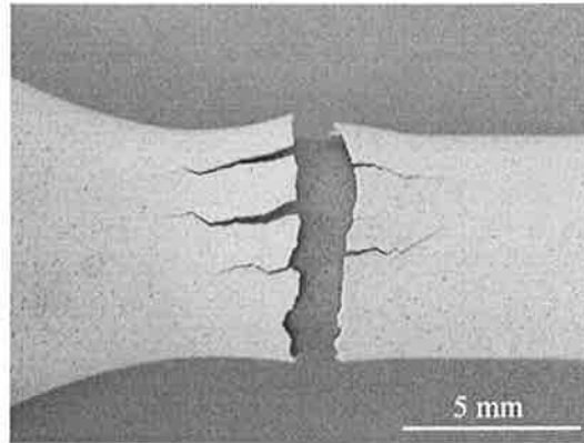
Figure V.4 : éprouvette 83A1 (AM1 bas soufre, pré-oxydation cyclique 45 cycles d'1h à 1100°C, cylindre Ø 6), écaillage localisé dans la zone centrale, faciès de type 3.
