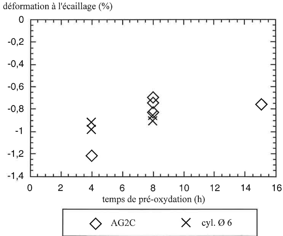
Figure V.13 : courbe d'écaillage des éprouvettes AG2C et cylindriques Ø 6, effet de la durée de pré-oxxydation isotherme sur la déformation à l'écaillage, matériau standard.
