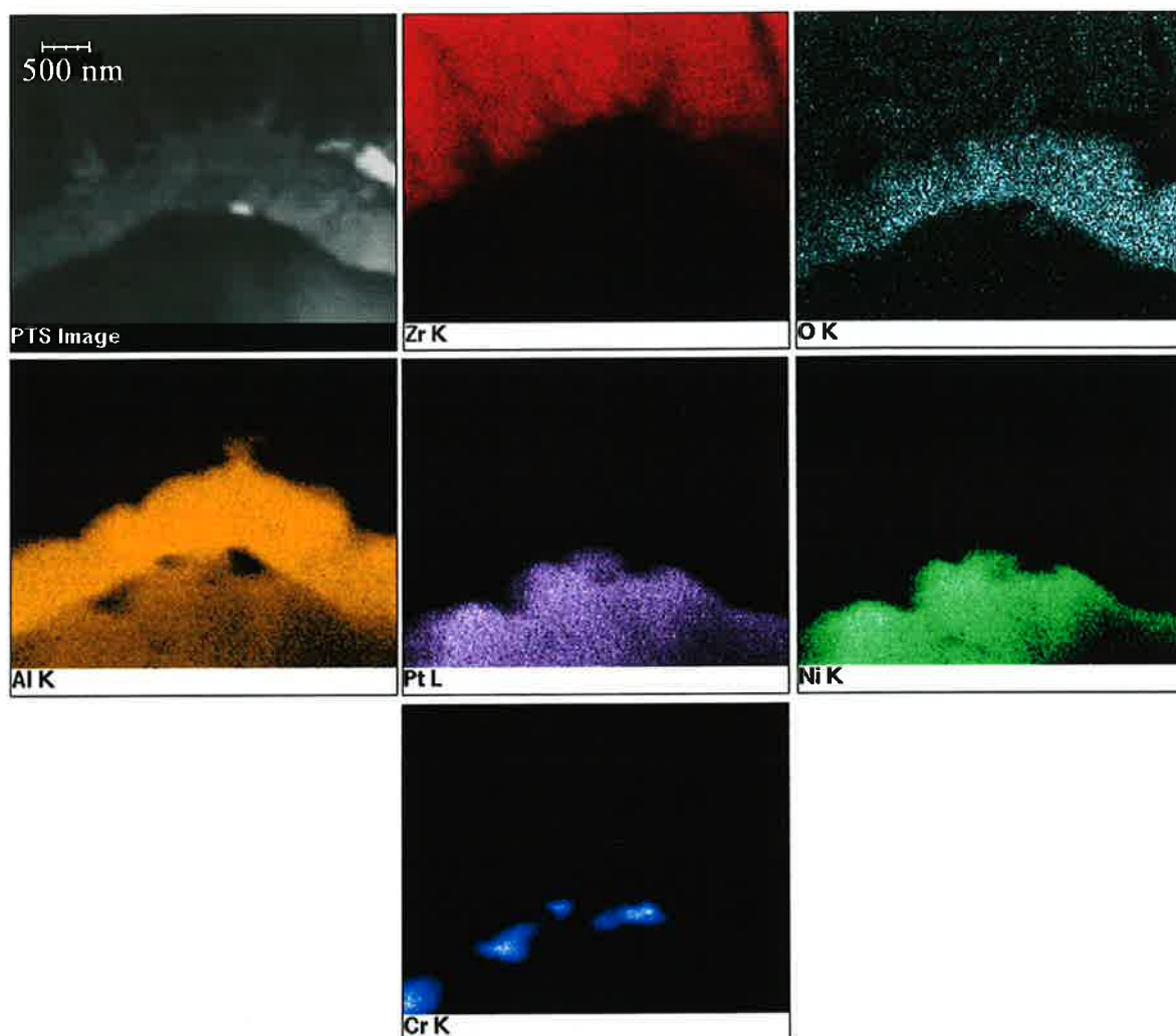
Figure II.15 : interfaces zirconie / alumine et alumine / sous-couche (cartographies X, microscopie en transmission), matériau dopé en yttrium, état brut de dépôt.
