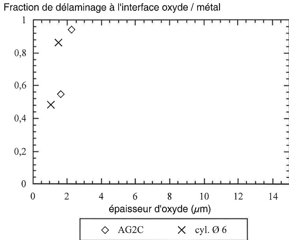
Figure V.30 : courbe de localisation de l'écaillage en fonction de l'épaisseur d'oxyde, pré-oxydation isotherme, matériau standard, comparaison entre les géométries AG2C et cylindres Ø 6
