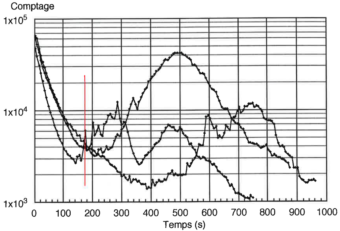
Figure VI.7 : profils du soufre obtenu par SIMS, échantillon oxydé 1h à 1100°C, AM1 standard revêtu NiAlPt, comparaison de trois profils.
