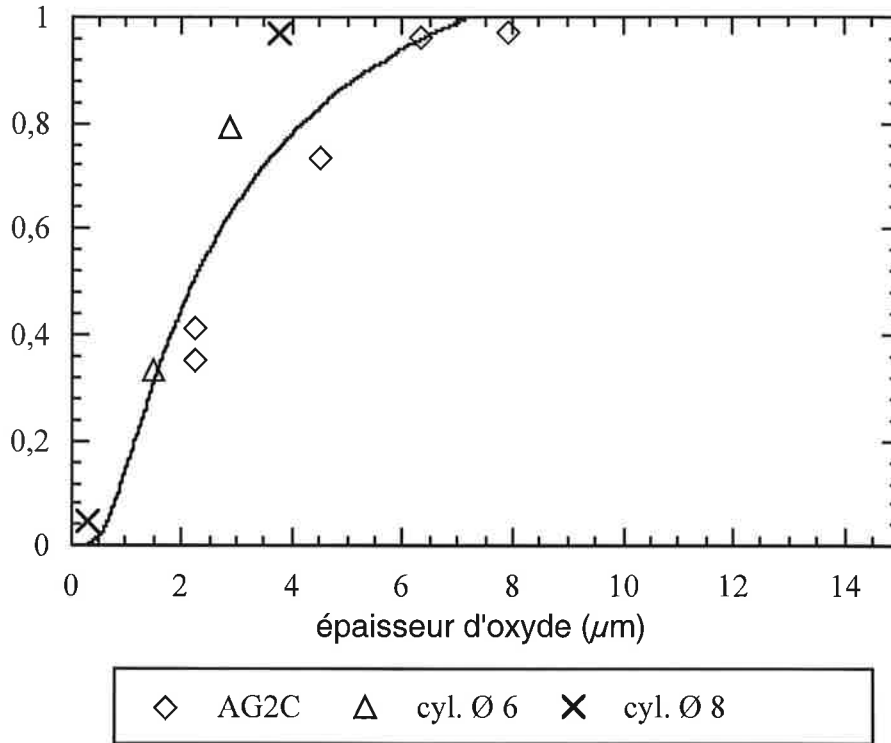
Figure V.28 : courbe de localisation de l'écaillage en fonction de l'épaisseur d'oxyde, pré-oxydation isotherme, matériau bas soufre, comparaison entre les géométries AG2C, cylindres \varnothing 6 et cylindres \varnothing 8
