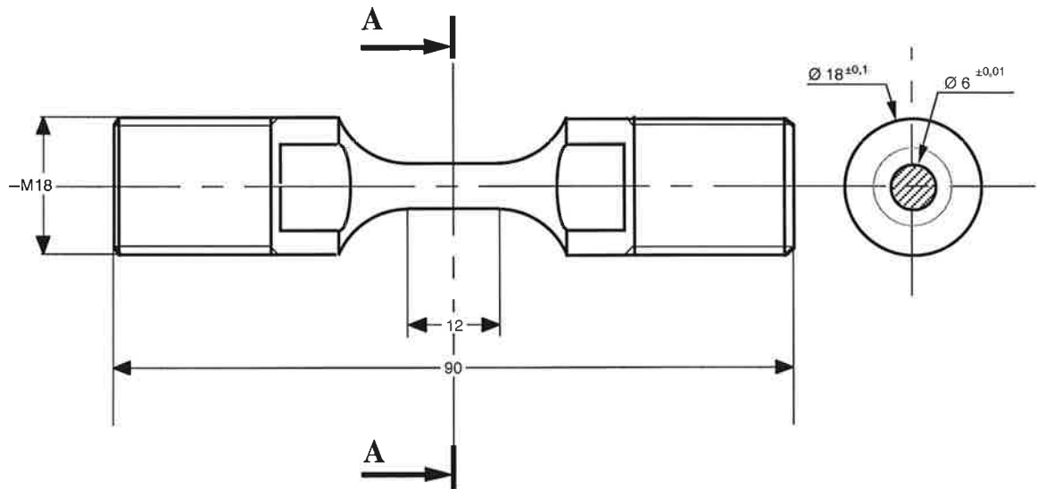
Figure I.9 : schéma de l'éprouvette cylindrique \text{Ø } 6 .
