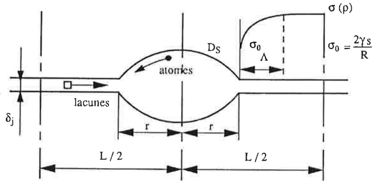
Figure VI.30 : Modèle de croissance des cavités intergranulaires par diffusion intergranulaire de Hull et Rimmer d'après François [François1995].
