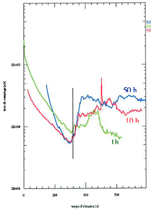
Figure VI.8 : profils du soufre obtenu par SIMS, échantillons oxydés 1h (vert), 10h (rouge) et 50h (bleu) à 1100°C, AM1 standard revêtu NiAlPt.
