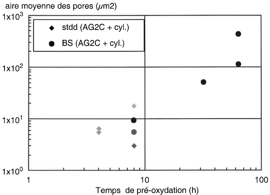
Figure VI.12 : aire moyenne des pores en fonction du temps de pré-oxydation à 1100°C, comparaison des échantillons standard et bas soufre, géométries AG2C et cylindrique, pré-oxydation isotherme.
