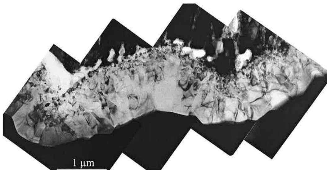
Figure III.25 : observation en microscopie en transmission de la couche d'alumine formée sur un substrat yttrié, échantillon oxydé 192h. épaisseur (μm)
