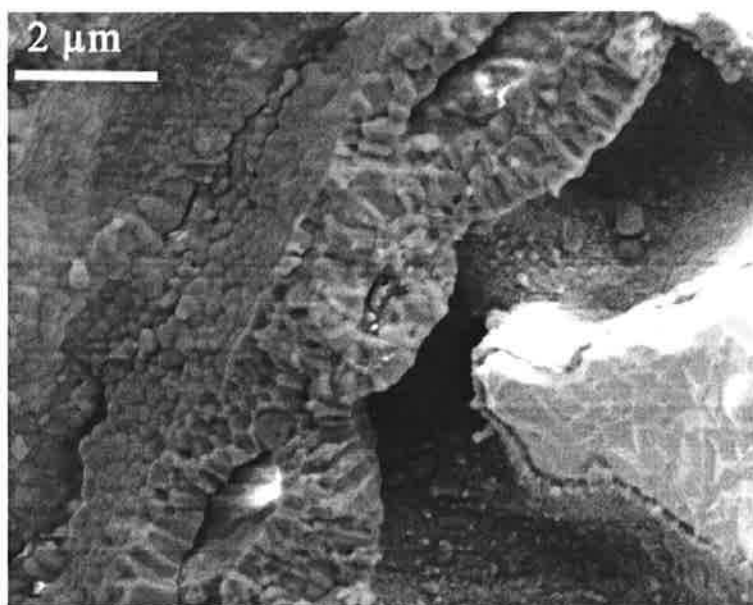
Figure IV.19 : vue des pores et de multi-couches dans une couche d'alumine et ré-oxydation d'un pore, éprouvette bas soufre testée en fatigue anisotherme, \Delta \epsilon \text{ mec} = 0,56 \% , temps équivalent à 1100^\circ\text{C} = 50\text{h} .
