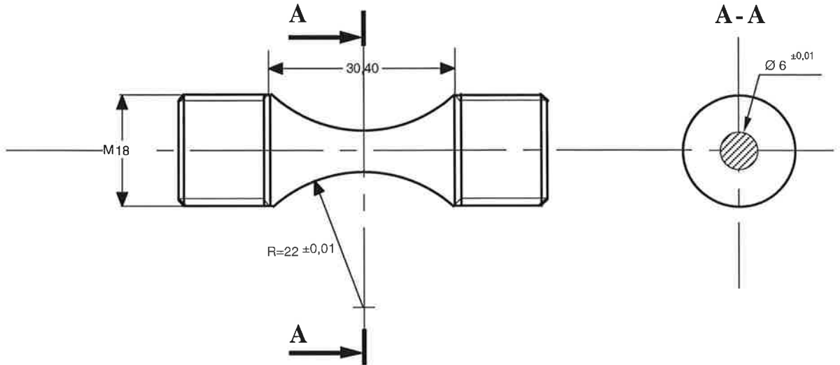
Figure I.8 : schéma d'une éprouvette AG2C (Axisymétrique à Génératrice Circulaire Concave) ou éprouvette diabolo.
