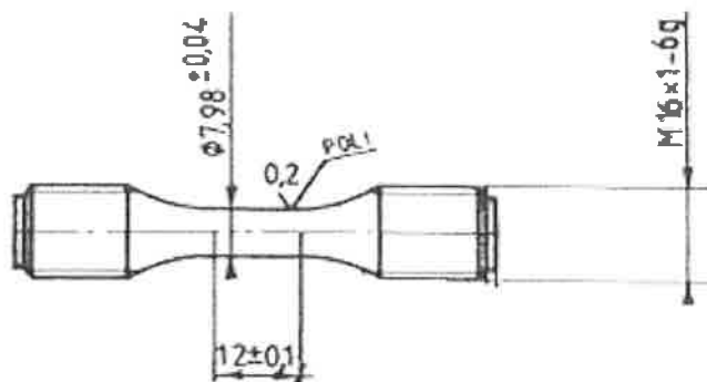
Figure I.10 : schéma de l'éprouvette cylindrique \text{Ø } 8 (d'après un document Snecma Moteurs).
