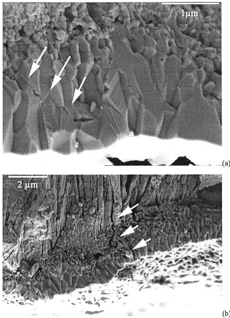
Figure VI.38 : présence de fissures dans la couche d'alumine, vue en microscopie à balayage d'écailles provenant d'une éprouvette testée en fatigue anisotherme, cycle BTBA, \Delta\varepsilon_{méc} = 0,56\% , t_{1100^{\circ}\text{C}} = 27\text{h} .
