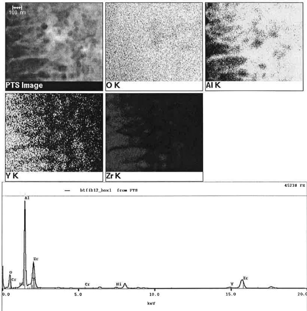
Figure III.29 : cartographies spectrales de l'interphase entre l'alumine et la zirconie et spectre associé à la zone à petits grains dans laquelle coexistent des grains d'alumine et de zirconie, microscopie en transmission, lame mince en section transverse réalisée par FIB et analyse en mode STEM, échantillon oxydé 8h en fatigue anisotherme.
