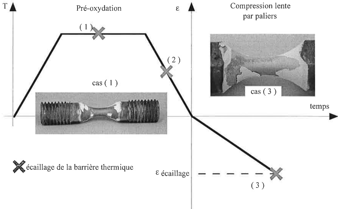
Figure VI.21 : schéma montrant les différents cas d'écaillage (1. pendant le traitement d'oxydation, 2. au cours du refroidissement, 3. au cours de l'essai de compression).
