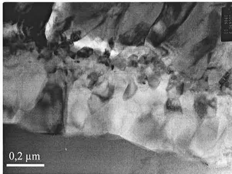
Figure IV.1 : observation de la couche d'alumine formée sur un échantillon avec un substrat bas soufre oxydé 50h à 1100°C, lame mine en section transverse observée en MET. T éprouvette (°C)
