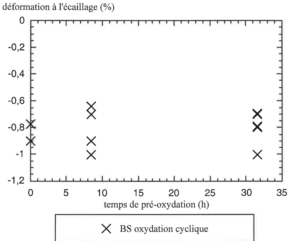
Figure V.14 : courbe d'écaillage des éprouvettes cylindriques Ø 8, effet de la durée de pré-oxxydation cyclique sur la déformation à l'écaillage, matériau bas soufre.
