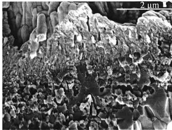
Figure III.28 : interface zircon (contraste clair) / alumine (contraste foncé), échantillon à substrat bas soufre oxydé 32h à 1100°C ( électrons secondaires, MEB).
