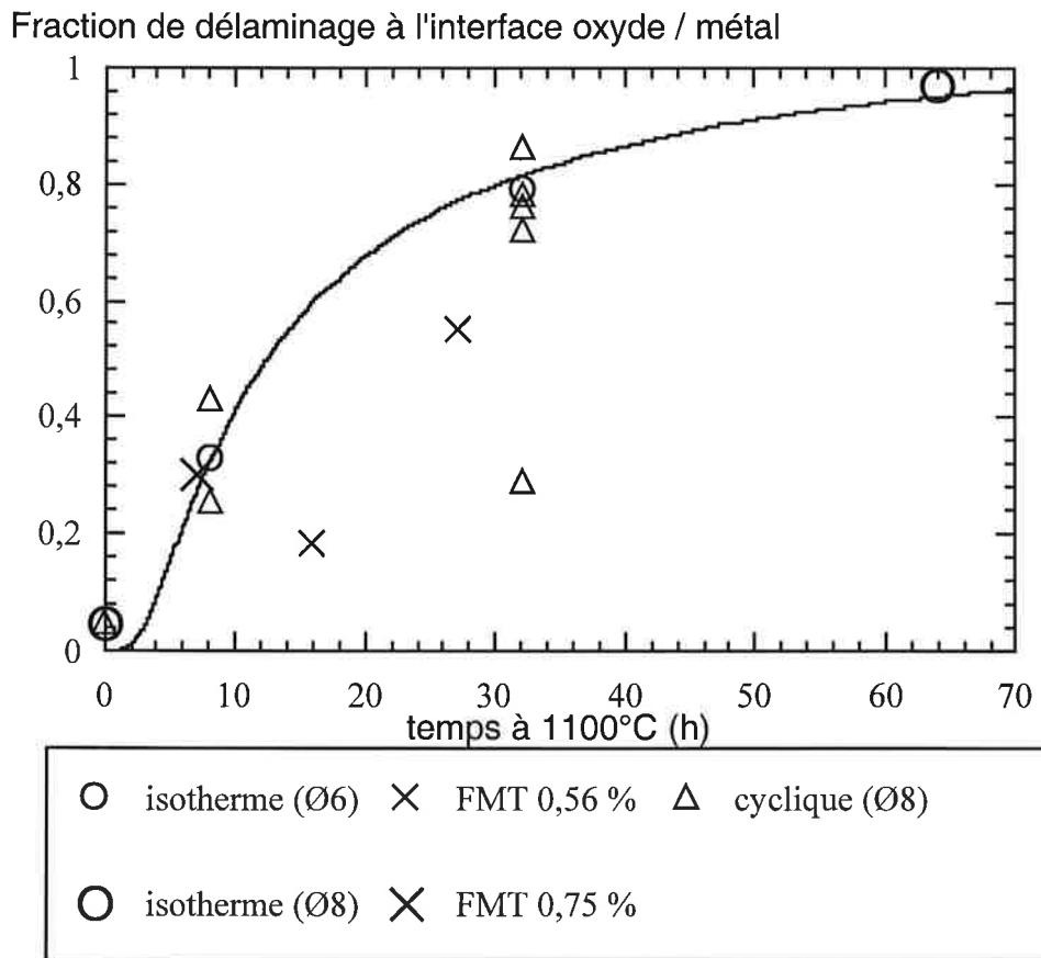
Figure V.33 : courbe de localisation de l'écaillage, matériau bas soufre, géométries cylindriques Ø 6 Ø 8 et tubulaires, comparaison en fonction du type de pré-oxidation.
