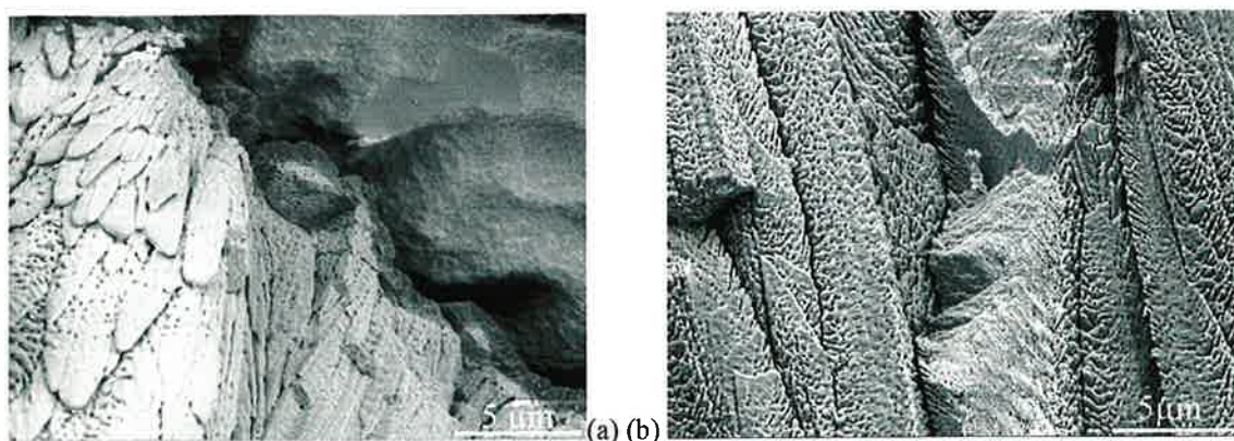
Figure II.16 : fractographie montrant la microstructure du revêtement céramique. (a) échantillon 84C2, 12 cycles à 1100°C, (b) échantillon X5950A, fatigue anisotherme t (à 1100°C) = 16h.
