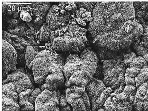
Figure III.21 : vue de la surface convolutive de la couche d'alumine formée sur un échantillon plan avec un substrat bas soufre après ré-oxydation de la sous-couche suite à l'écaillage lors d'un traitement thermique de 500 h à 1100°C.
