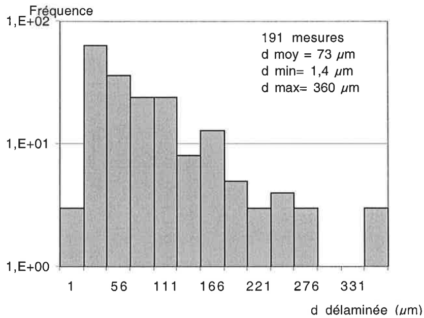
Figure VI.24 : histogramme des distances délaminées, éprouvette AG2C pré-oxydée en isotherme 64h à 1100°C, substrat bas soufre.
