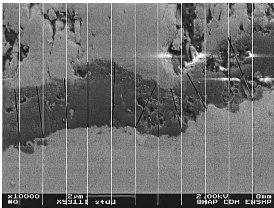
Figure AII.1: exemple de mesures de l'épaisseur d'oxyde sur une coupe de l'échantillon X53111.
