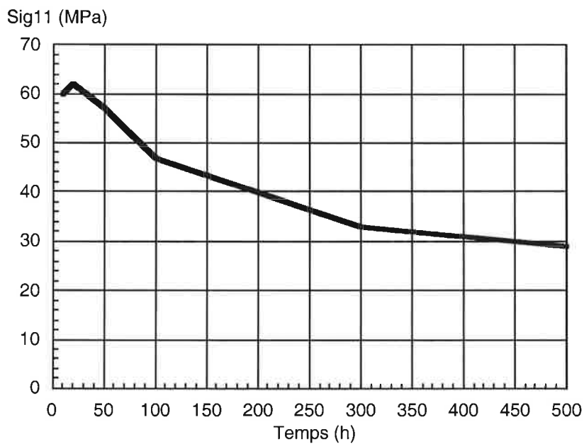
Figure VI.28: évolution des contraintes radiales à chaud en fonction de l'épaisseur d'oxyde, d'après Caliez [Caliez2001].
