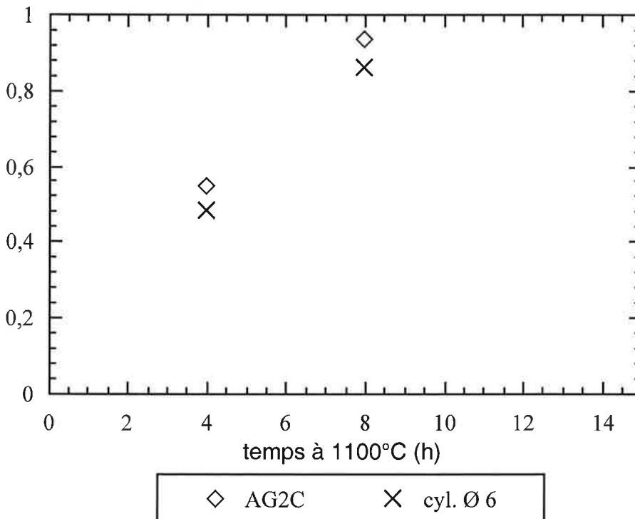
Figure V.29 : courbe de localisation de l'écaillage, pré-oxydation isotherme, matériau standard, comparaison entre les géométries AG2C et cylindres \varnothing 6
