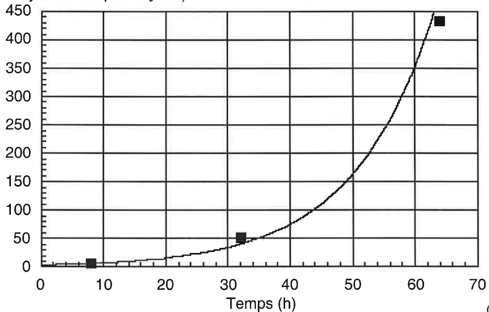
Figure VI.29 : (a) aire moyenne des pores indépendants en fonction du temps d'oxydation isotherme à 1100^\circ\text{C} , éprouvettes AG2C avec un substrat bas soufre,
