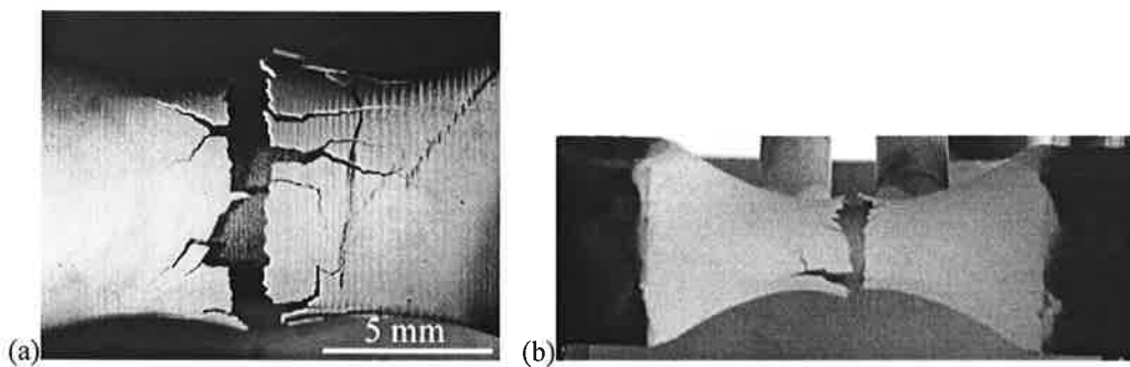
Figure V.6 (a et b): éprouvette X5947D (AM1 bas soufre, oxydation isotherme 32h à 1100°C, AG2C) (a) importante fissuration transverse orientée parallèlement à la direction de sollicitation, (b) l'écaillage est localisée dans la section centrale de l'éprouvette de plus faible rayon de courbure.
