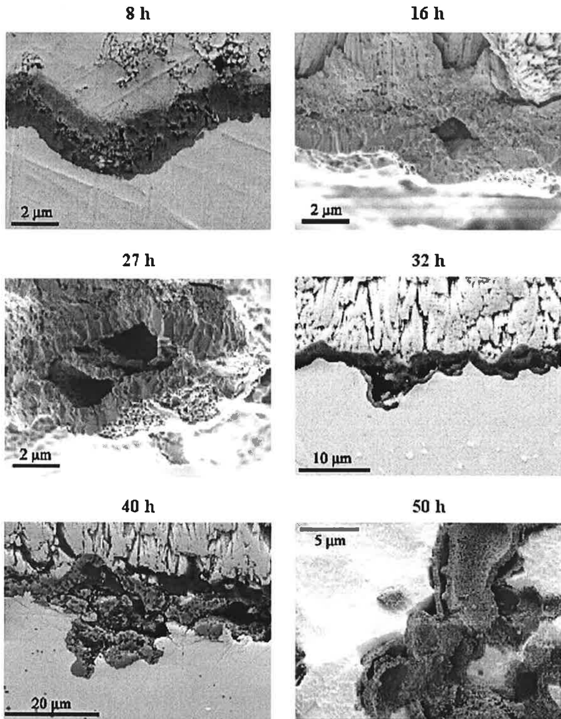
Figure IV.17 : évolution de la porosité dans la couche d'alumine, éprouvettes bas soufre testées en fatigue anisotherme, cycle BTBA ( \Delta \epsilon_{\text{méc}} = 0,56 \% ), temps équivalent à 1100°C entre 8h et 50h, observations sur coupes (8h, 32h et 40h), sur écailles (16h et 27h) et en surface (50h) en microscopie à balayage.
