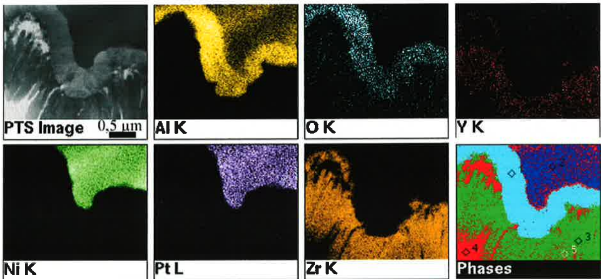
Figure II.14 : interfaces zircon / alumine et alumine / sous-couche (cartographies X, microscopie en transmission), matériau dopé en yttrium, état brut de dépôt.
