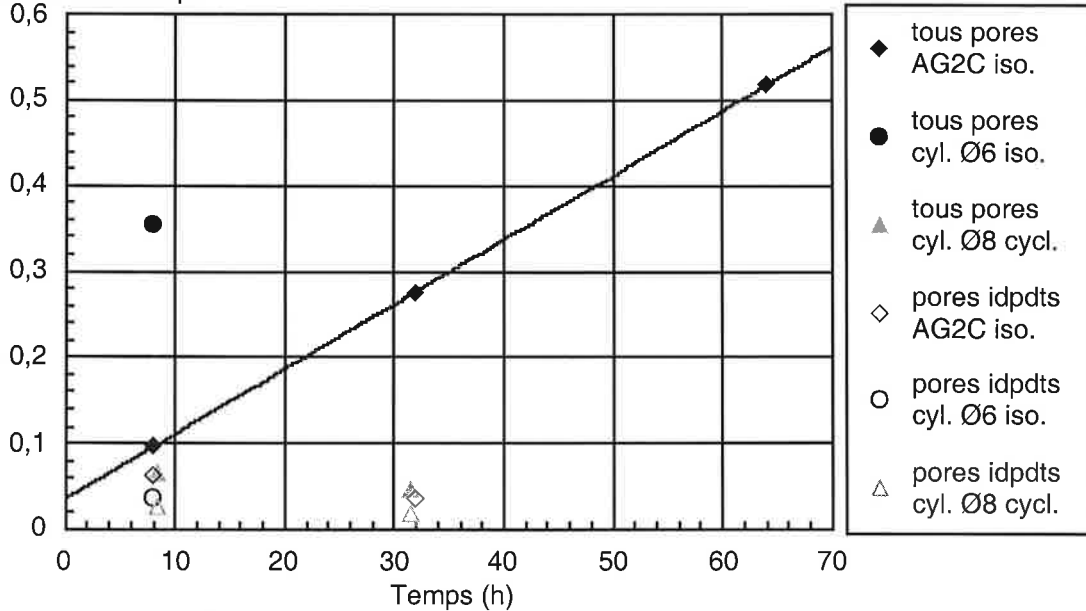
Figure VI.31 : fraction surfacique de pores (tous les pores et pores indépendants) en fonction du temps équivalent à 1100°C, comparaison des pré-oxydations cycliques et isothermes.
