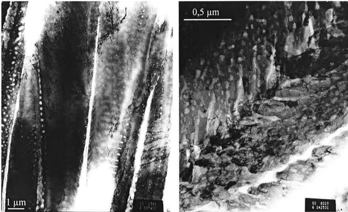
Figure II.20 : pores intragranulaires alignés dans la zircone (microscopie en transmission).
