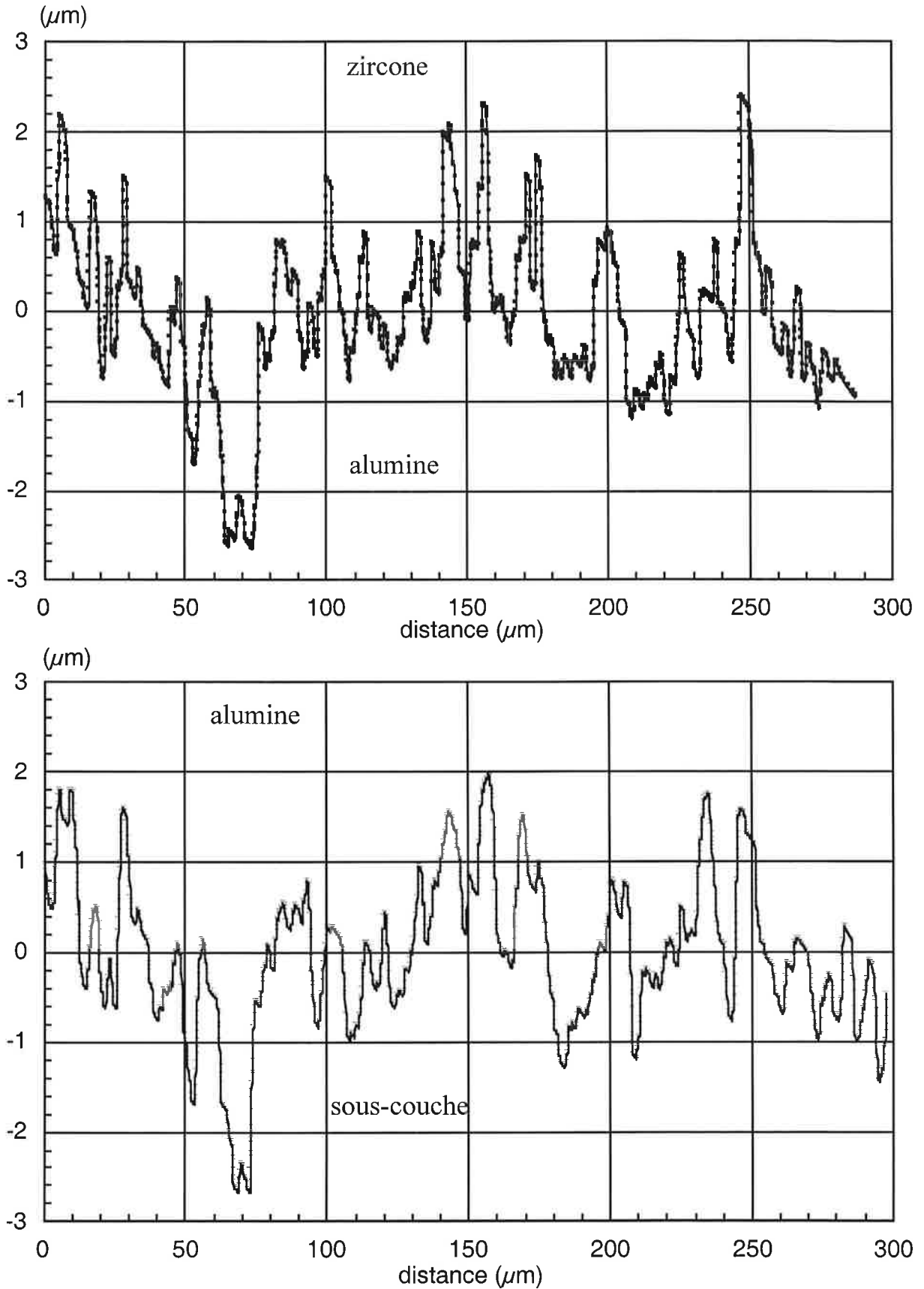
Figure III.22 : graphes représentant la rugosité aux interfaces zirconium/ alumine et alumine / sous-couche après un traitement de 50h à 1100°C (échantillon KZ4-1, plan bas soufre).
