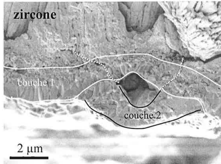
Figure VI.37 : vue d'une multicouche composée de deux monocouches sur une écaille d'une éprouvette testée en fatigue anisotherme, cycle BTBA, \Delta\varepsilon_{méc} = 0,56\% , t_{1100^{\circ}\text{C}} = 16\text{h} .
