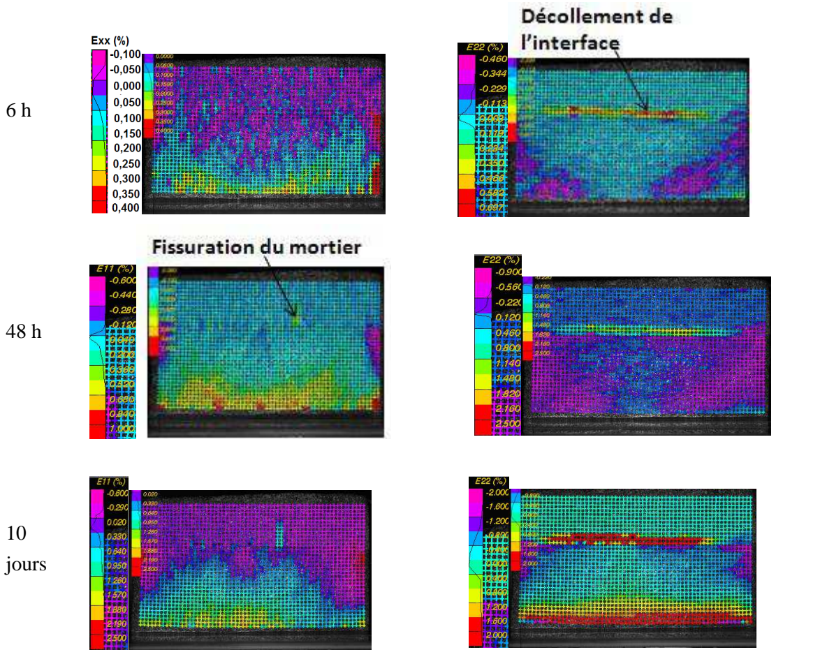
Figure A3-1 : Évolution des déformations d'un assemblage épiceá sens convexe-mortier soumis à un test d'imbibition.
