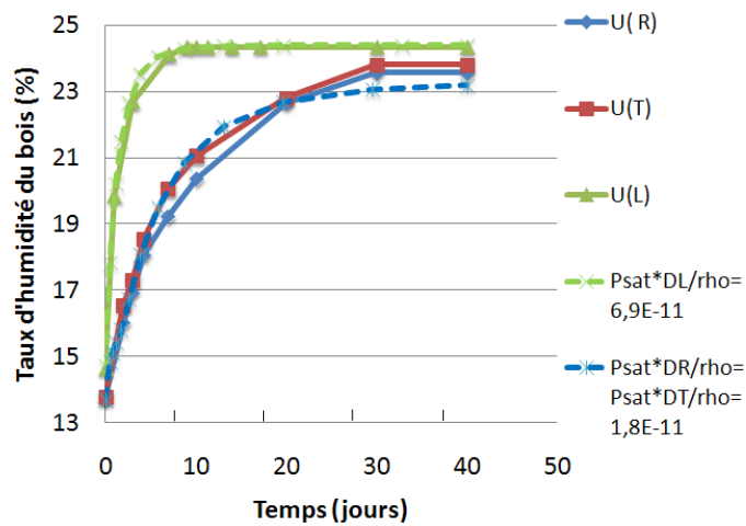
Figure 2-8 : Courbes représentant le taux d'humidité moyen dans le bois (a) initialement à l'équilibre à HR=55 % soumis à HR=81 %, (b) initialement à l'équilibre à HR=81 % soumis à HR=97 %, obtenues expérimentalement (traits pleins) et par le calcul (pointillés) pour le cas de l'épicéa. Les valeurs de Psat.D/rho indiquées sur les graphes sont exprimées en m^2.s^{-1} .
