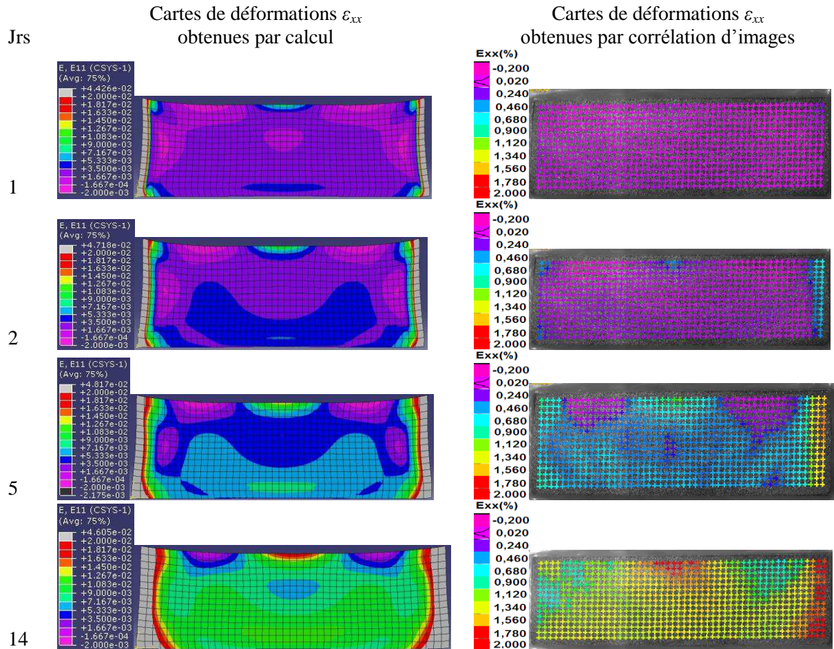
Figure 5-4 : Comparaison des cartes de déformations \epsilon_{xx} numériques et expérimentales à 1, 2, 5 et 14 jours de l'Épicéa.
