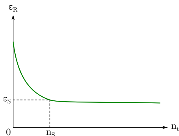
FIGURE 2.4 – Évolution de l'allongement à rupture en fonction de l'avancement de la réaction de coupure de chaîne [204]
