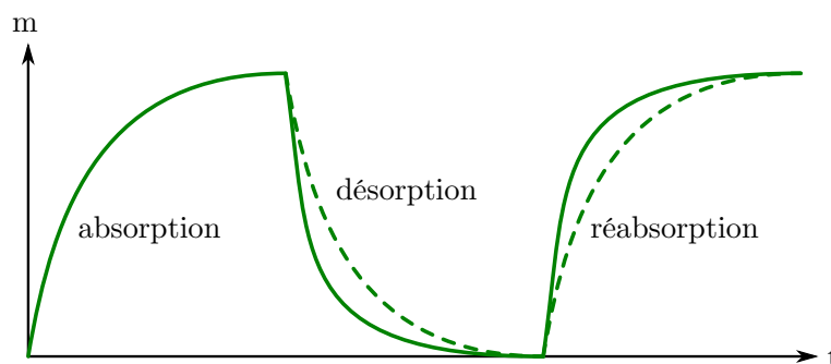
FIGURE 2.9 – Diffusion avec endommagement, mise en évidence par des cycles de sorption [67] ; les cinétiques sans endommagement sont représentées en pointillés
