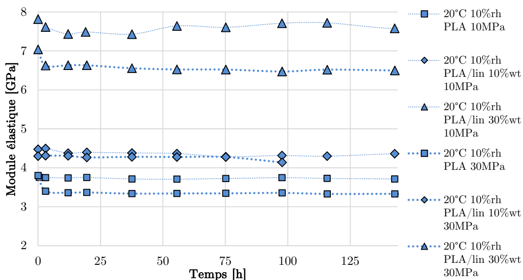
FIGURE 9.2 – Module d'élasticité du PLA et des composites PLA/lin au cours du fluage en atmosphère sèche à 20°C (10%hr)
