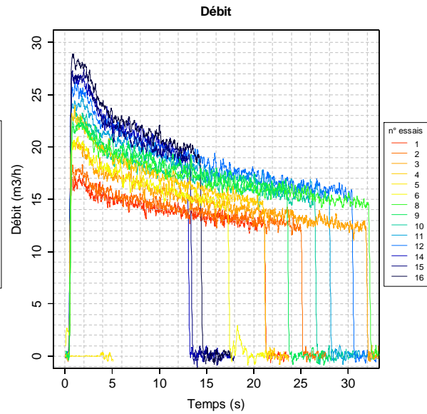
Figure 136 : débit ; caractérisation
