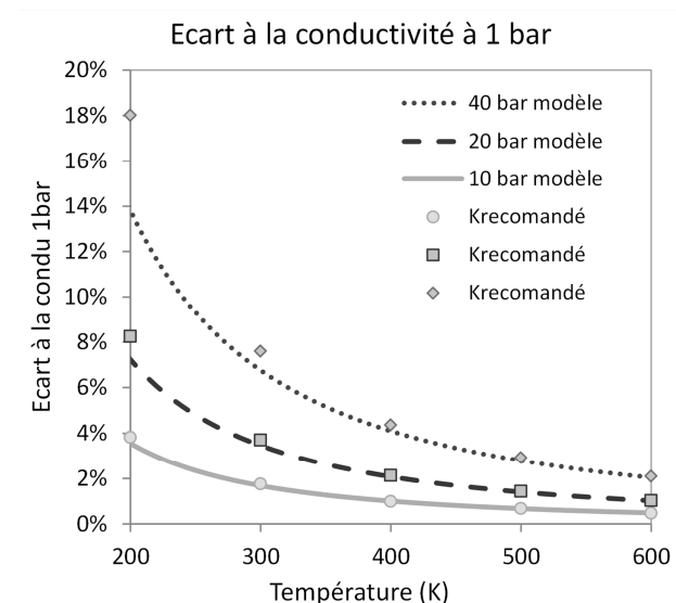
Figure 57 : écart à la conductivité à 1 bar de l'air pour différents couples P-T [20]
