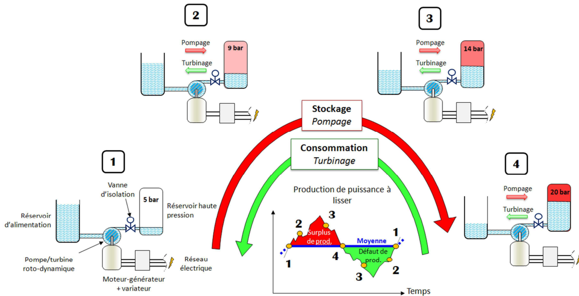
Figure 9 : principe de fonctionnement du système de stockage hydropneumatique en cycle fermé En parallèle, concernant le réservoir de stockage, on pourrait s'inspirer d'un système de compresseur volumétrique d'air dans lequel des chambres de compression diverses alimentent un grand réservoir d'accumulation, et non pas se limiter à une chambre de compression seule. Ce mode de fonctionnement, évoqué dans [9], est désigné comme un cycle ouvert. Il est illustré par la Figure 10.
