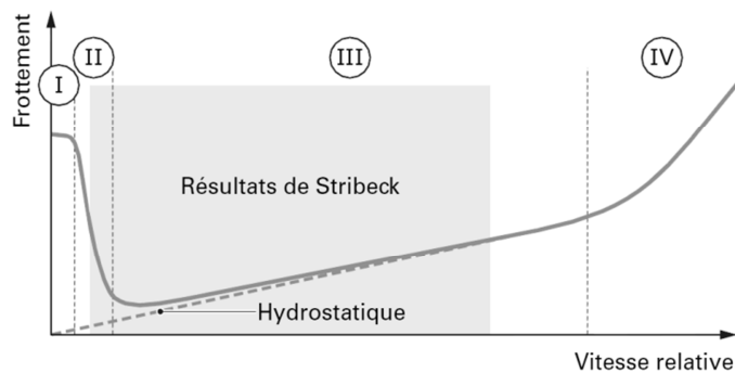
Figure 88 : coefficient de frottement fonction de la vitesse relative [33] ; zone I : lubrification limite, zone II : lubrification mixte, zone III : lubrification hydrodynamique, zone IV : régime non laminaire pour contacts de surface
