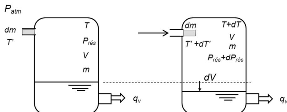
Figure 68 : évolutions subies par l'air du réservoir d'alimentation
