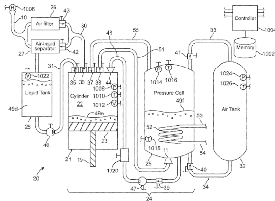
Figure 13 : structure du système de stockage LightSail Energy [11]
