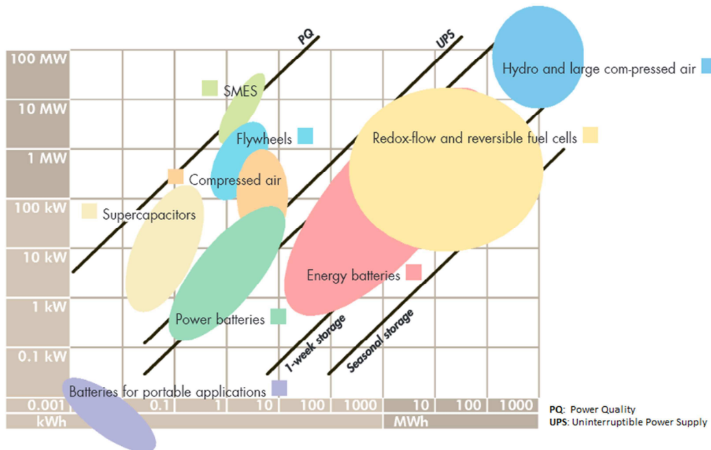
Figure 2 : Capacité énergétique et puissance de sortie de différentes technologies de stockage ; la taille des zones indiquées est à l'image de plages de puissances et énergies possibles [2]
