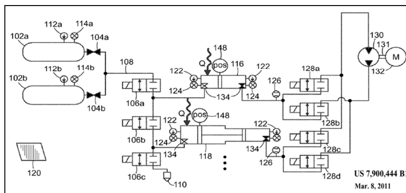
Figure 12 : système de stockage SustainX [10]
