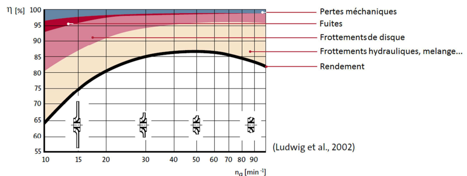
Figure 73 : rendement hydraulique selon le type de pompe ; courbe adapté par [29]
