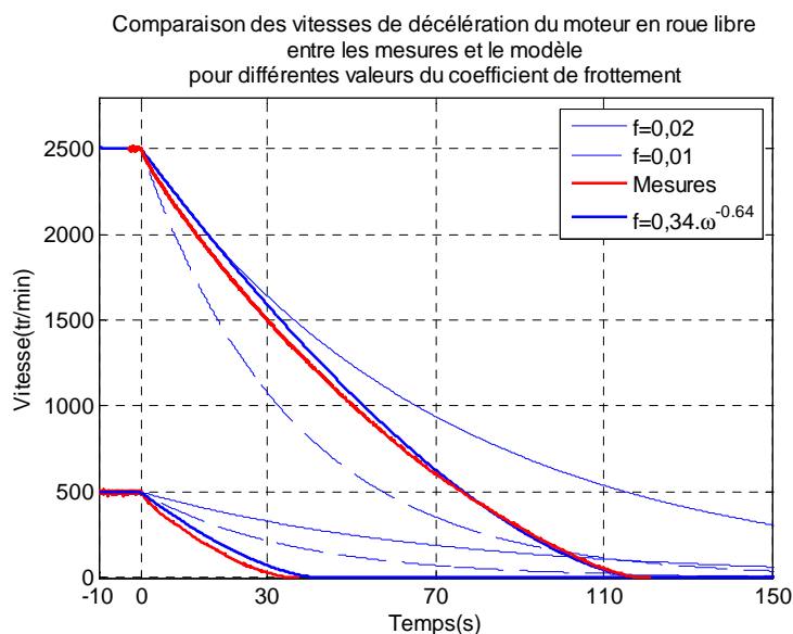
Figure 96 : simulation d’essais de lâcher en roue libre moteur seul
