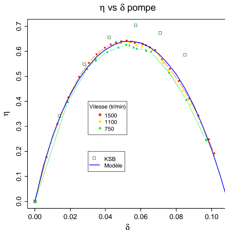
Figure 130 : rendement pompe fonction du coefficient de débit
