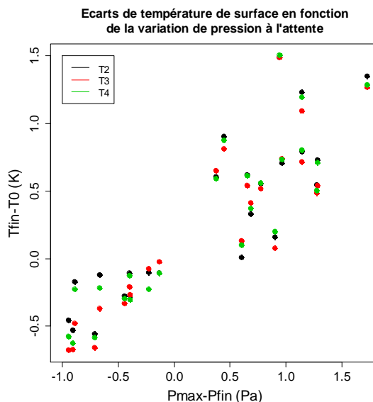
Figure 105 : Ecart entre les températures initiales et finales de paroi
