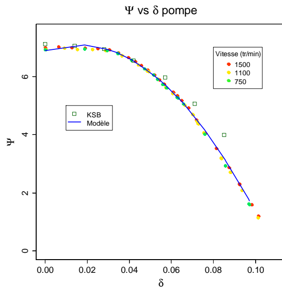
Figure 128: surpression adimensionnée fonction du coefficient de débit
