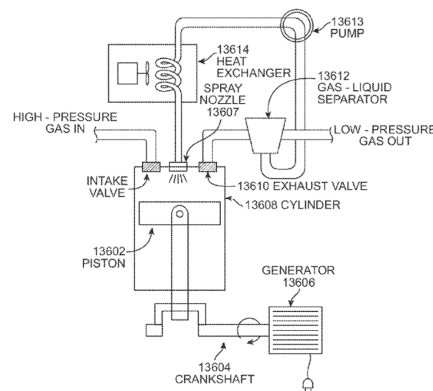
Figure 14 : LightSail Energy, système à prise directe [11]
