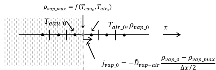
Figure 43 : indications sur le modèle pour la prise en compte de la diffusion de vapeur
