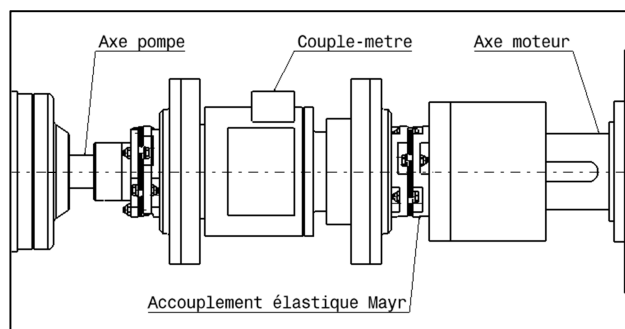
Figure 18 : accouplements et couple-mètre
