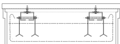
Figure 19 : schéma pour le coffrage et ferrailage de la dalle principale
