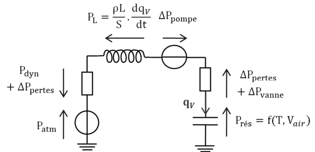
Figure 81 : analogie électrique du réseau d'eau
