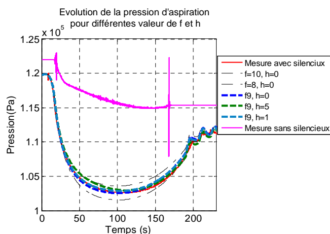
Figure 100 : pression d'aspiration
