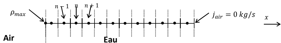
Figure 31 : illustration du problème de diffusion d'air dissous dans l'eau
