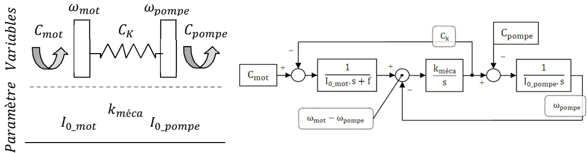
Figure 87 : structure de calcul pour ligne mécanique
