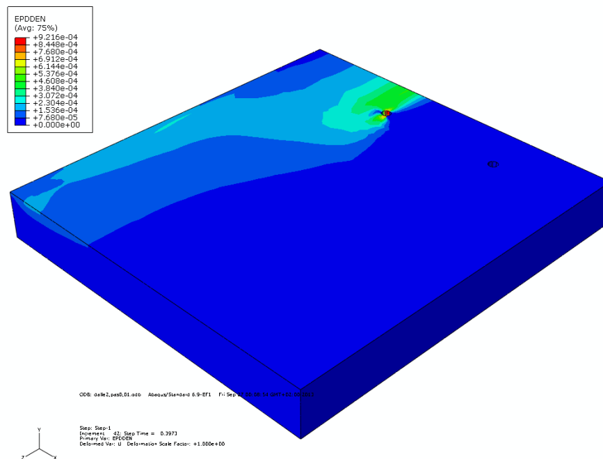
FIGURE 6.16 – Plastification (densité de déformation plastique) de la dalle 2 pour une charge égale à 6,3 kN
