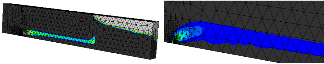
FIGURE 3.16 – Rupture par peeling-off
