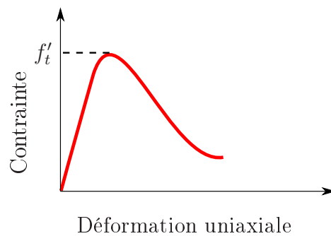
FIGURE 3.3 – Comportement du béton en traction uniaxiale
