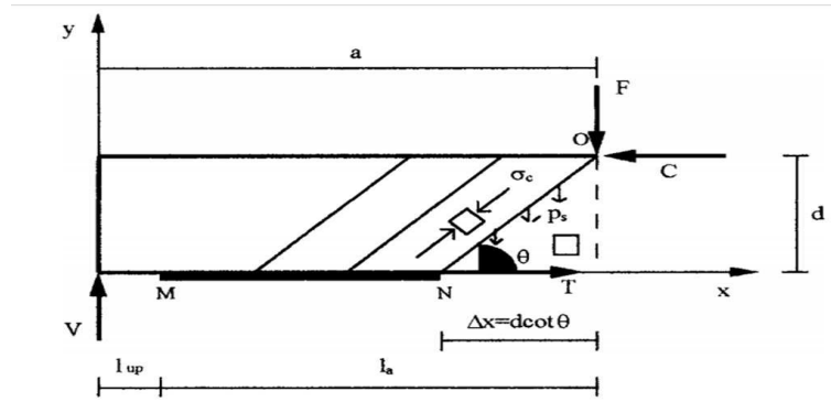
FIGURE 1.11 – Diagramme du corps libre avec la méthode des bielles et tirants
