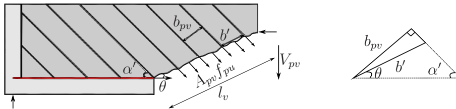
FIGURE 2.4 – Diagramme des forces mobilisées pour une fissure d'effort tranchant
