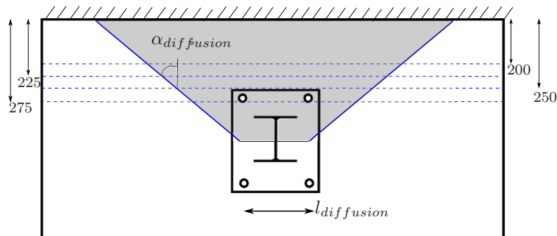
FIGURE 6.11 – Diffusion de la charge
