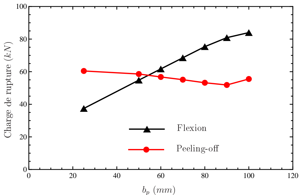
FIGURE 4.4 – Influence de la largeur de la plaque composite sur la charge de rupture
