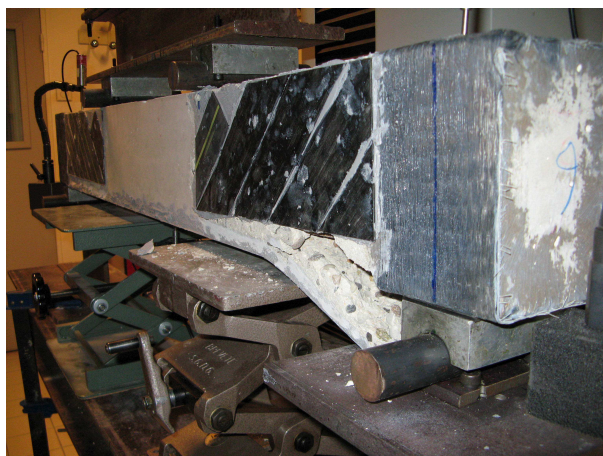
FIGURE 2.12 – Rupture de poutres renforcées par peeling-off
