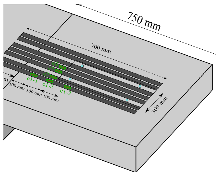
FIGURE 5.18 – Position des jauges de déformation sur les plats en PRF de la dalle 4
