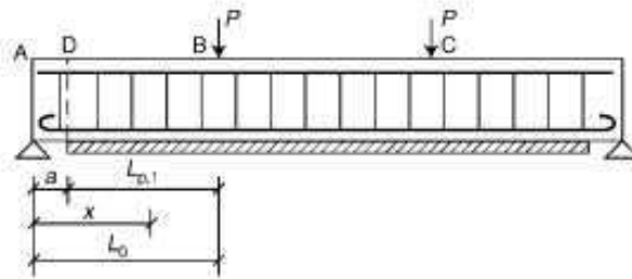
FIGURE 1.6 – Longueur du renfort dans la zone de cisaillement
