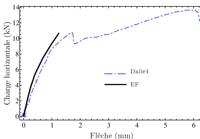
FIGURE 6.25 – Comportement global de la dalle 4
