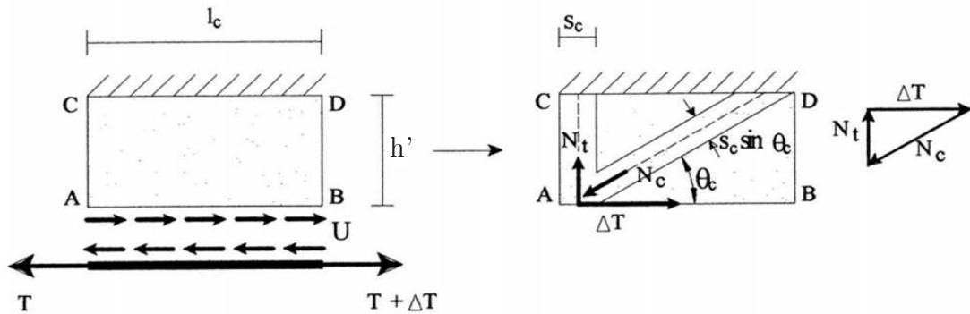
FIGURE 1.12 – Méthode des bielles et tirants pour une partie du béton d'enrobage entre deux fissures
