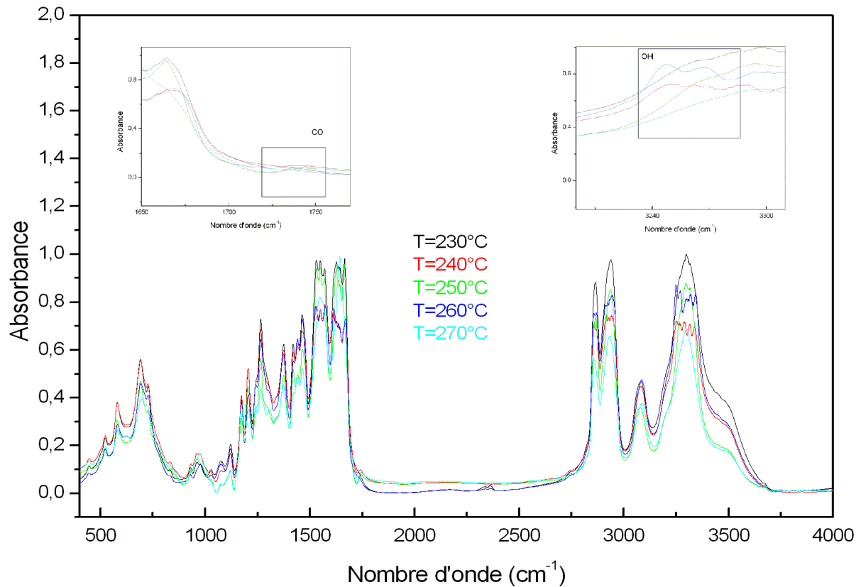
Figure VI.4 : Spectre IR du PA6 à T=230, 240, 250, 260 et 270°C pour t=20 min
