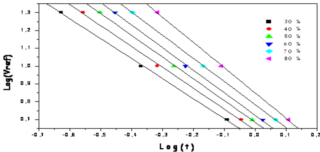
Figure IV.20: Variation de \log(V_{ref}) en fonction de \log(t) du PA6.
