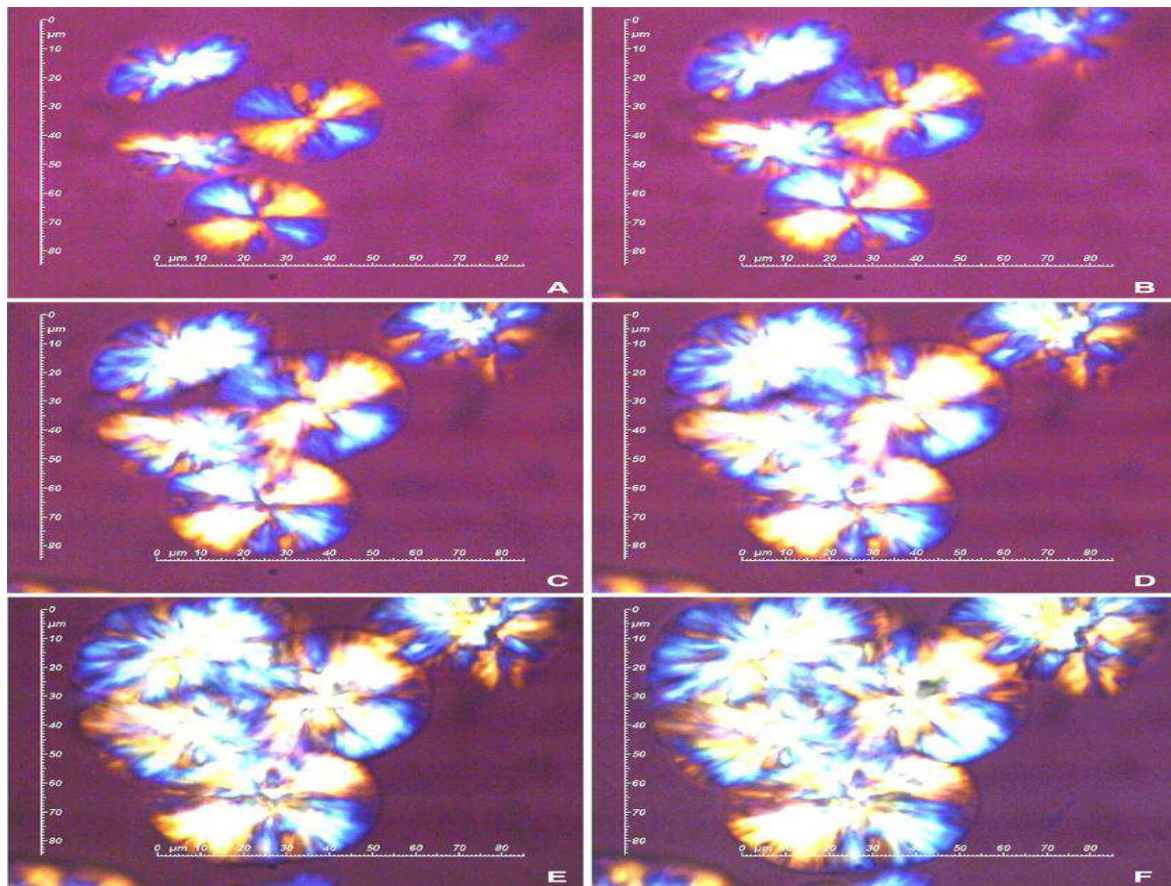
Figure IV.11: visualisation des sphérolites durant la cristallisation du PA 12 à la température de 168°C et à différents temps de maintien. (a) 120min, (b) 130min, (c) 140min, (d) 150min, (e) 160min, (f) 170min
