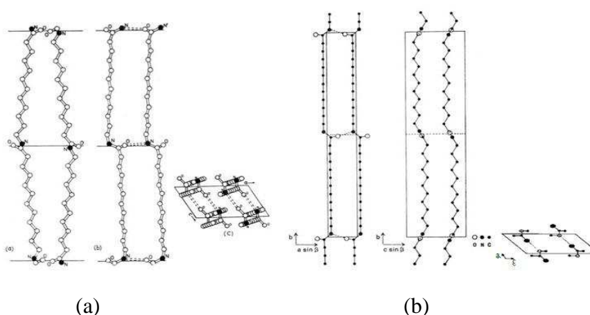
Figure I.4 : Structures cristallines du PA12. (a) Modèle de Inoue et Hoshino [7], (b) Modèle de Cojazzi et al. [15].
