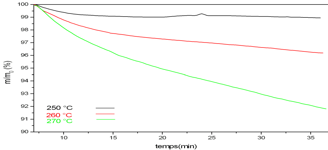
Figure VI.2 : Variation de la fraction massique restante pendant le vieillissement thermique de poudre de PA6 exposé à 250, 260 et 270°C (isotherme).
