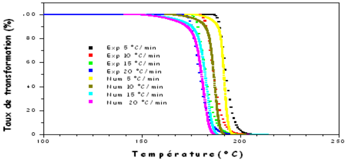
Figure IV.14 : Evolution du taux de transformation de la cristallinité relative du PA6.
