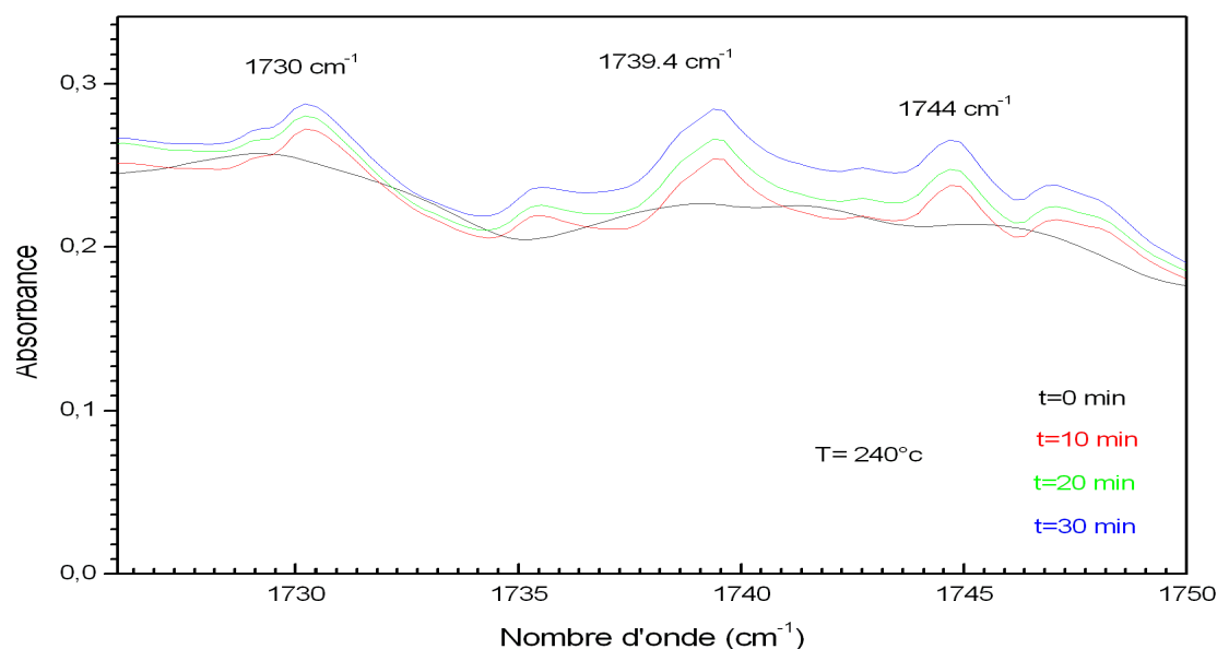
Figure VI.7 : Spectre IR représentant l'évolution des pics de C=O à T=240^{\circ}\text{C} et t=0, 10, 20 et 30\text{ min} .
