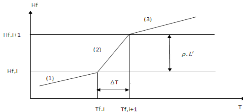
Figure V.3: Loi d'évolution de l'enthalpie de fusion en fonction de la température. [70]
