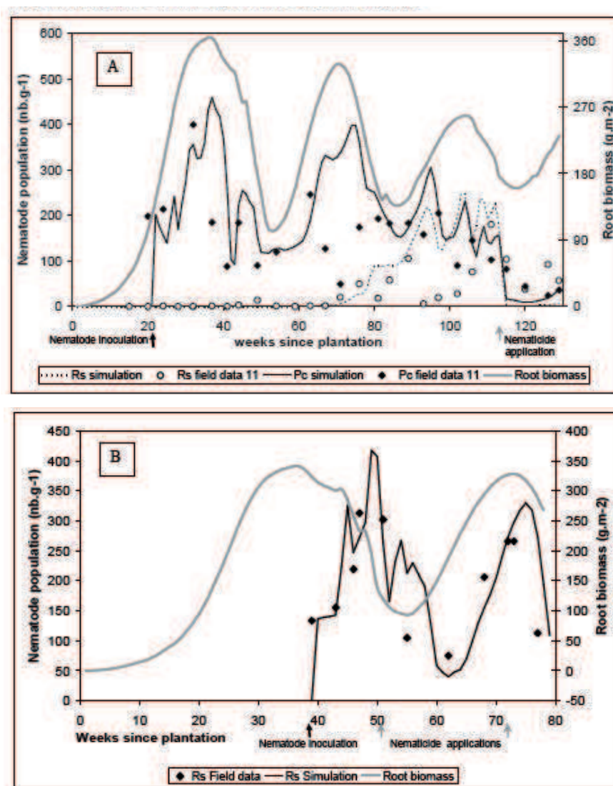
Figure 3 Variations au cours du temps des densités mesurées (field data) et simulées (simulation) des espèces Radopholus similis (Rs) et Pratylenchus coffeae (Pc) dans les racines (nombre/g) et de la biomasse racinaire (Root biomass) (en g/m 2 ) simulées par le model SIMBA pour deux stratégies de gestion des nématodes phytoparasites : (A) monoculture avec pesticides, (B) plantations de bananiers après canne à sucre avec de faible apport en pesticides (extrait de Tixier et al., 2006).
