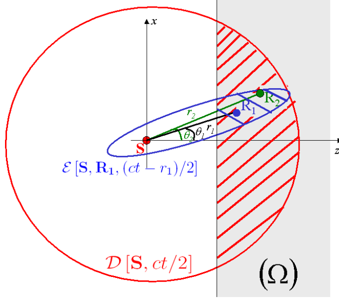
FIG. IV.8: Différentes notations utilisées pour le calcul de l'intensité multiple diffusée I^M(X = 0, t)
