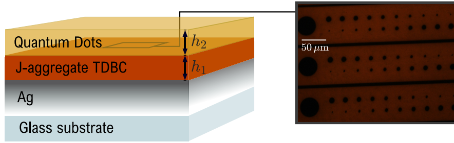
Figure C.4 – Schéma d'un échantillon multicouche constitué de deux films minces fluorescents déposés sur une couche de 50 nm d'argent évaporé sur un substrat en verre. La première couche déposée, d'épaisseur h_1 , contient l'agrégat J TDBC. L'image de microscopie en champ sombre montre la lithographie optique réalisée sur cette couche, dans laquelle l'exposition à un laser UV a photo-blanchi les zones sombres circulaires. Ensuite, une deuxième couche d'épaisseur h_2 contenant des boîtes quantiques est déposée.
